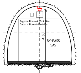
SEZIONE A-A 1:100 COUPE A-A 1:100
