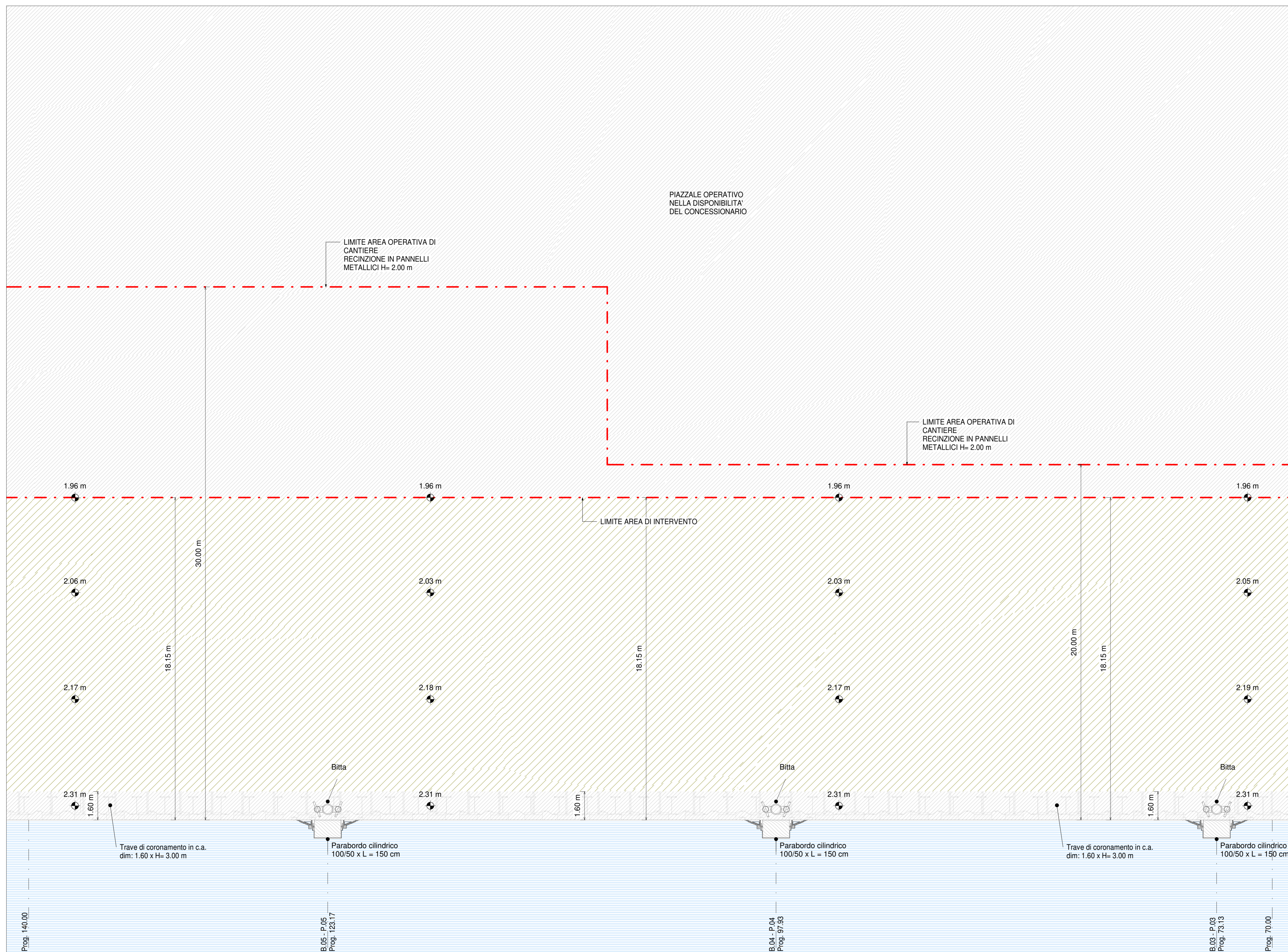
Pianta generale delle demolizioni e degli scavi - Inq. 2 1 : 100
