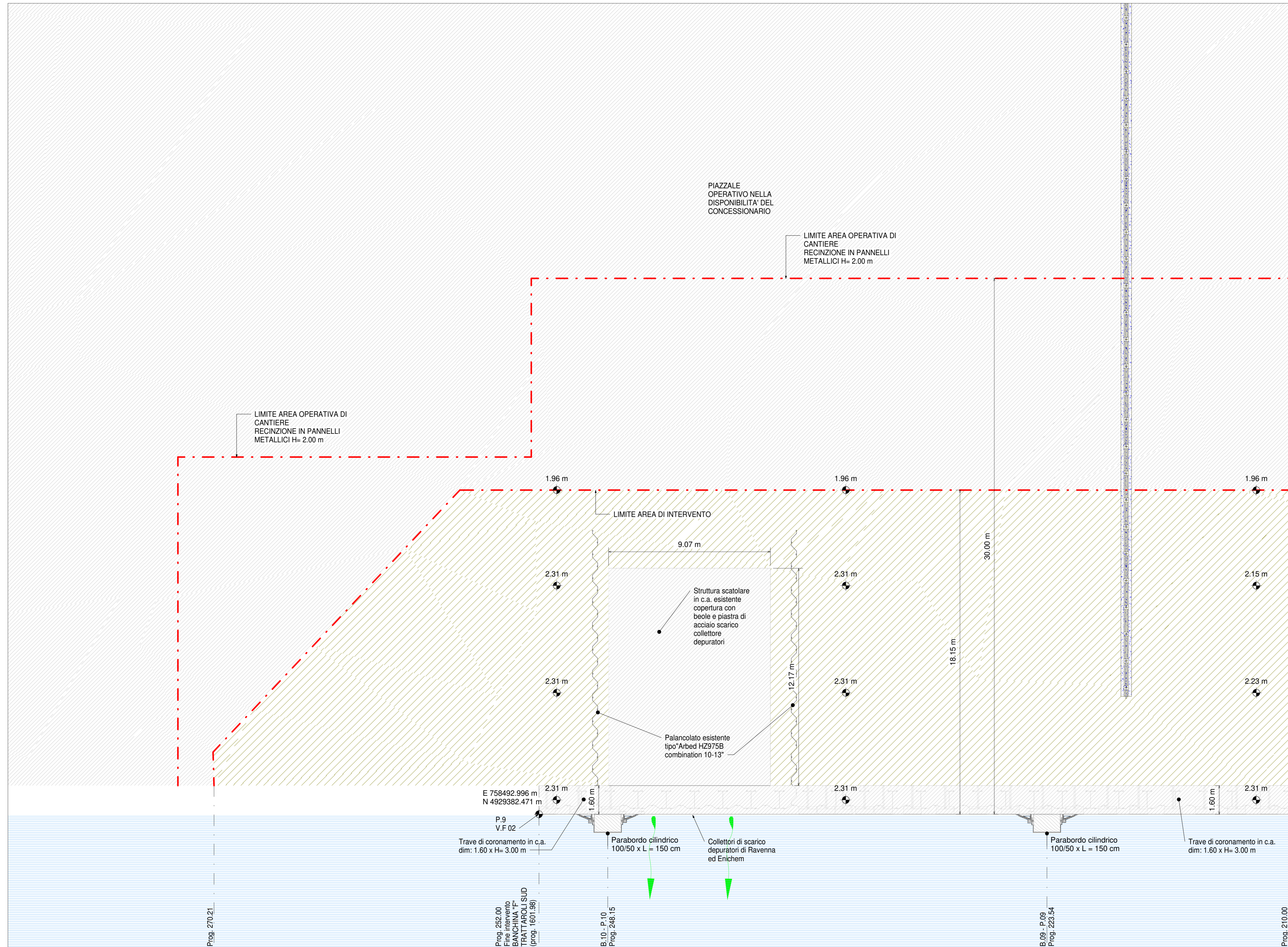
Pianta generale delle demolizioni e degli scavi - Inq. 4
