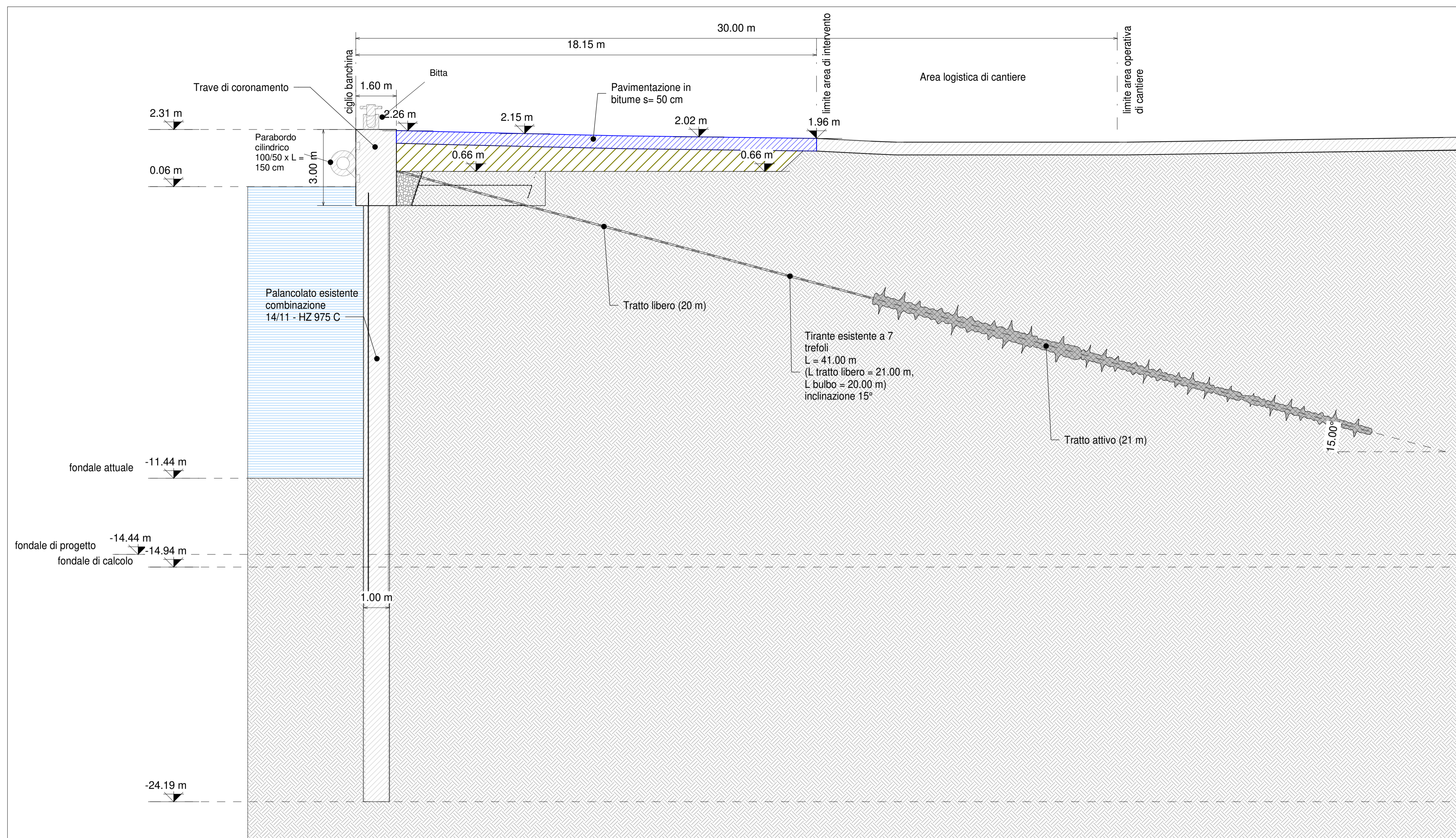
Sezione A-A - demolizioni 1 : 100
