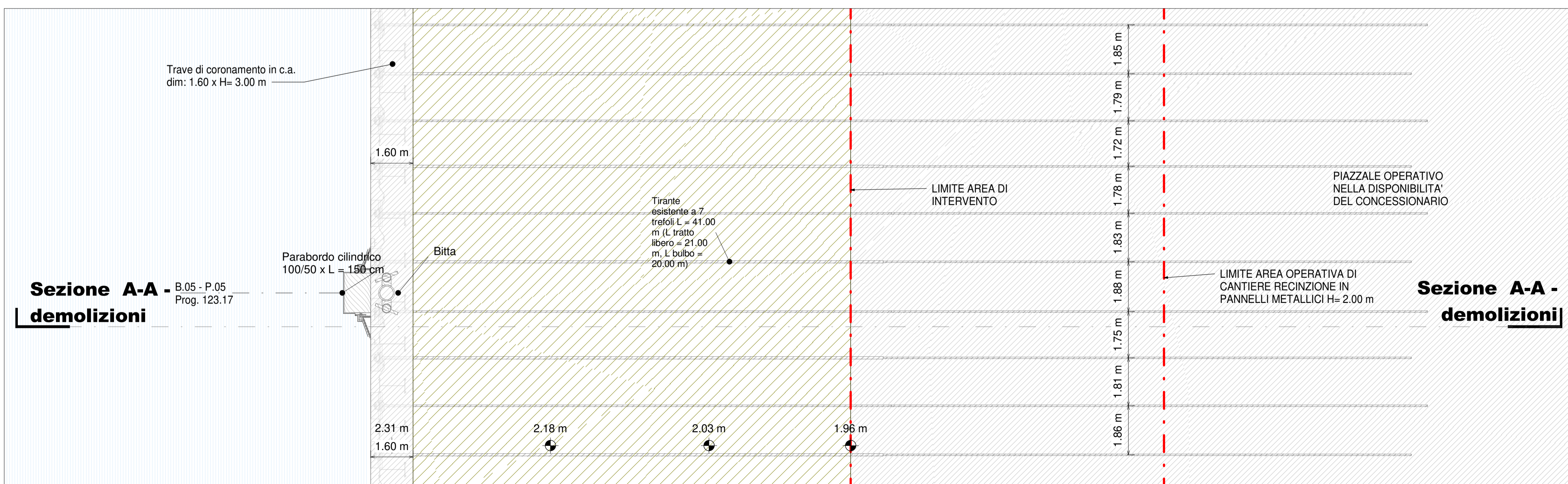
Pianta degli scavi e delle demolizioni ubicazione sezione 1 : 100
