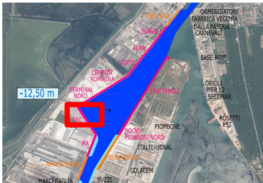
Figura 1 – Planimetria relativa alle banchine da adeguare con individuazione della banchina TRATTAROLI SUD (G)
