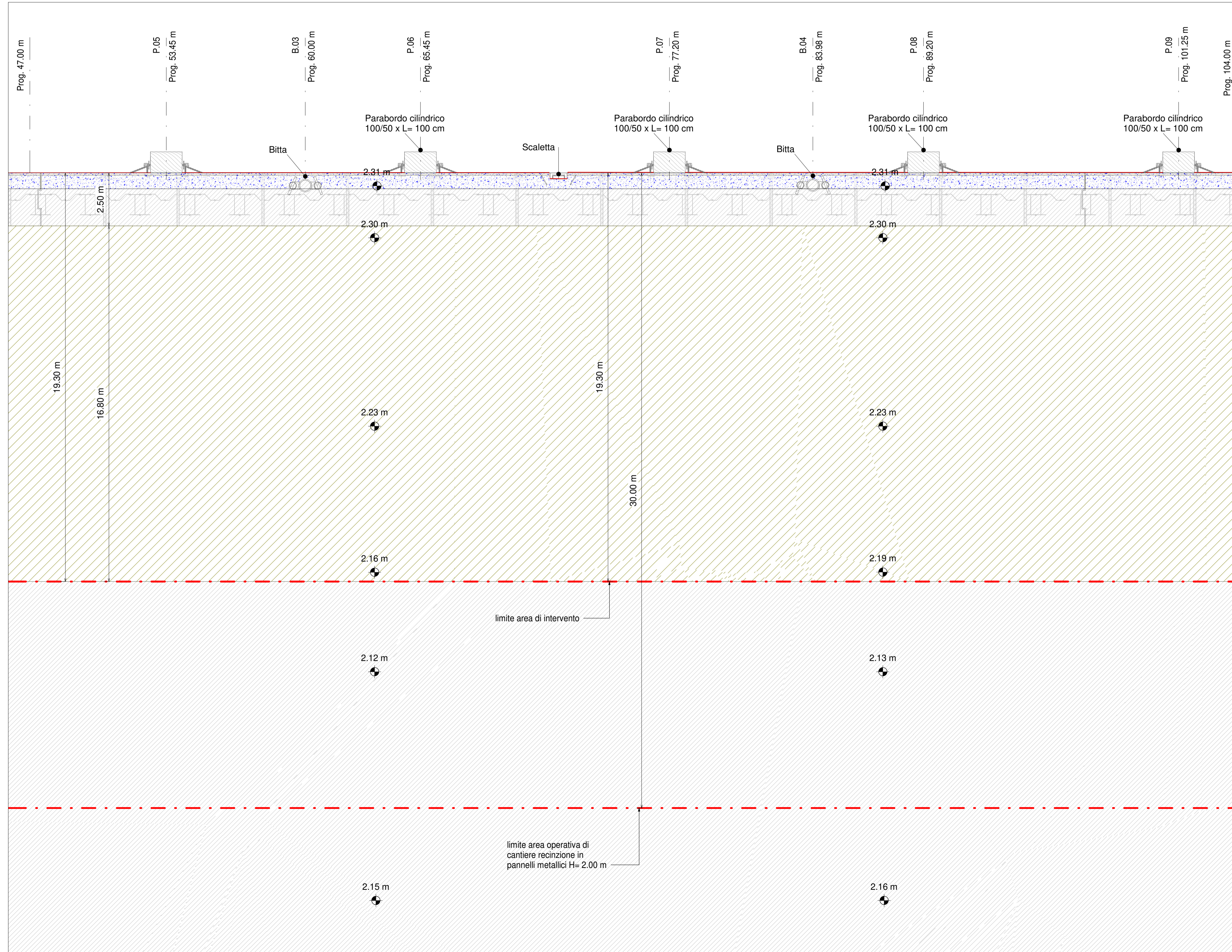
Pianta generale delle demolizioni e degli scavi - Inq. 2
