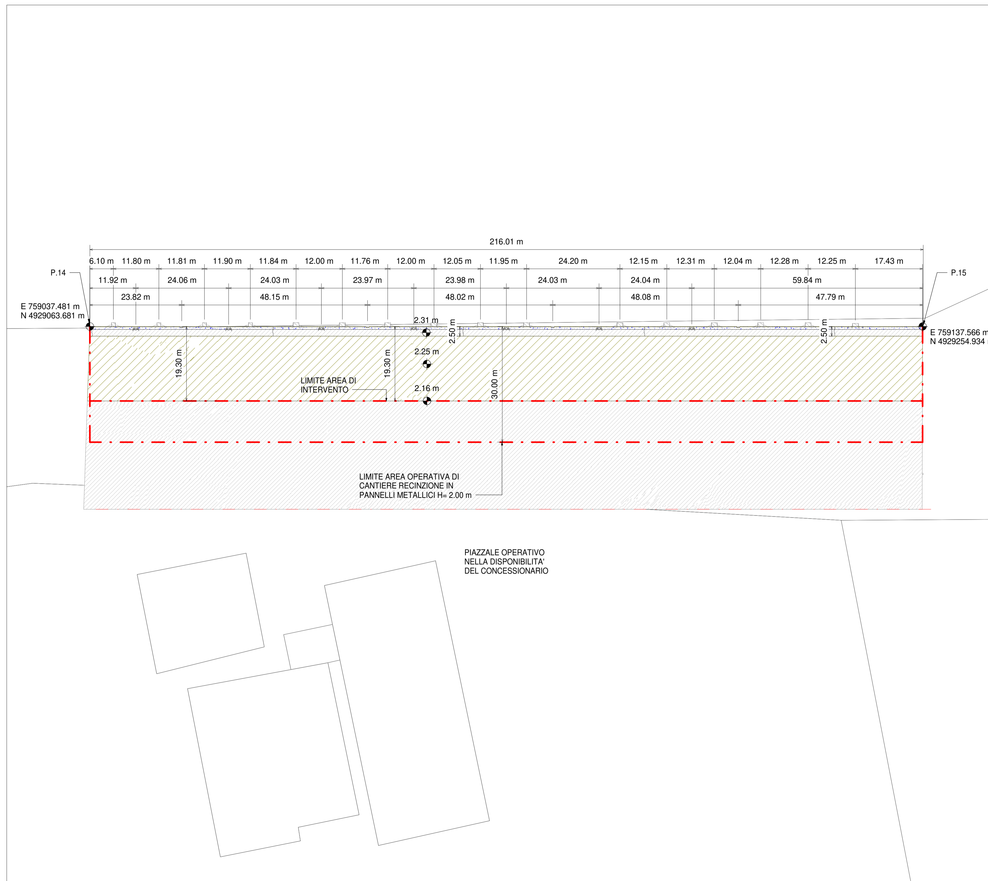
Planimetria generale delle demolizioni e degli scavi 1 : 500
