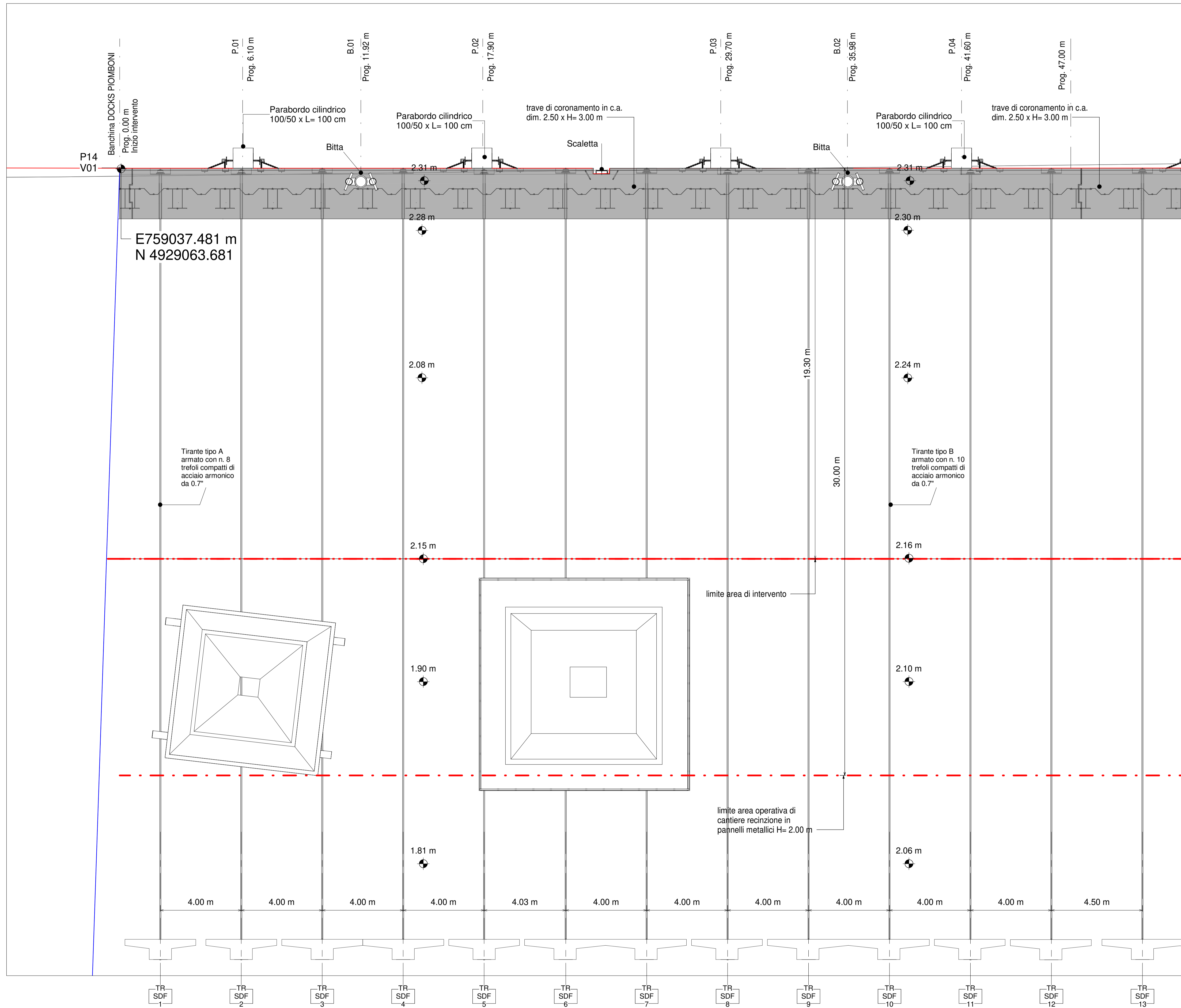
Pianta SDF - Inq. 1 1 : 100
