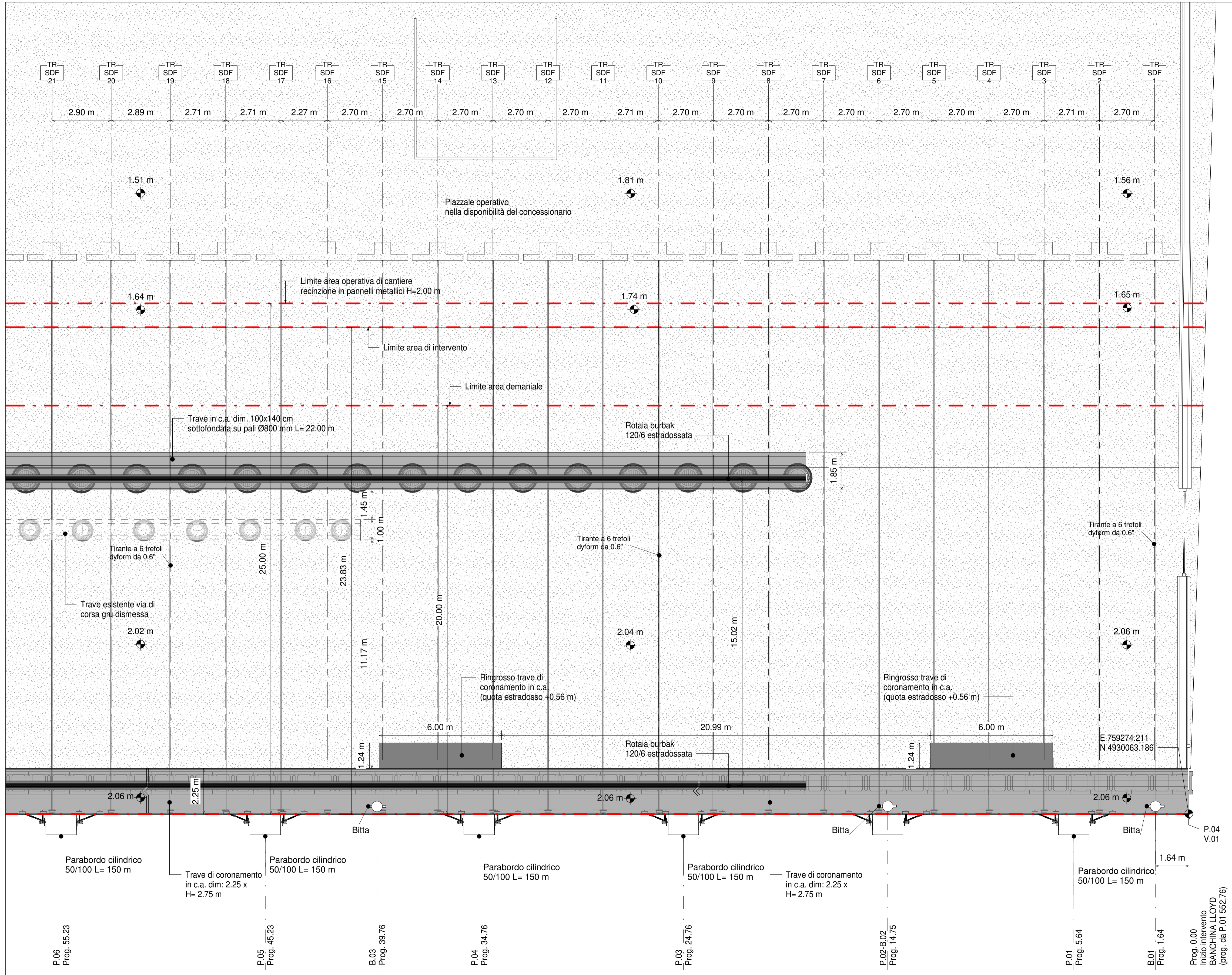
Pianta SDF - Inq.1 1 : 100
