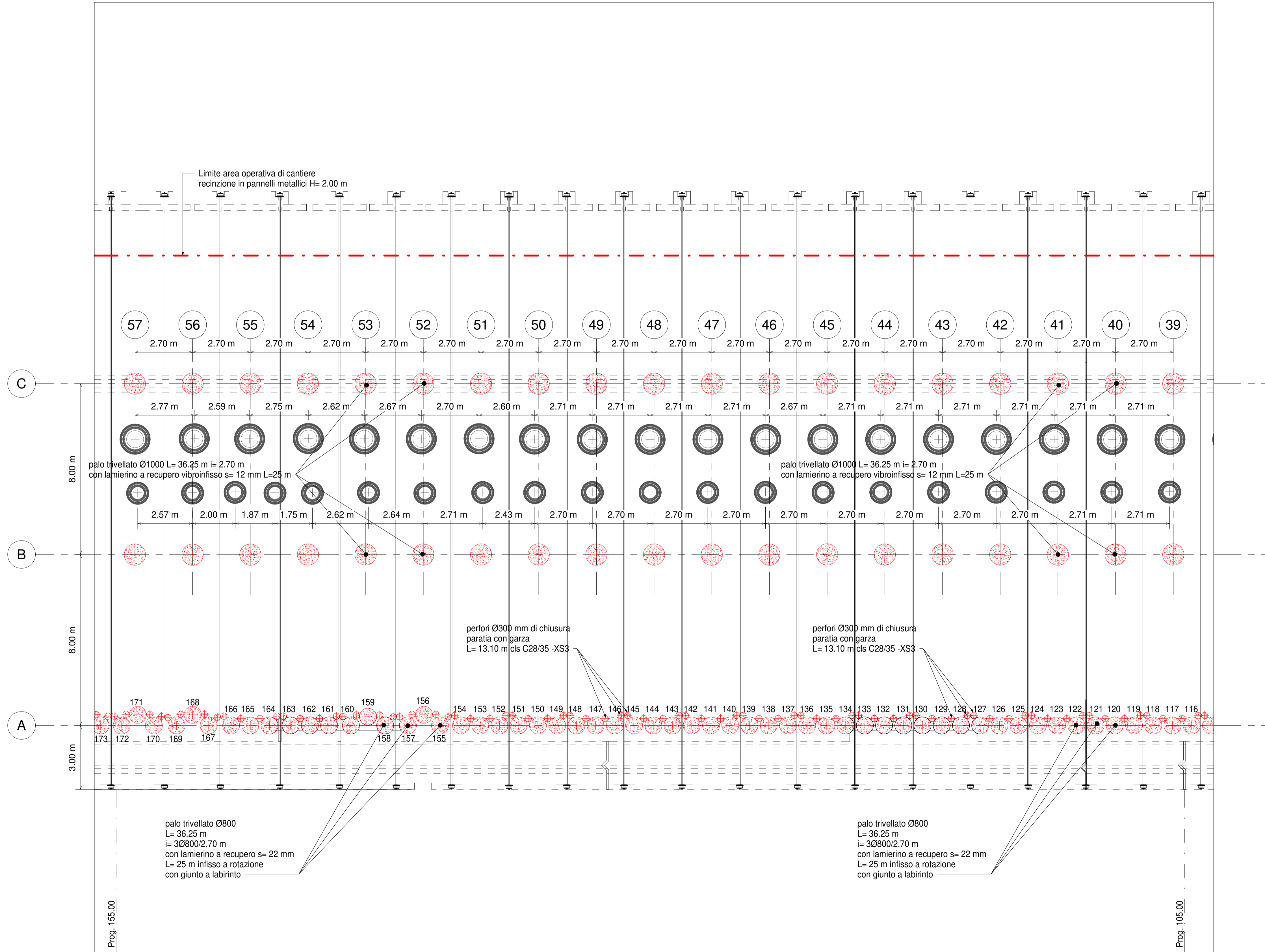
Pianta tracciamento pali - Inq.3
