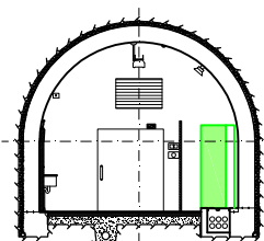
SEZIONE B-B 1:100 COUPE B-B 1:100
