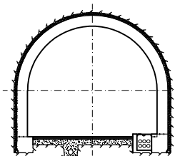
SEZIONE C-C 1:100 COUPE C-C 1:100
