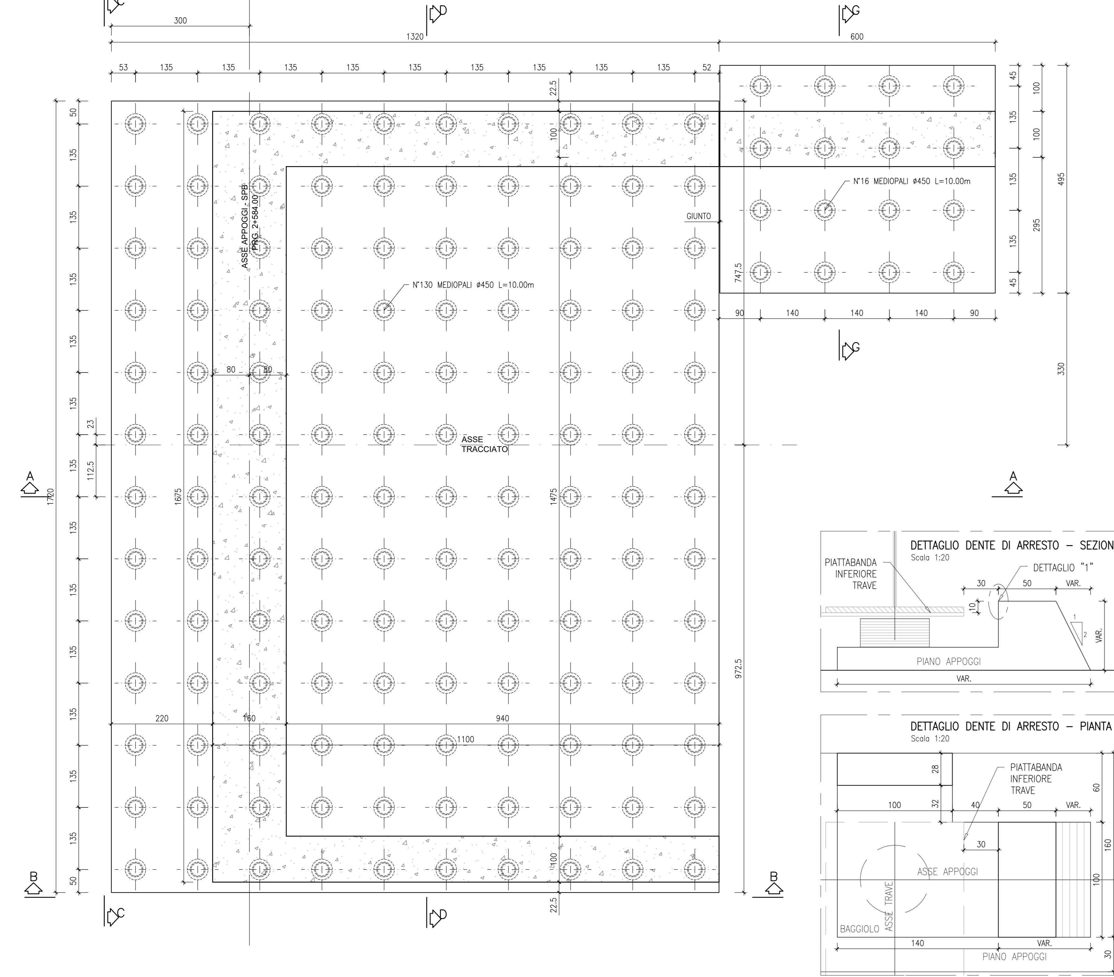
SEZIONE E-E SCALA 1:50
