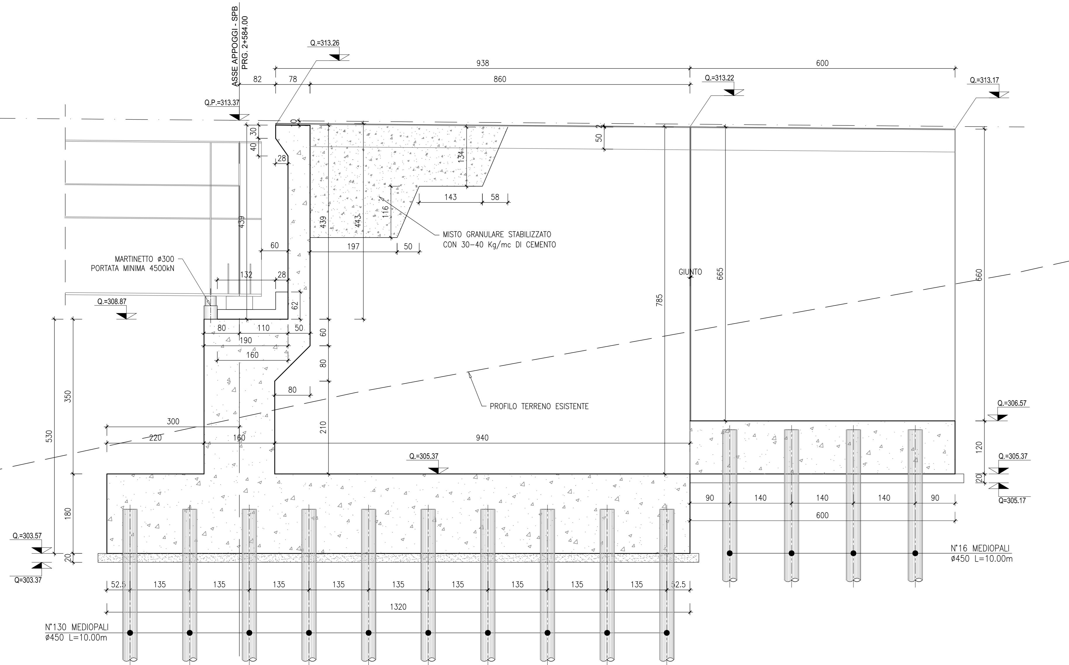
SEZIONE A-A SCALA 1:50
