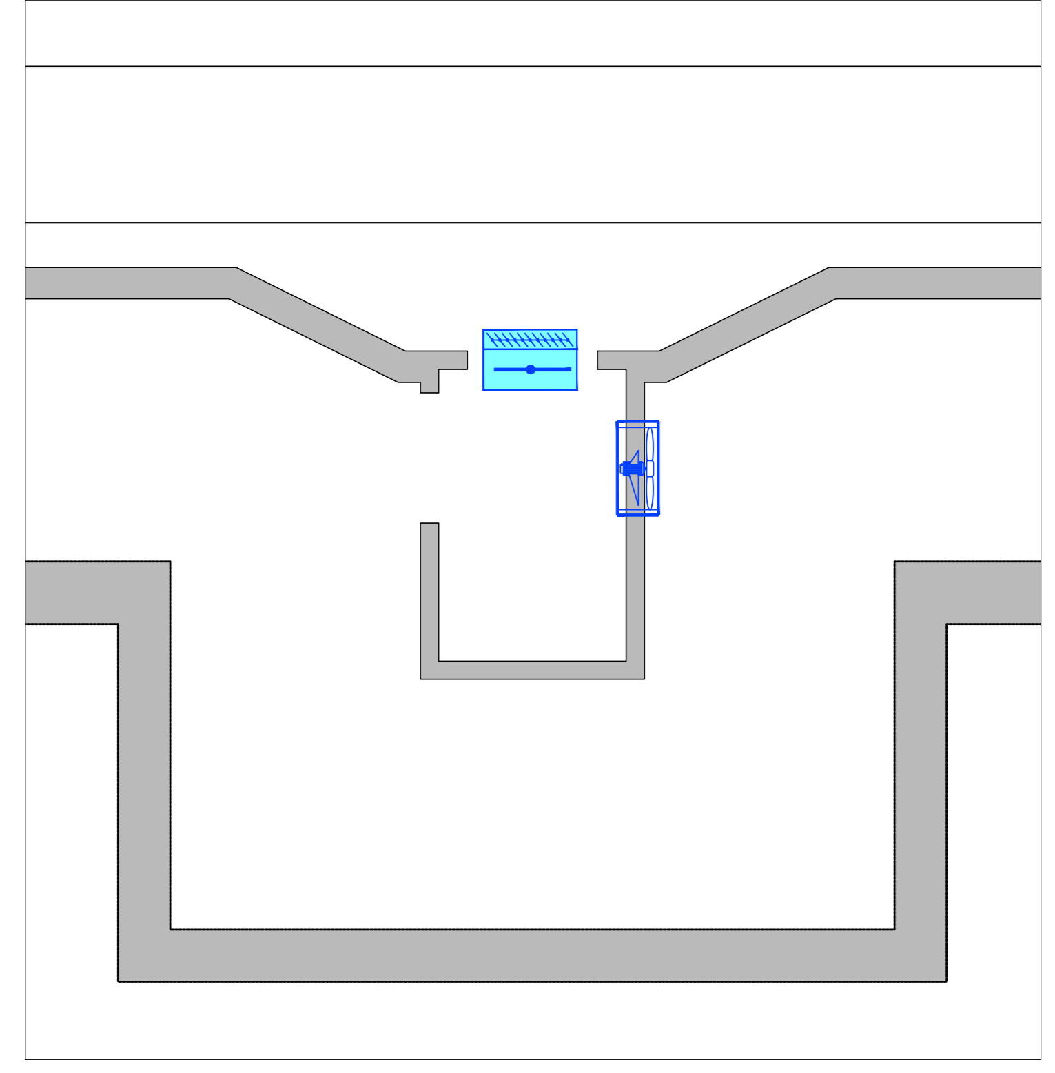
PLANIMETRIA LUOGO SICURO - SCALA 1:50
