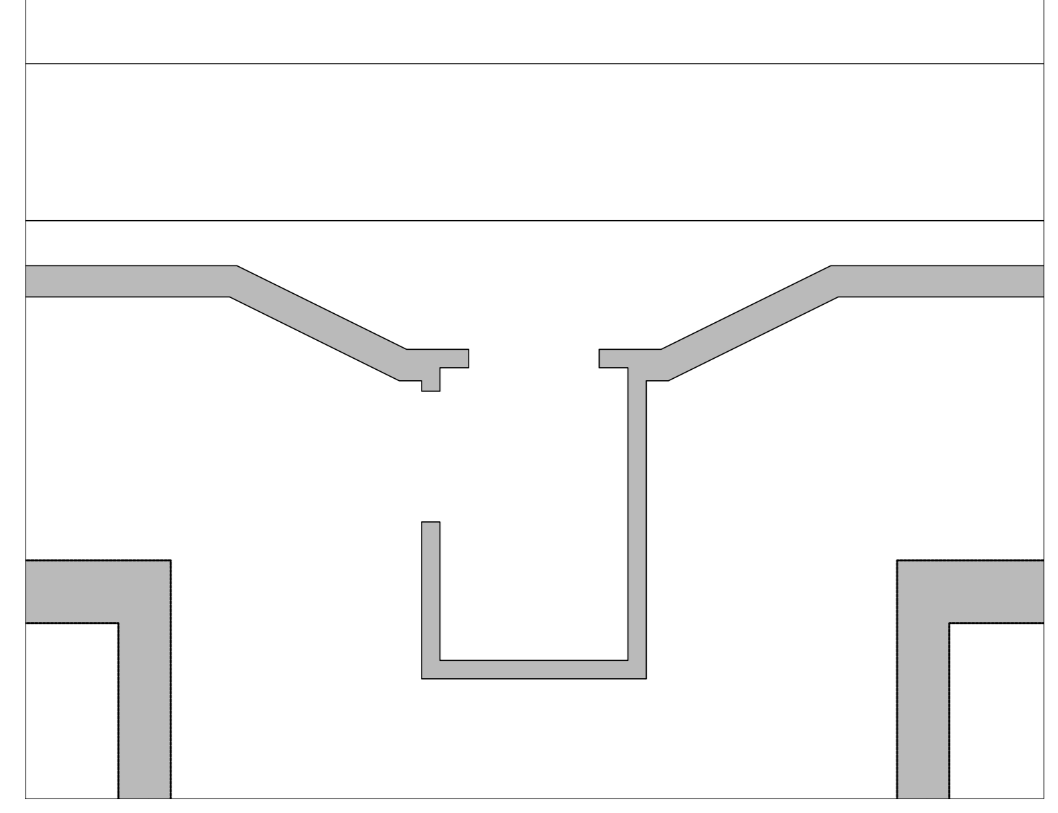
PLANIMETRIA LUOGO SICURO - SCALA 1:50
