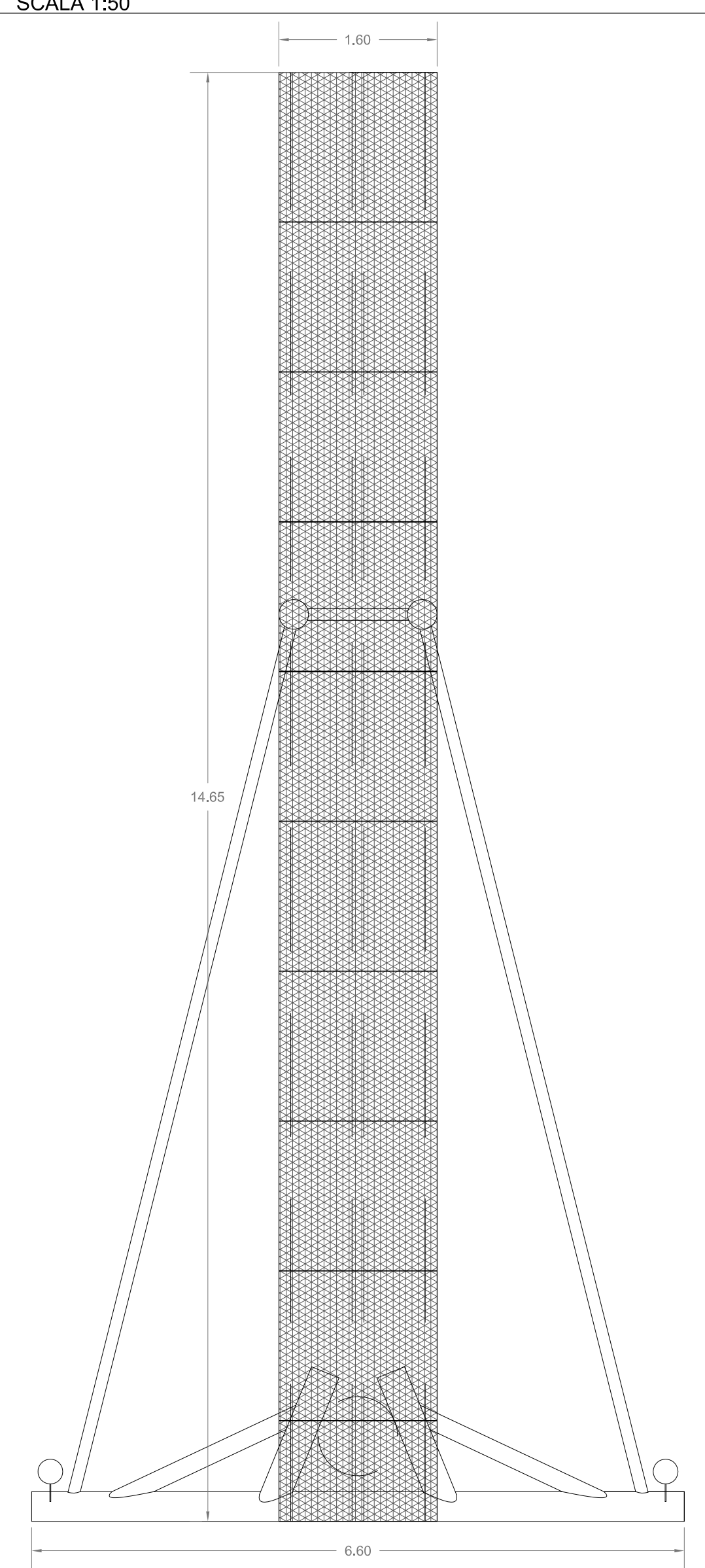
PARTICOLARE C PIANTA - pontiletto per carico e scarico prodotti infustati SCALA 1:50
