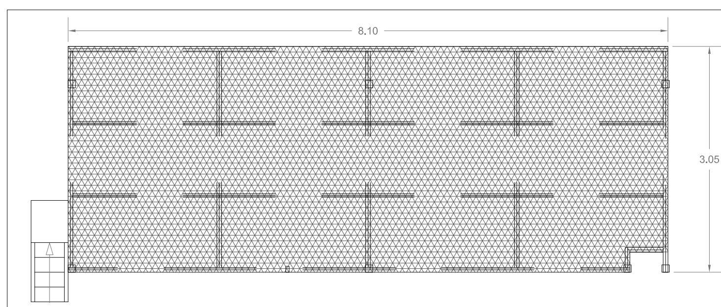
PARTICOLARE B PIANTA - piano di appoggio per prodotti infustati SCALA 1:50
