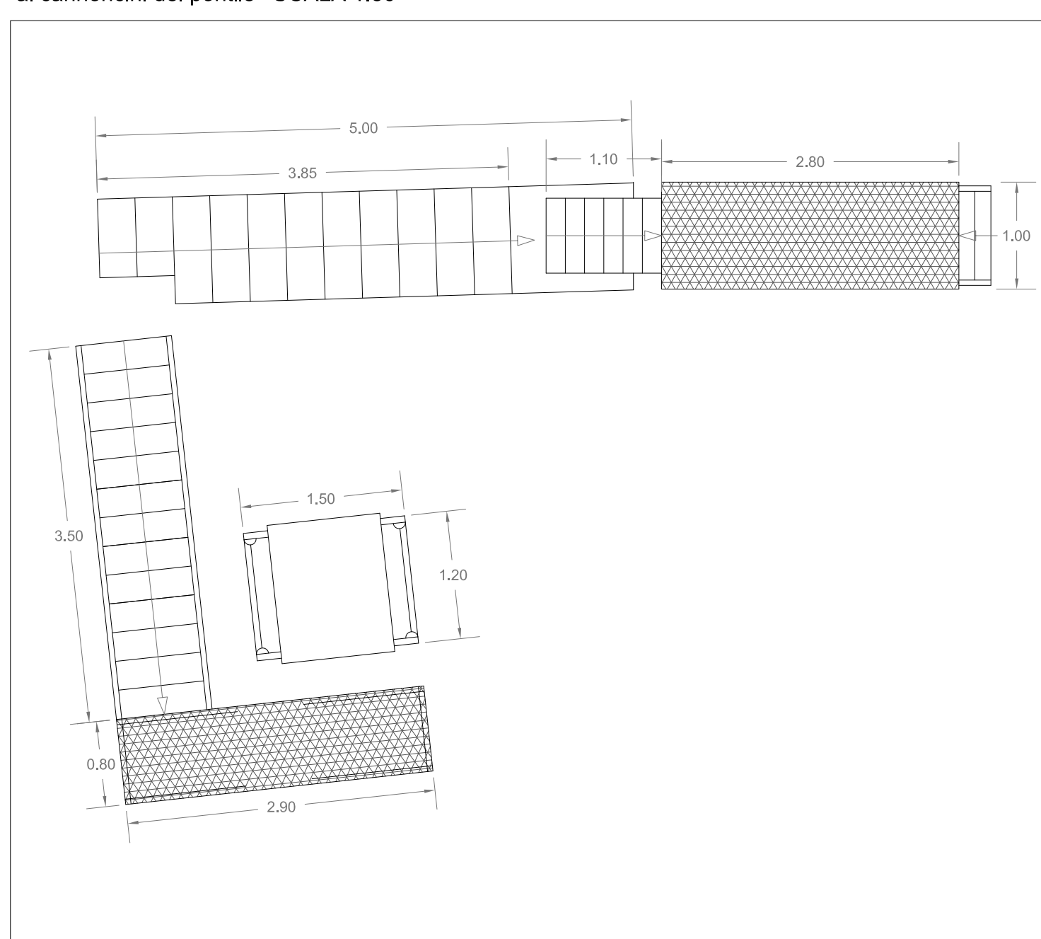
PARTICOLARE B PIANTA - piano di appoggio per prodotti infustati SCALA 1:50
