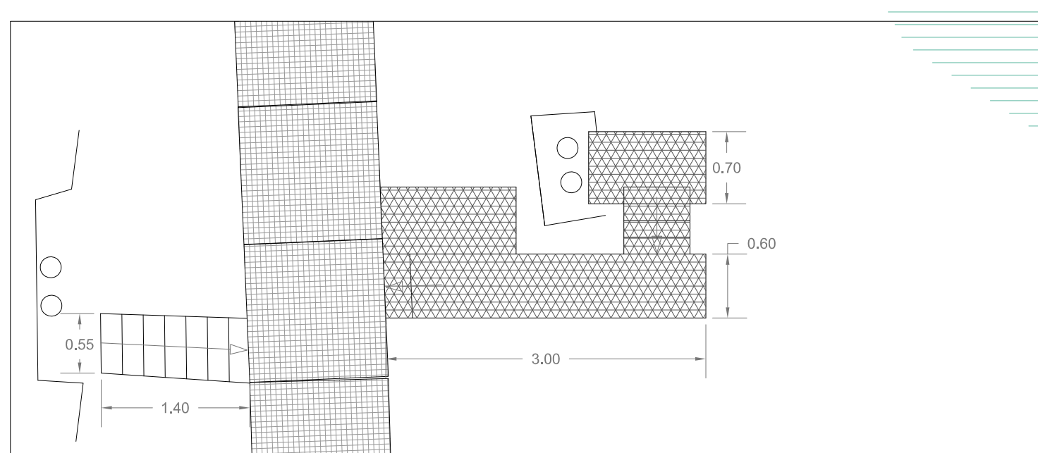
PARTICOLARE A PIANTA - accessi bitte a terra SCALA 1:50
