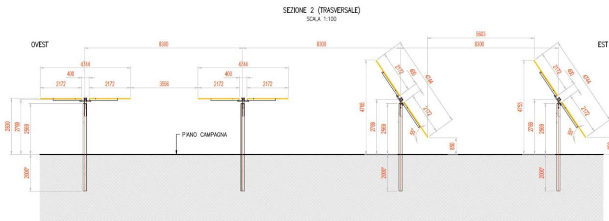
Particolare strutture sostegno moduli e distanze di campo
