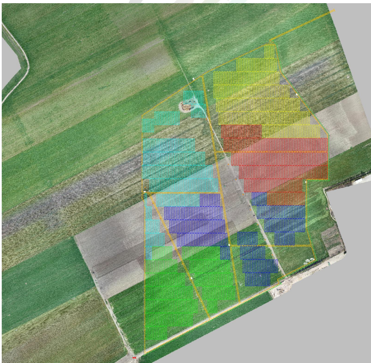
Figura 2-1: Layout d'impianto su Ortofoto
