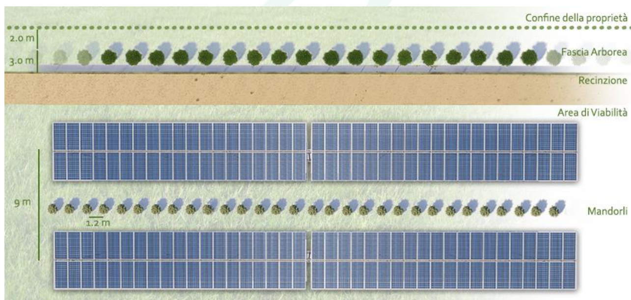
Figura 2-2: Soluzione Agro-Solare: barriera verde perimetrale, viabilità interna, tracker e componente agronomica: Mandorleto Intensivo
