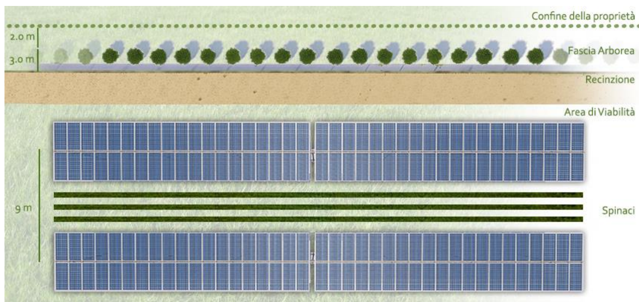
Figura 2-2: Soluzione Agro-Solare: barriera verde perimetrale, viabilità interna, tracker e componente agronomica: Spinacio da Industria
