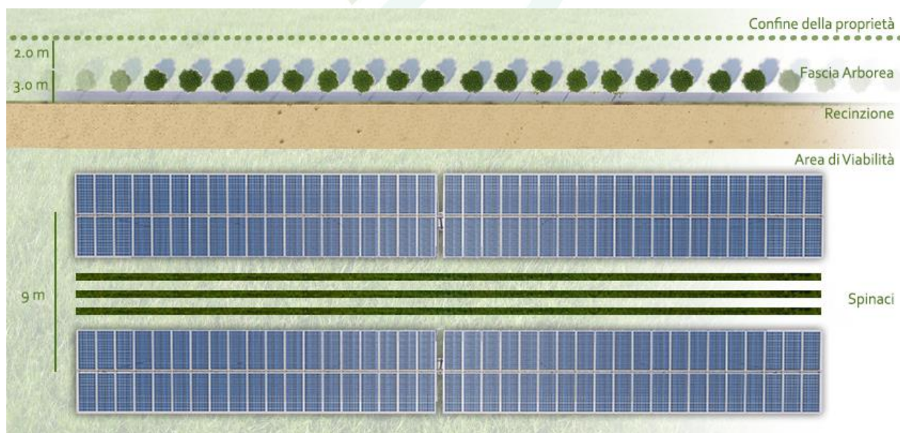
Schema impianto agri-voltaico: Spinacio da Industria
