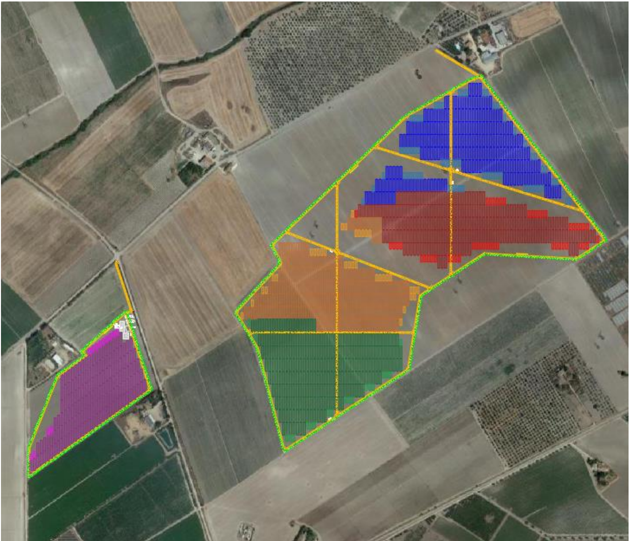
Layout impianto agri-voltaico
