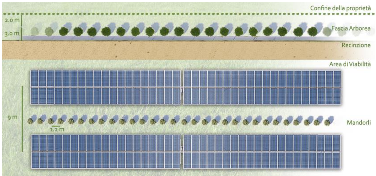
Schema impianto agri-voltaico: Mandorleto Intensivo
