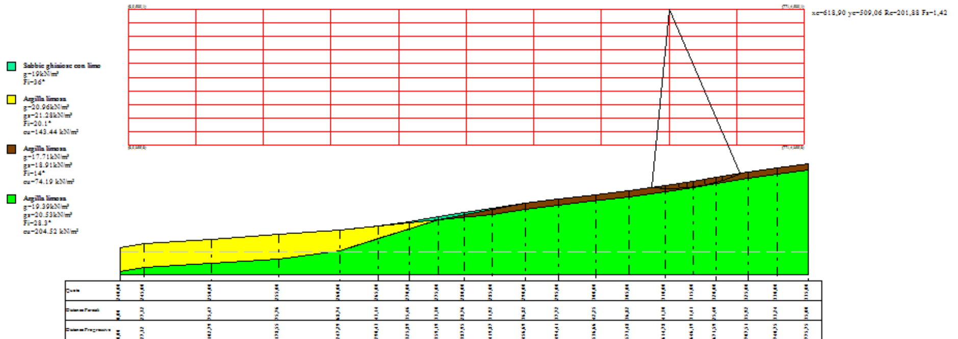
PESPA06 - Verifica di stabilità ante operam in condizioni drenate
