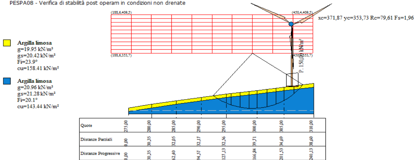
PESPA08 - Verifica di stabilità post operam in condizioni non drenate
