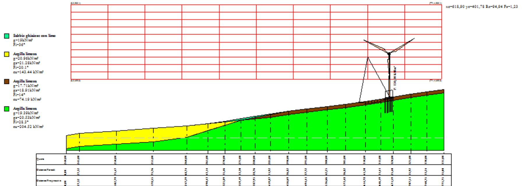
PESPA06 - Verifica di stabilità post operam in condizioni drenate
