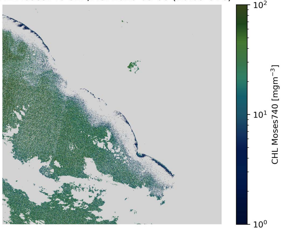
CHL Moses740 S2A/MSI 2020-03-06 (10:09 UTC)
