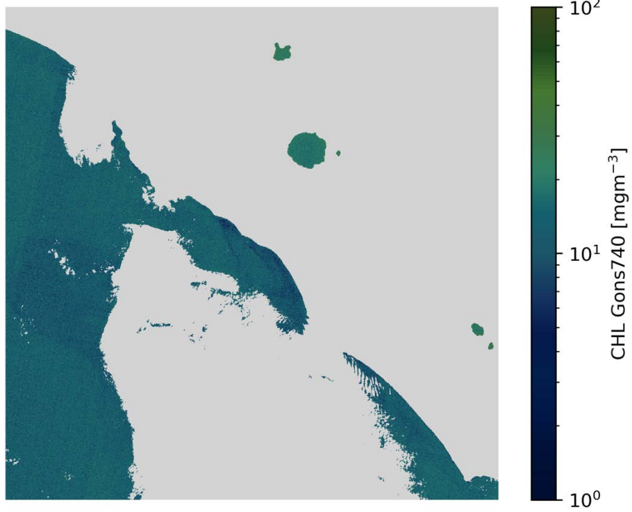
CHL Gons740 S2A/MSI 2020-11-11 (10:09 UTC)
