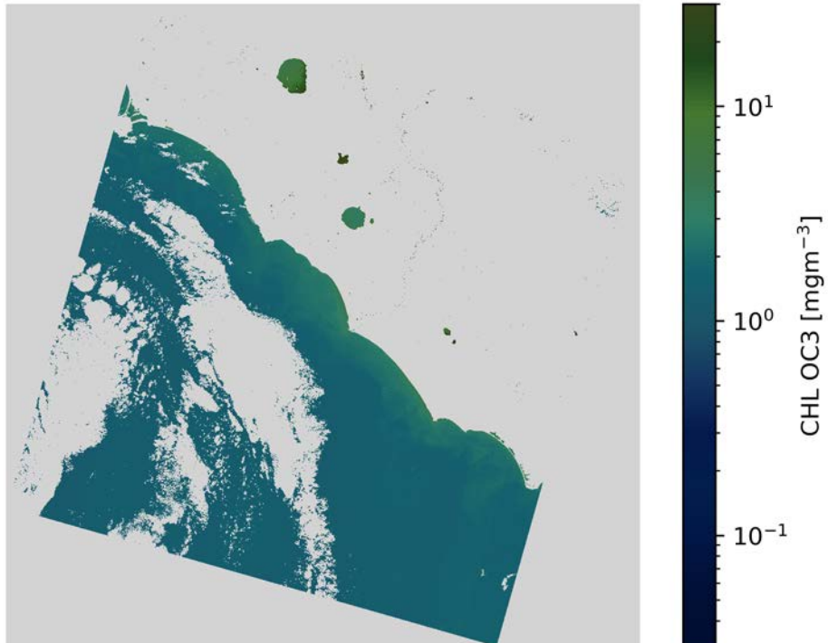
CHL OC3 L8/OLI 2020-02-21 (09:53 UTC)
