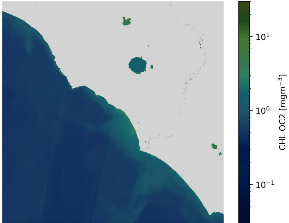
CHL OC2 S2B/MSI 2020-04-10 (10:09 UTC)
