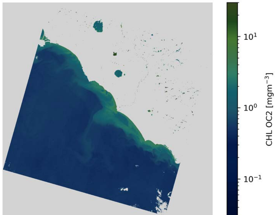
CHL OC2 L8/OLI 2020-03-08 (09:53 UTC)
