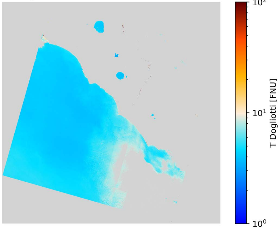
T Dogliotti L8/OLI 2020-07-30 (09:53 UTC)
