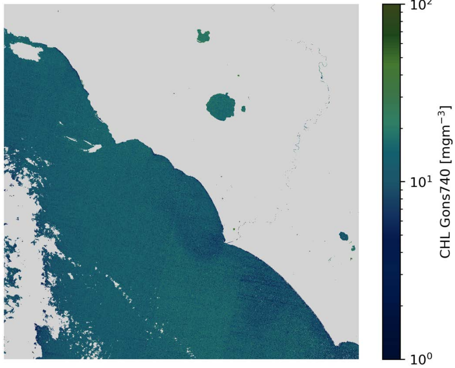
CHL Gons740 S2B/MSI 2020-09-07 (10:09 UTC)
