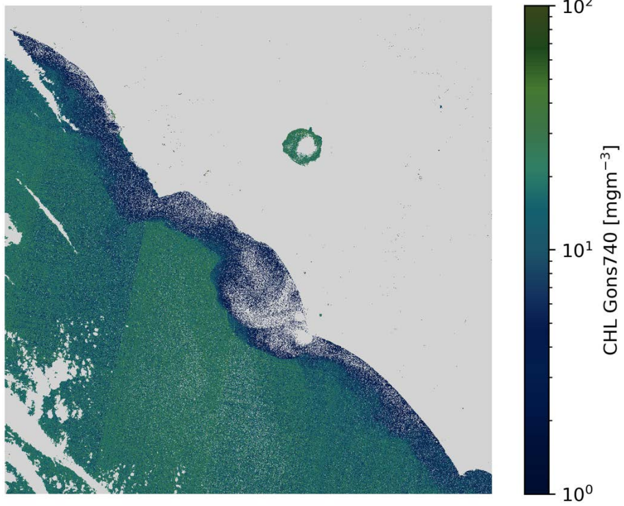
CHL Gons740 S2A/MSI 2020-12-11 (10:09 UTC)
