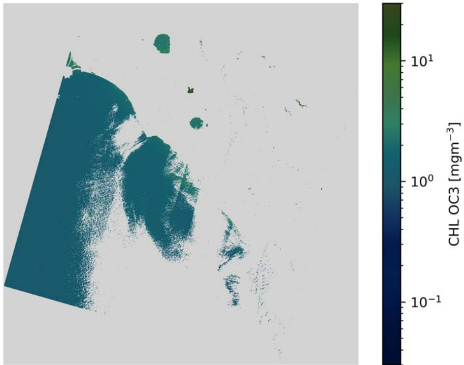
CHL OC3 L8/OLI 2020-07-14 (09:53 UTC)
