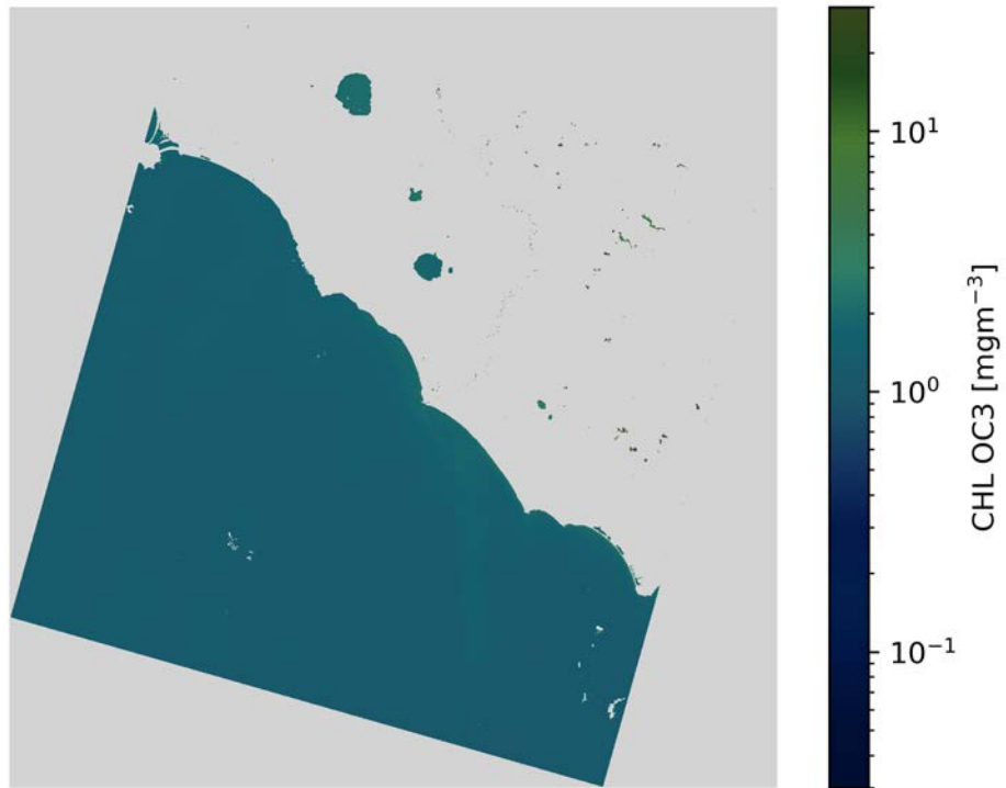
CHL OC3 L8/OLI 2020-09-16 (09:53 UTC)
