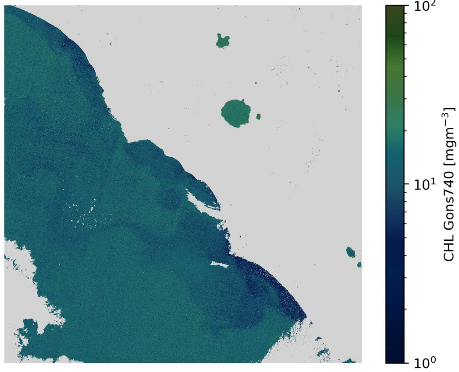
CHL Gons740 S2A/MSI 2020-11-01 (10:09 UTC)
