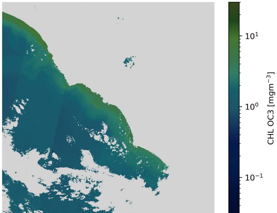
CHL OC3 S2A/MSI 2020-03-06 (10:09 UTC)
