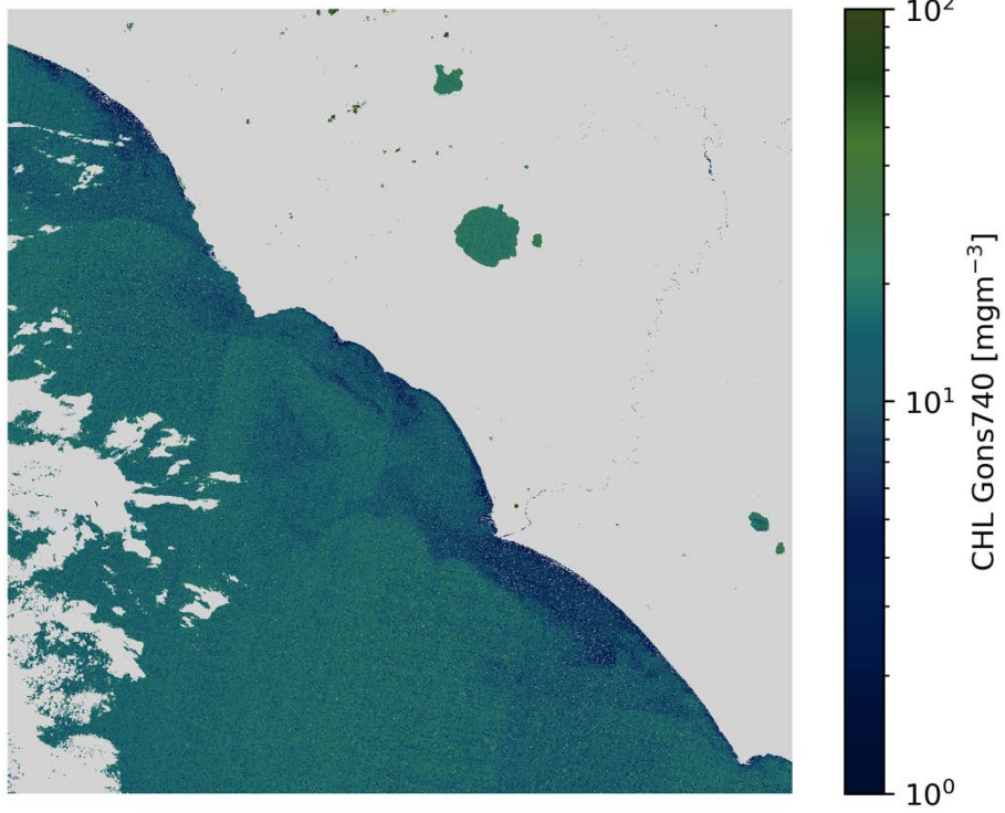
CHL Gons740 S2A/MSI 2020-10-22 (10:09 UTC)
