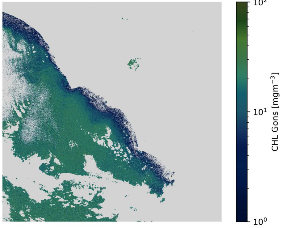
CHL Gons S2A/MSI 2020-03-06 (10:09 UTC)
