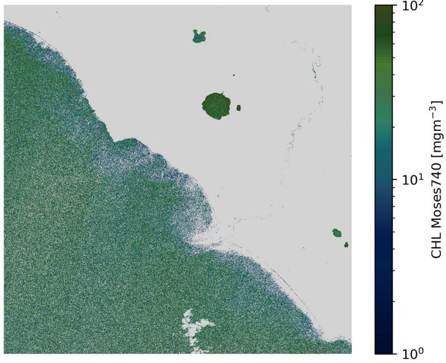
CHL Moses740 S2A/MSI 2020-04-15 (10:09 UTC)
