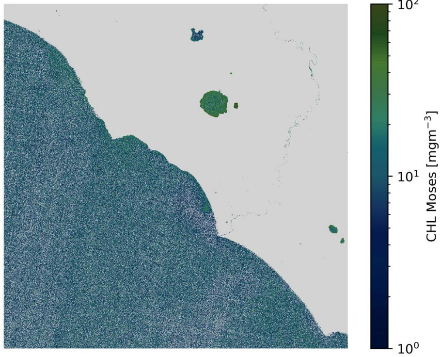
CHL Moses S2B/MSI 2020-04-10 (10:09 UTC)
