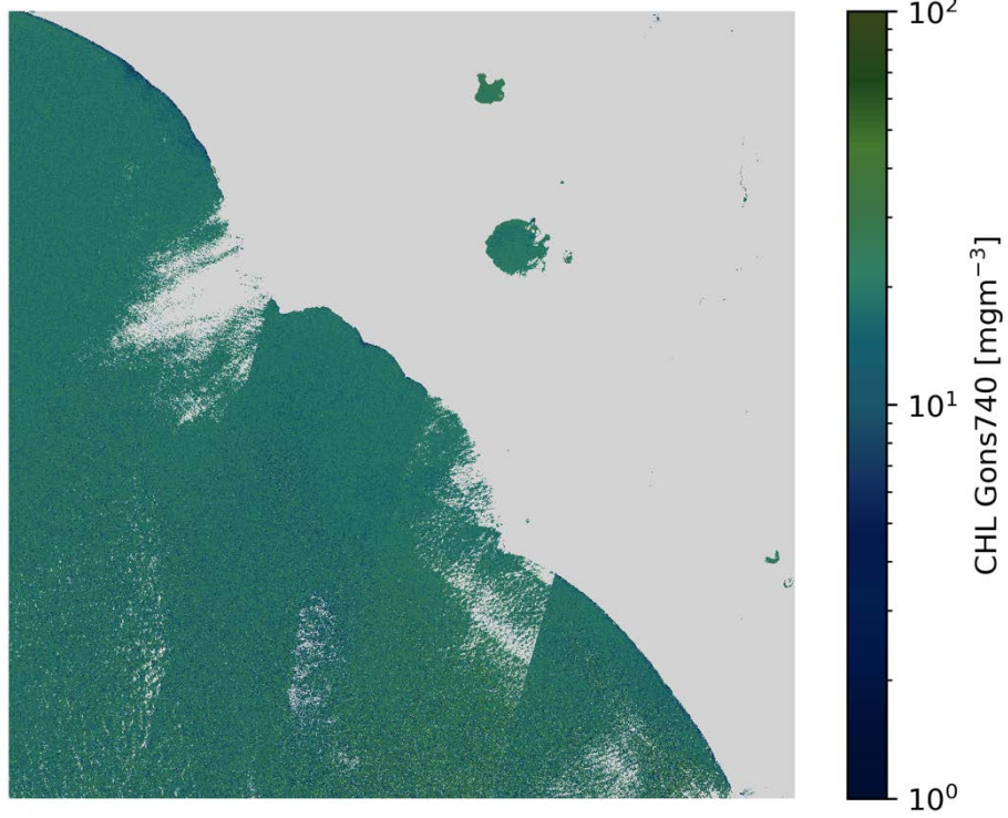
CHL Gons740 S2A/MSI 2020-07-14 (10:09 UTC)
