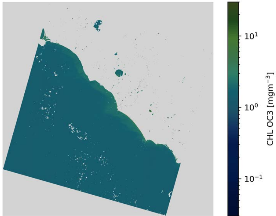
CHL OC3 L8/OLI 2020-03-24 (09:53 UTC)
