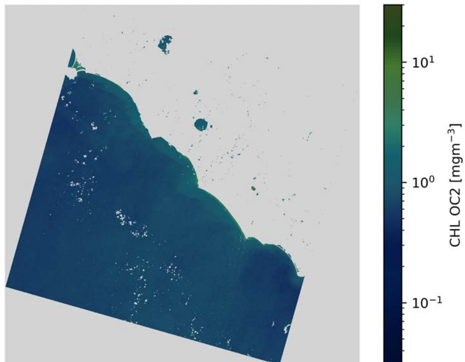
CHL OC2 L8/OLI 2020-03-24 (09:53 UTC)
