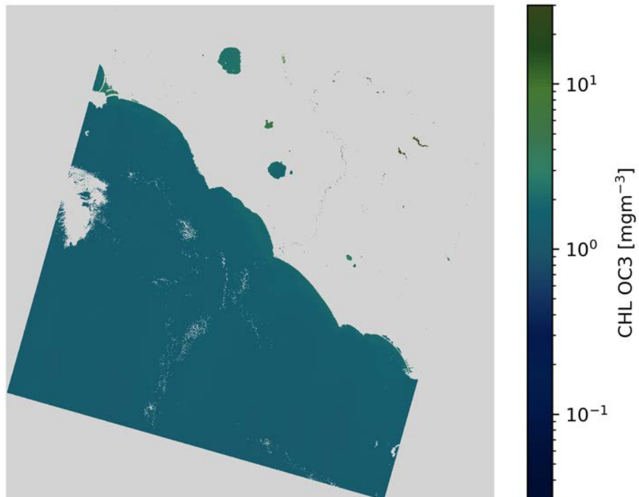
CHL OC3 L8/OLI 2020-04-09 (09:53 UTC)
