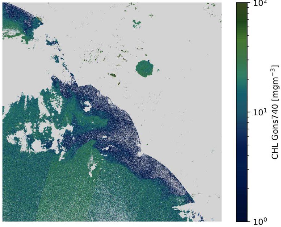
CHL Gons740 S2A/MSI 2020-12-31 (10:09 UTC)
