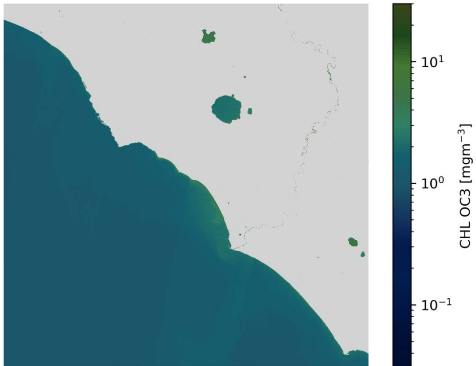
CHL OC3 S2B/MSI 2020-04-10 (10:09 UTC)
