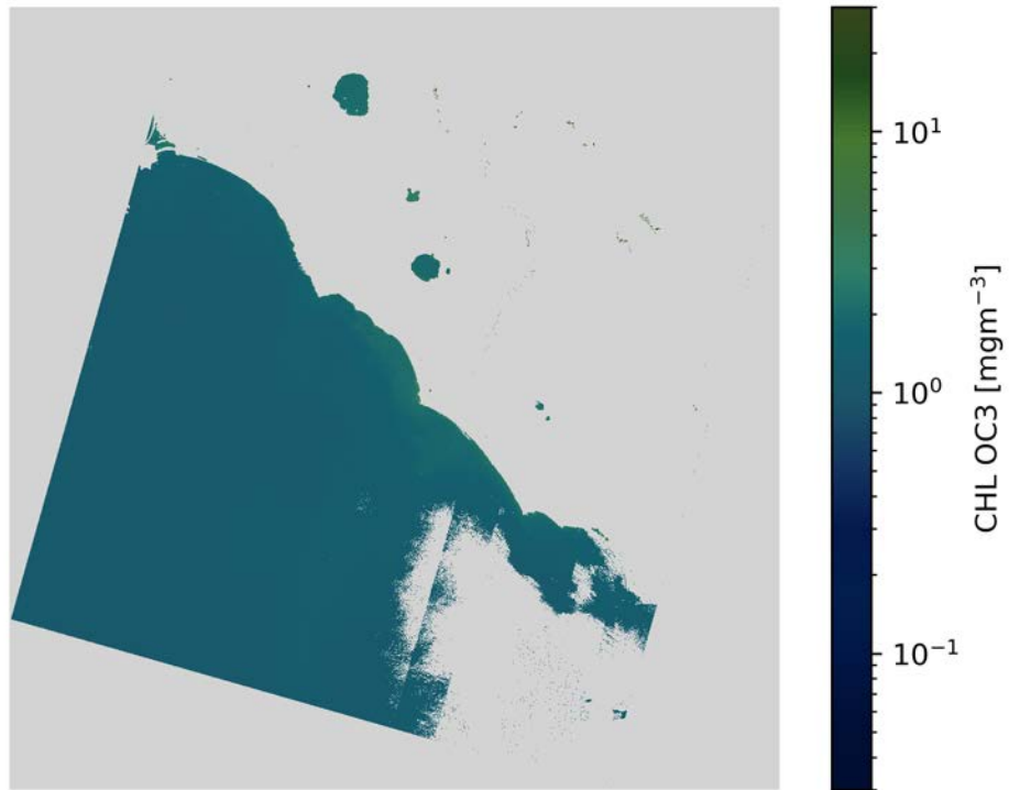
CHL OC3 L8/OLI 2020-07-30 (09:53 UTC)
