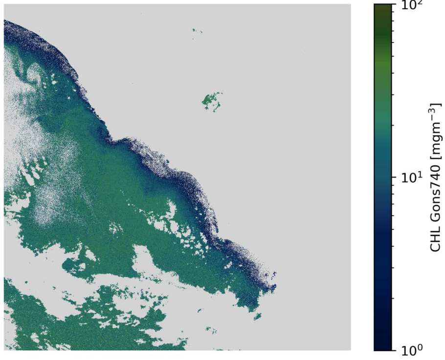
CHL Gons740 S2A/MSI 2020-03-06 (10:09 UTC)
