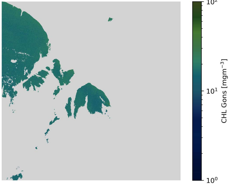
CHL Gons S2B/MSI 2020-03-21 (10:09 UTC)
