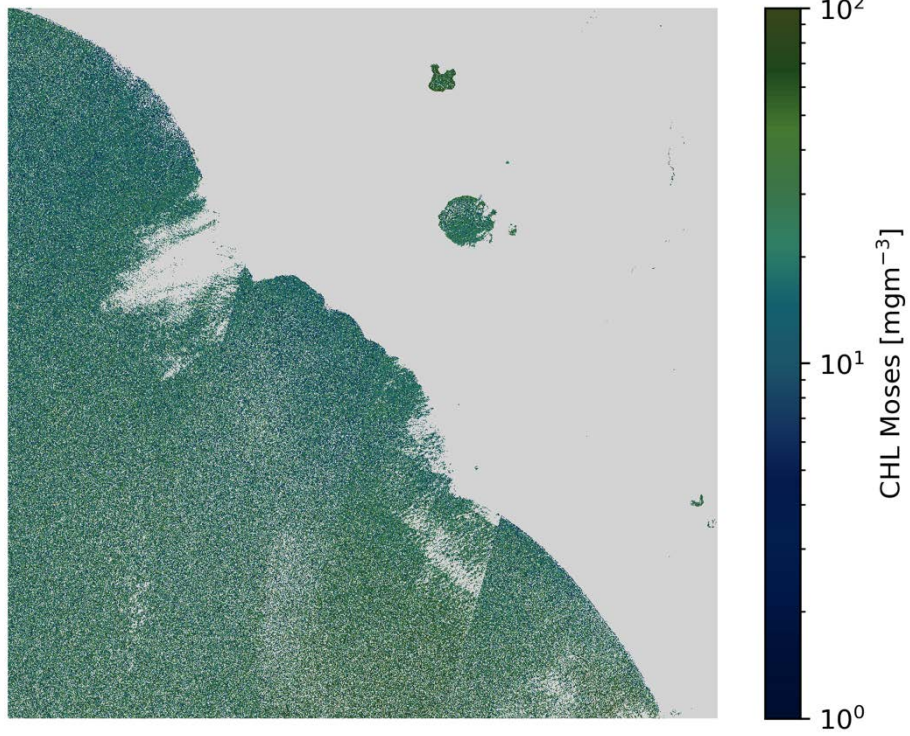
CHL Moses S2A/MSI 2020-07-14 (10:09 UTC)
