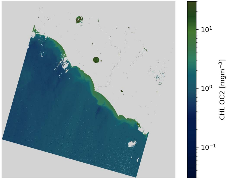
CHL OC2 L8/OLI 2020-02-05 (09:53 UTC)
