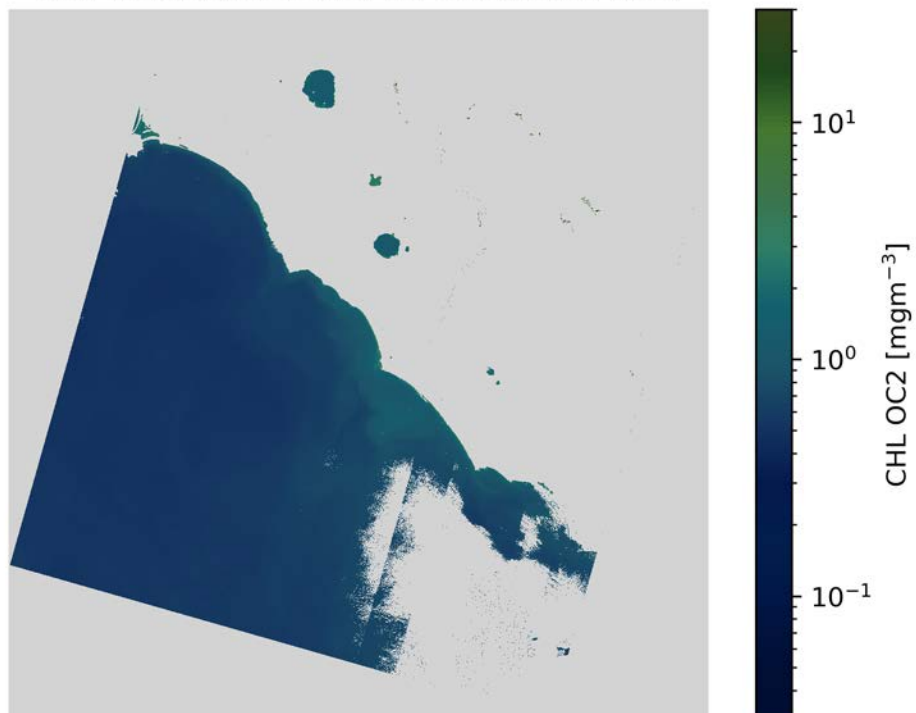
CHL OC2 L8/OLI 2020-07-30 (09:53 UTC)
