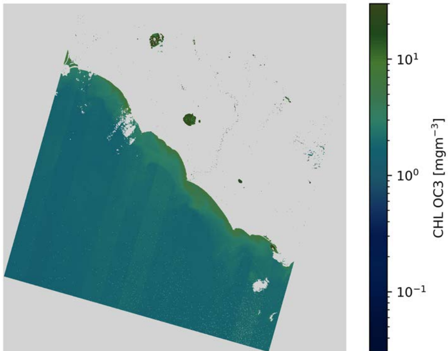
CHL OC3 L8/OLI 2020-02-05 (09:53 UTC)
