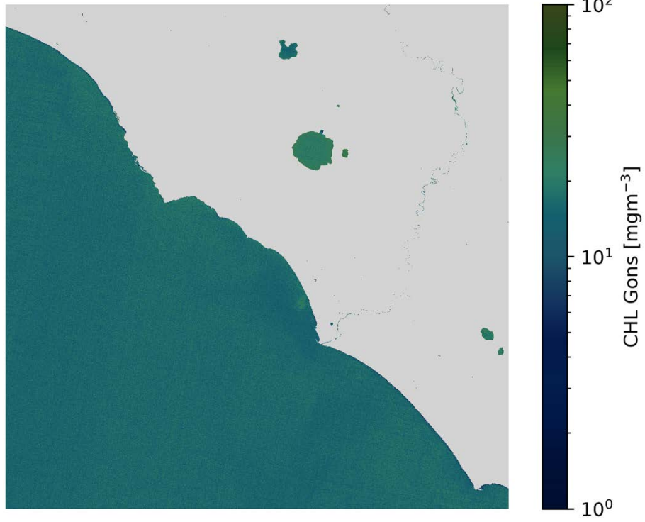
CHL Gons S2B/MSI 2020-04-10 (10:09 UTC)
