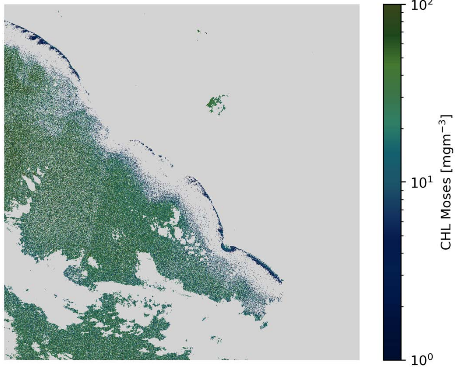
CHL Moses S2A/MSI 2020-03-06 (10:09 UTC)
