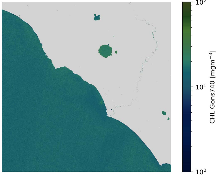
CHL Gons740 S2B/MSI 2020-04-10 (10:09 UTC)
