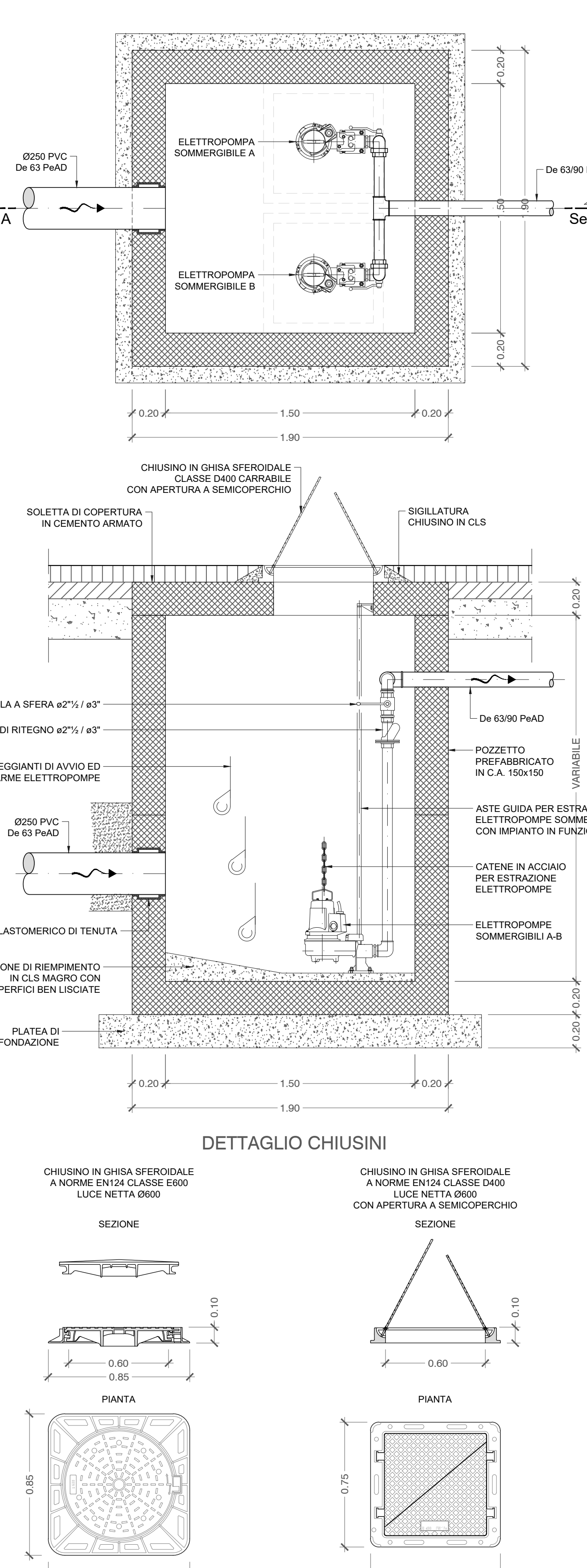
DETTAGLIO POZZETTO DI SOLLEVAMENTO n°1-2-3-4
