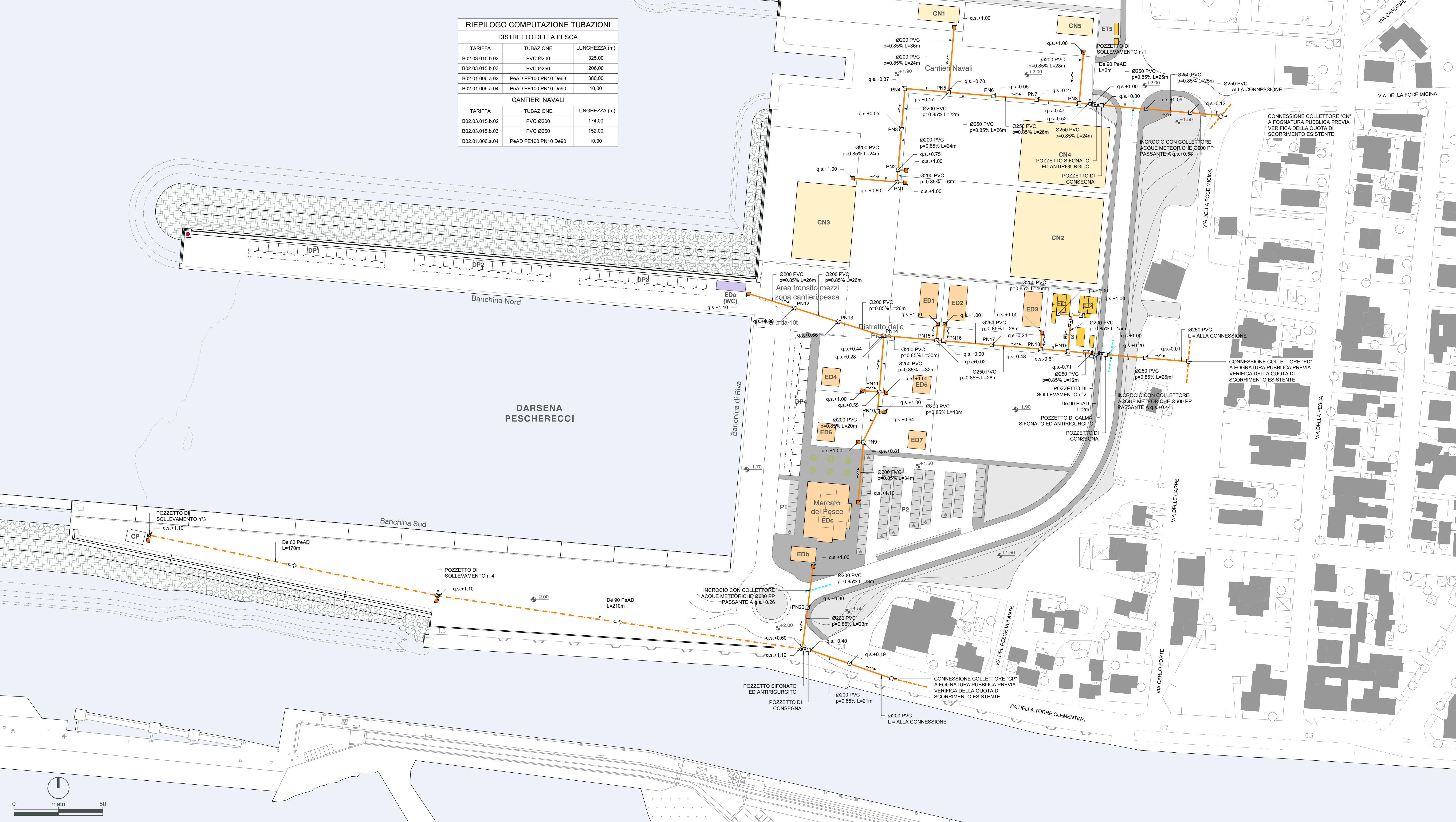
PLANIMETRIA DI PROGETTO Scala 1:1.000
