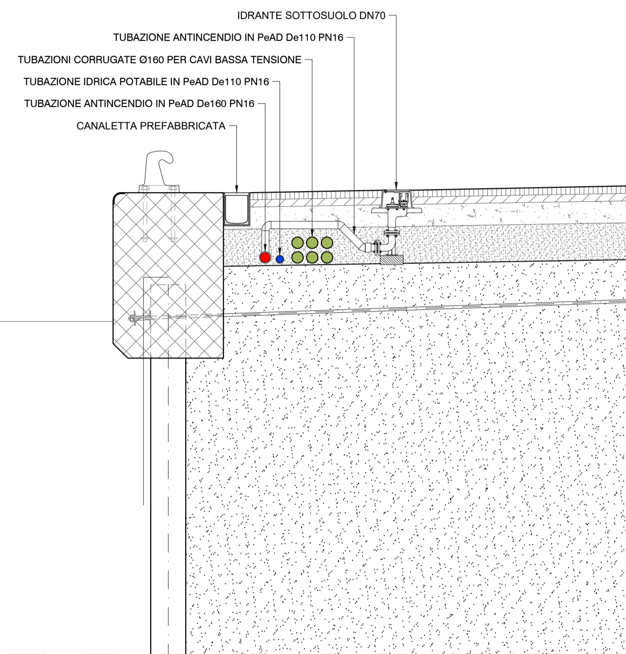
SEZIONE TIPOLOGICA ALLACCIO UTENZA IDRICA ANTINCENDIO Scala 1:50
