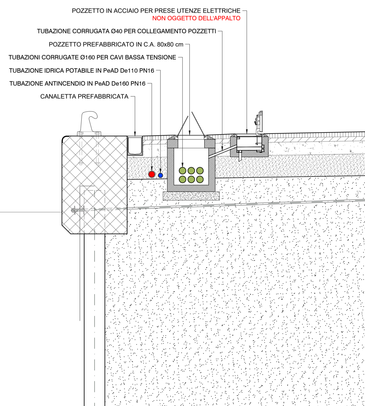
SEZIONE TIPOLOGICA ALLACCIO UTENZA ELETTRICA Scala 1:50
