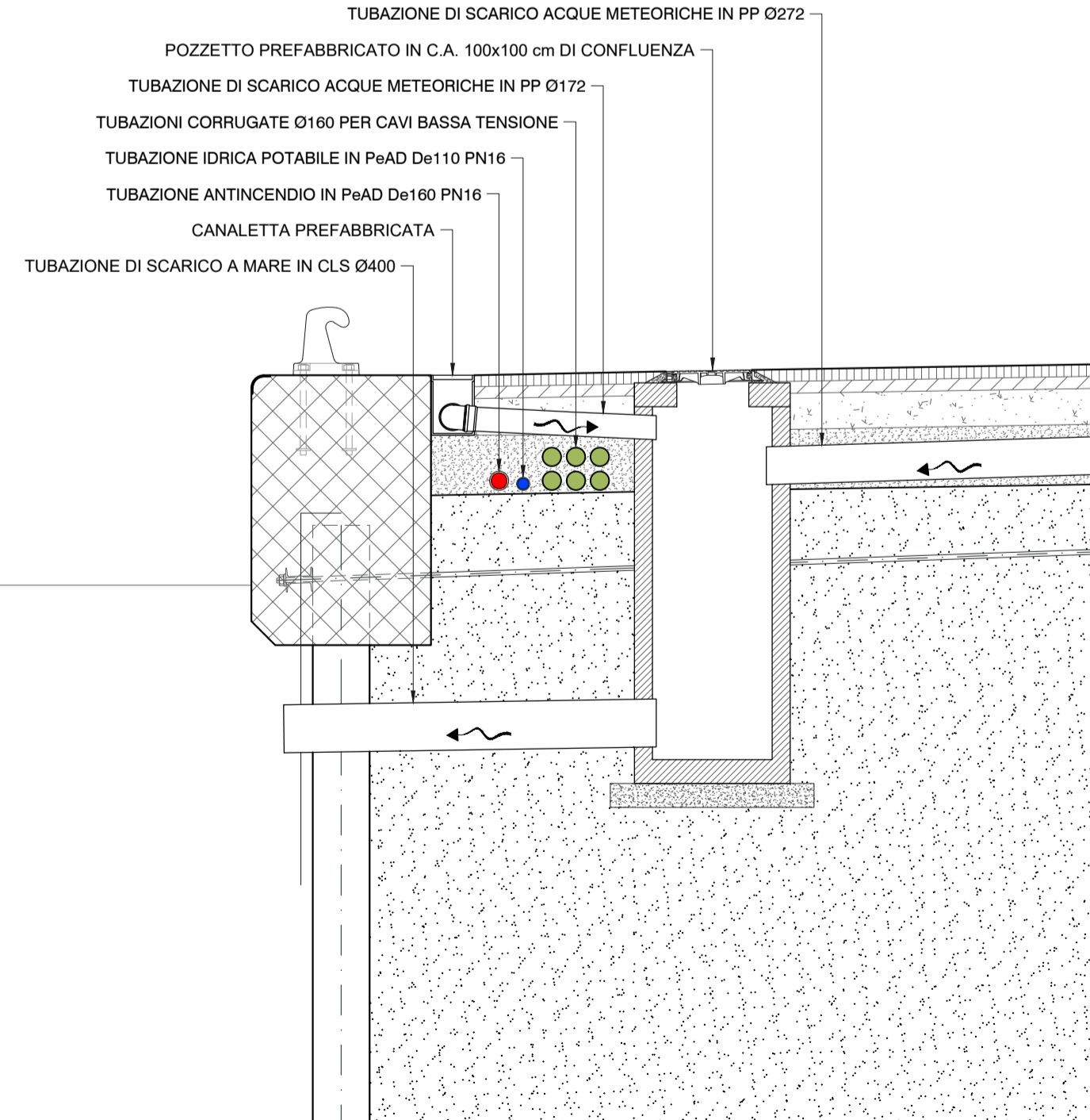
SEZIONE TIPOLOGICA SCARICO A MARE Scala 1:50
