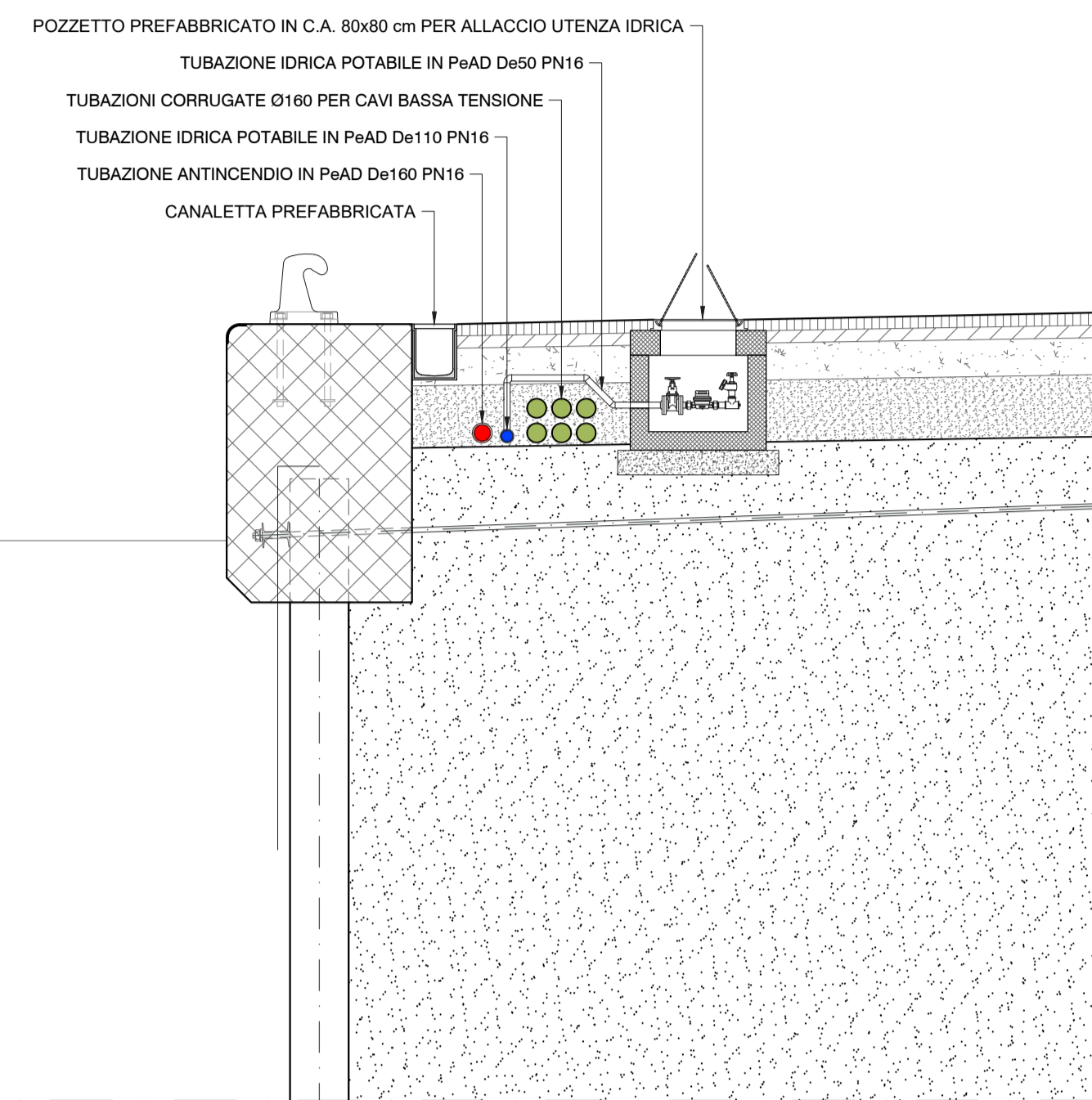
SEZIONE TIPOLOGICA ALLACCIO UTENZA IDRICA POTABILE Scala 1:50
