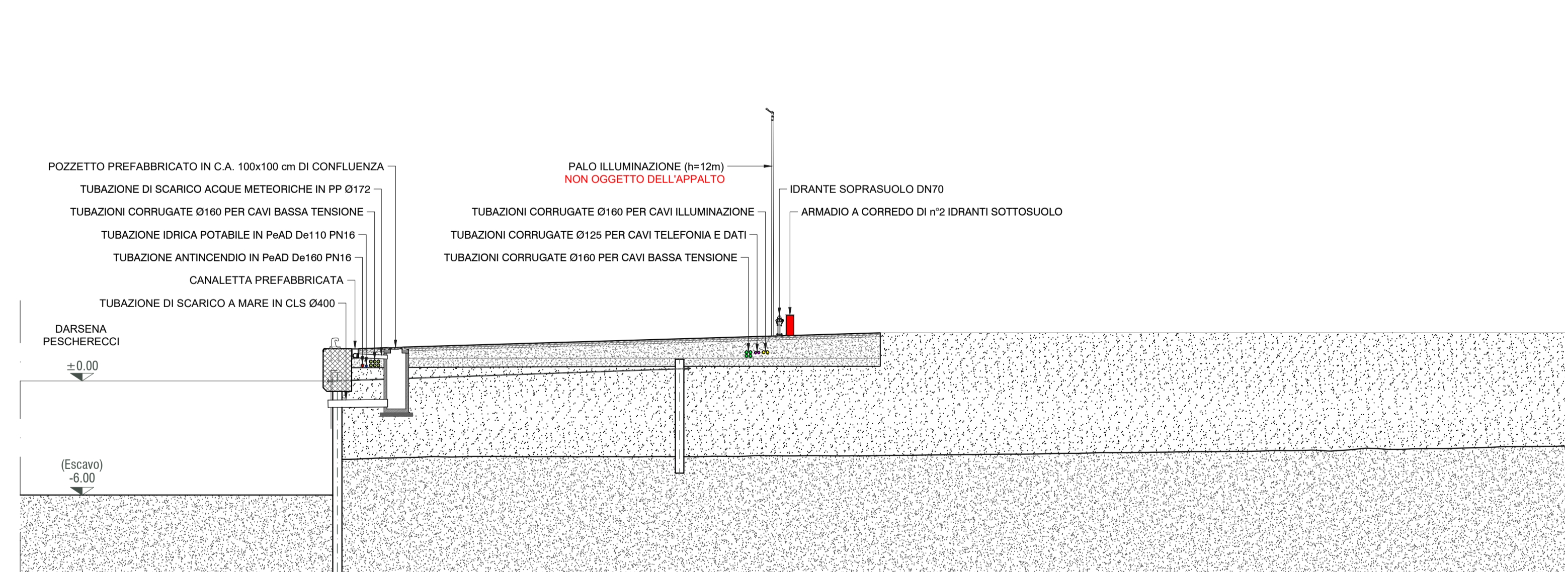
SEZIONE TIPOLOGICA BANCHINA RIVA Scala 1:200
