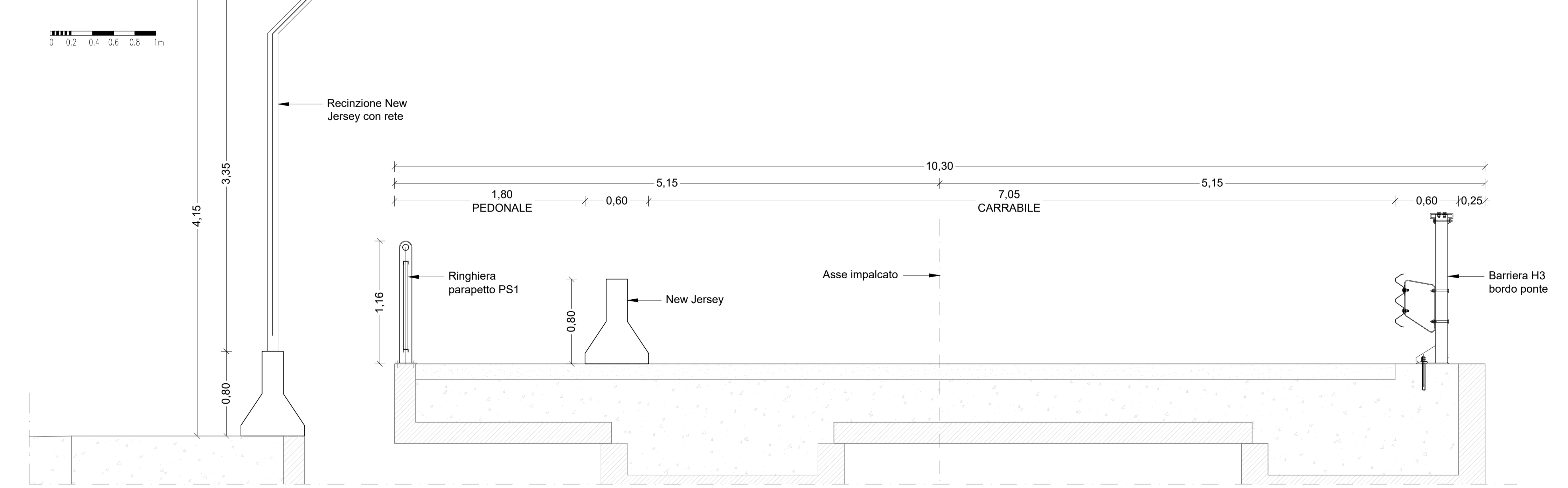
SEZIONE TRASVERSALE TIPO
