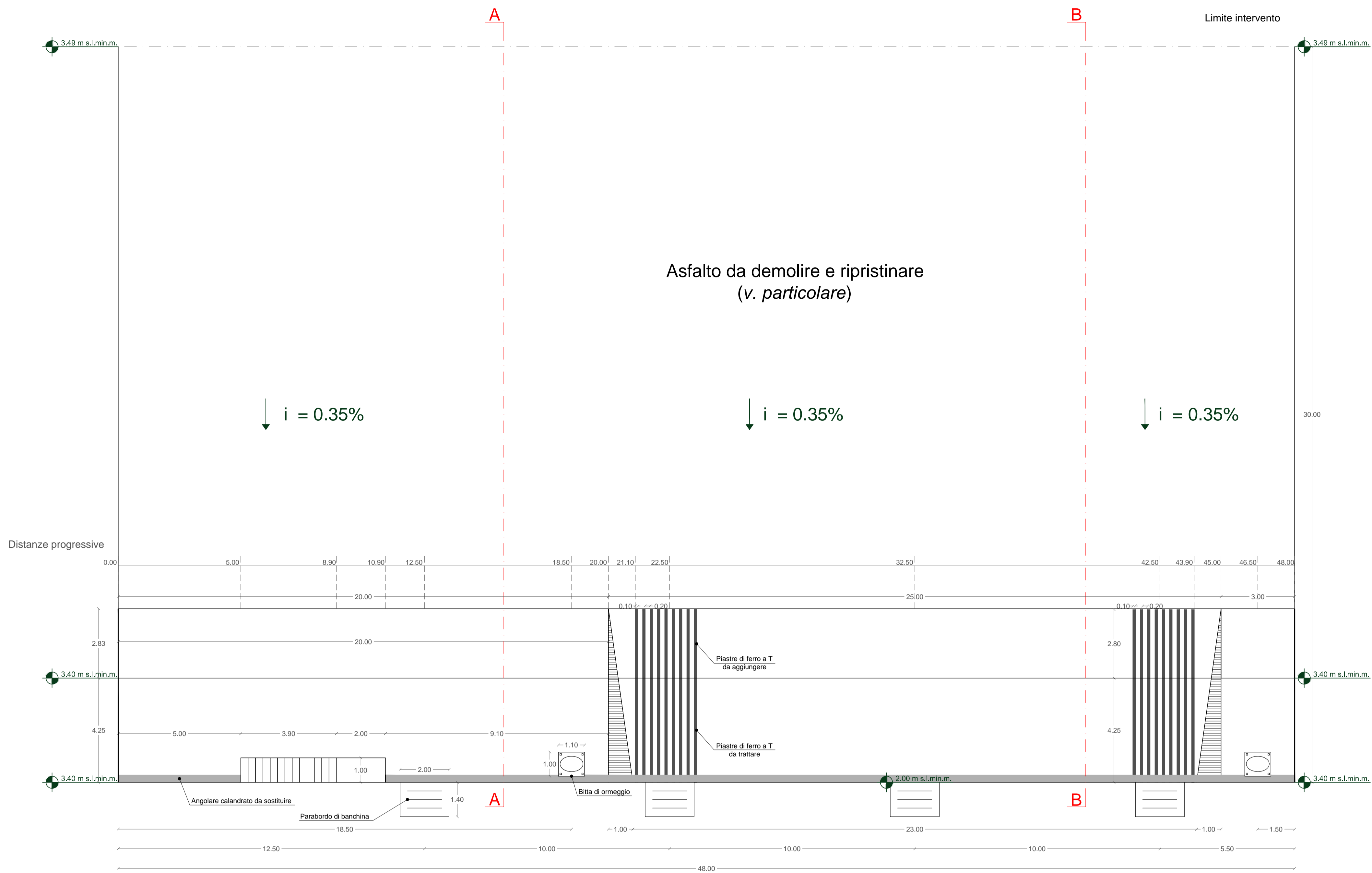
Planimetria - Tratto E (Scala 1:100)
