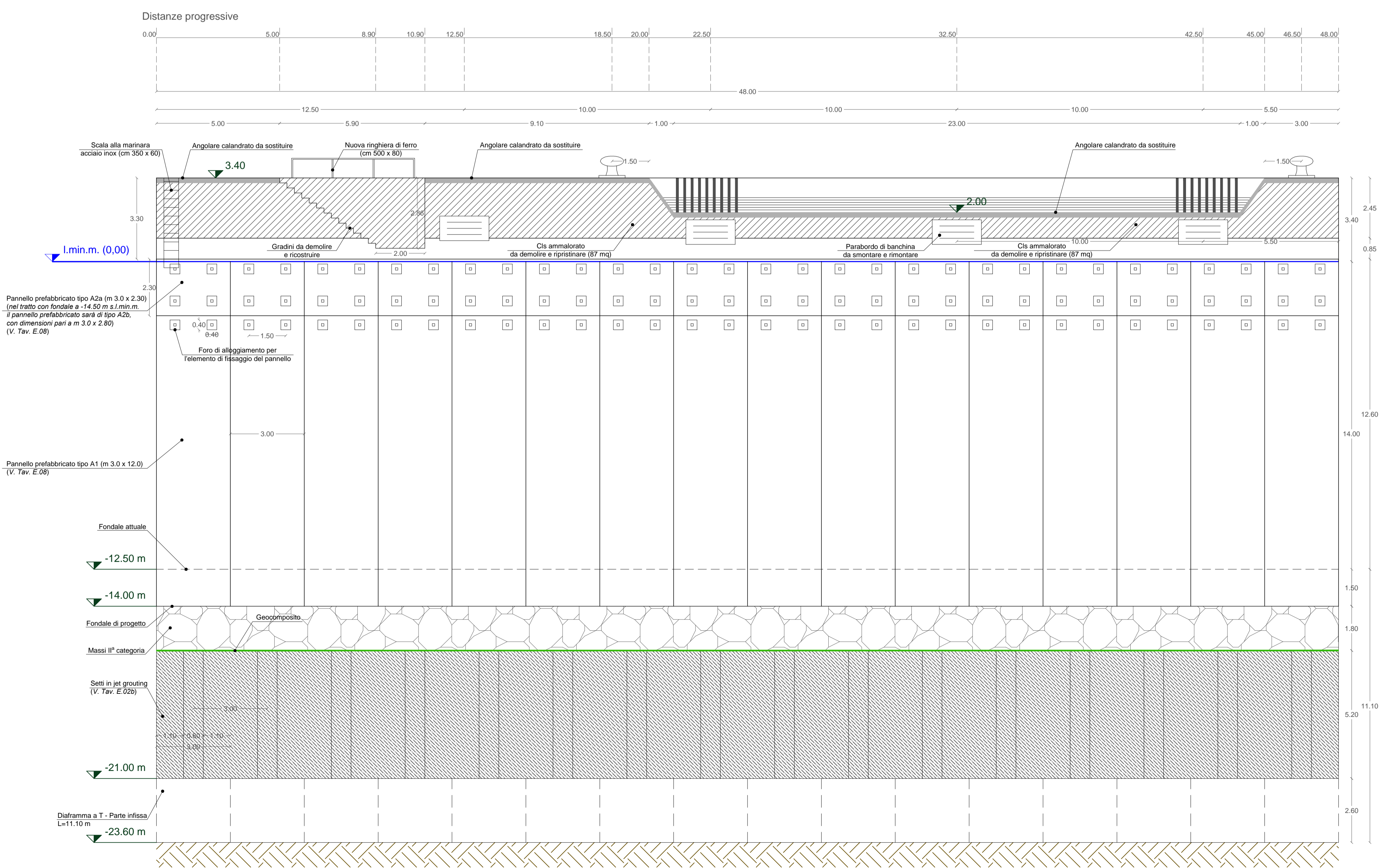
Prospetto - Tratto E (Scala 1:100)
