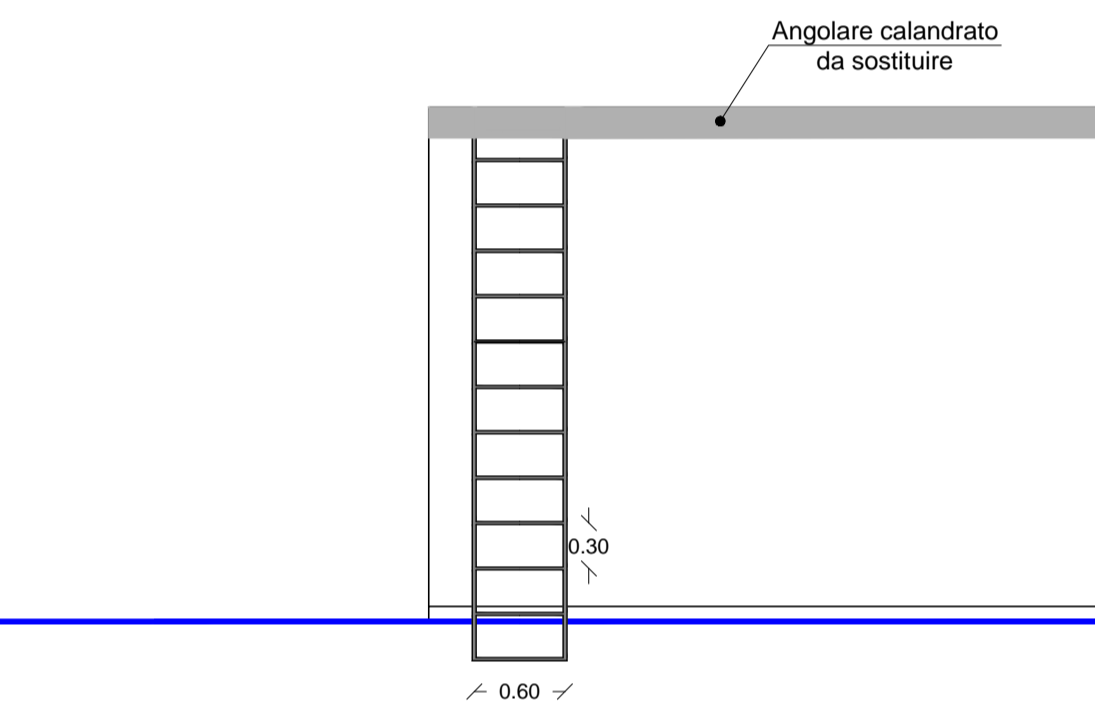
Particolare angolare calandrato (scala 1:25)
