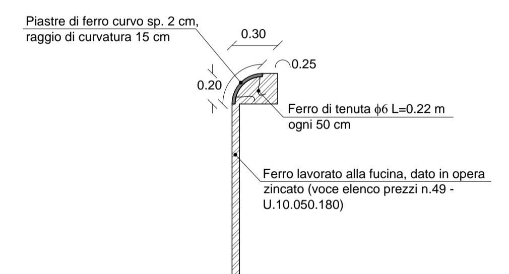
Particolare angolare calandrato (scala 1:25)
