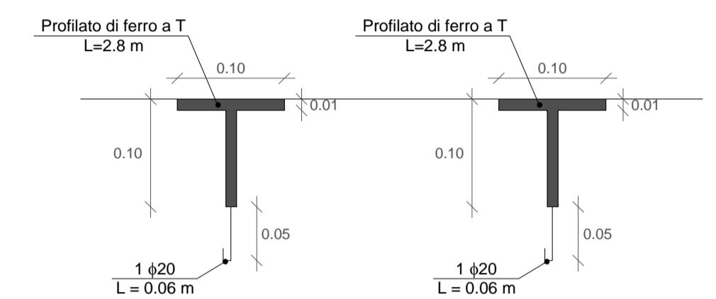
Particolare profilati di ferro a T (scala 1:5)
