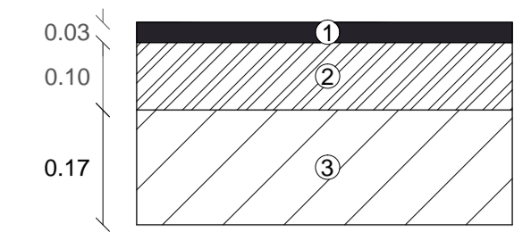
Particolare pavimentazione di progetto (scala 1:10)
