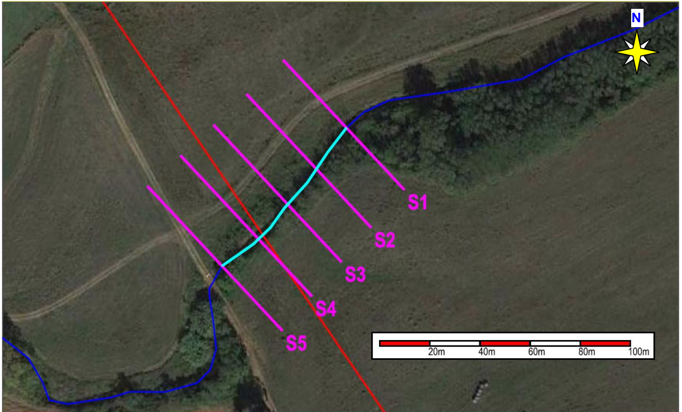
Fig.5.3/A: Foto aerea, con tronco d'alveo analizzato e sezioni di input
