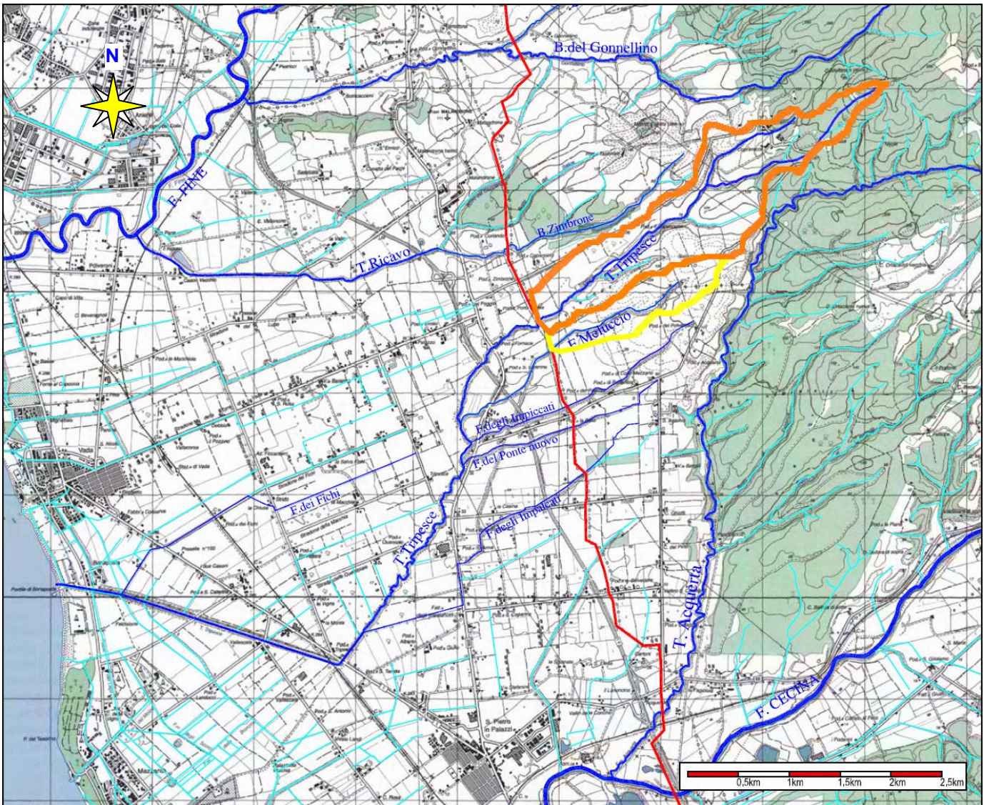
Fig.4.3/A: Bacini Imbriferi sottesi dalle sezioni di studio
