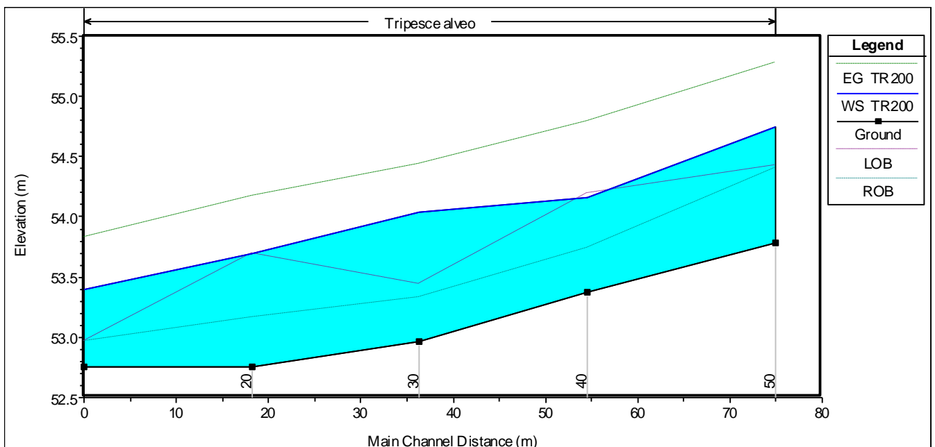
Fig.5.4/B: Schermata di Output del programma – Profilo longitudinale
