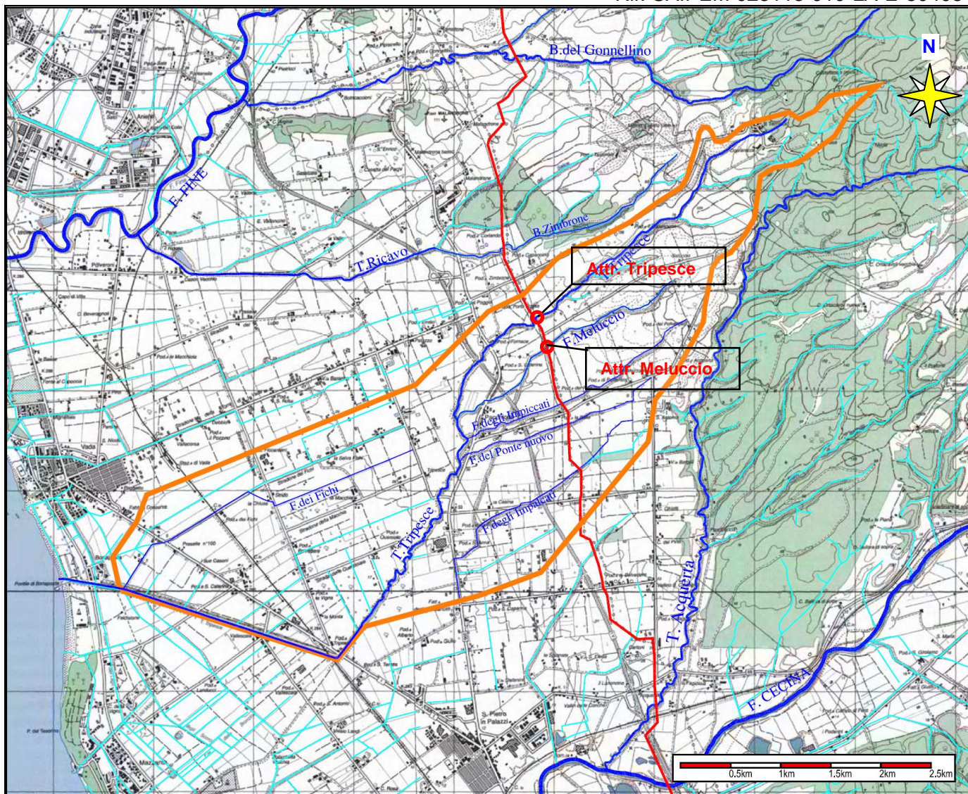
Fig.3.1/A: Bacino complessivo del Tripesce con indicazione ambiti di attraversamento in esame
