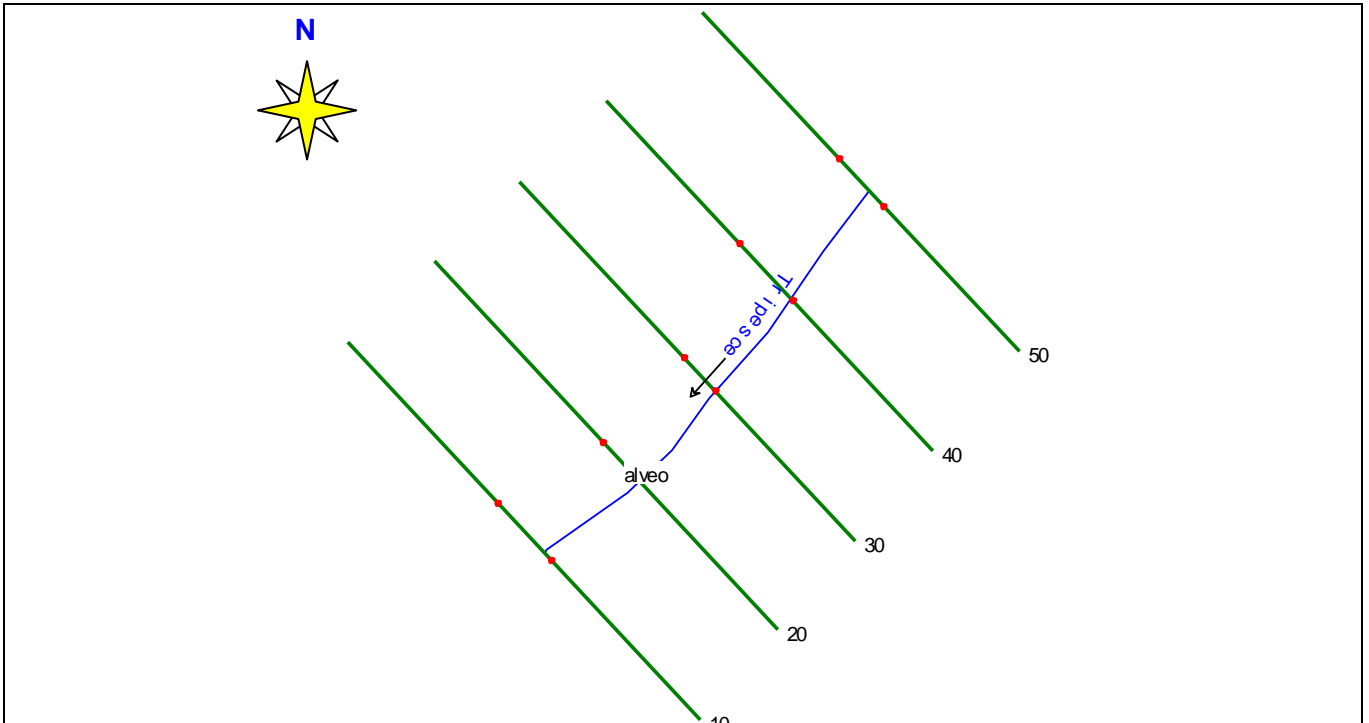
Fig.5.3/B: Modellazione geometrica in Hec Ras (RS50 a monte e RS10 a valle)
