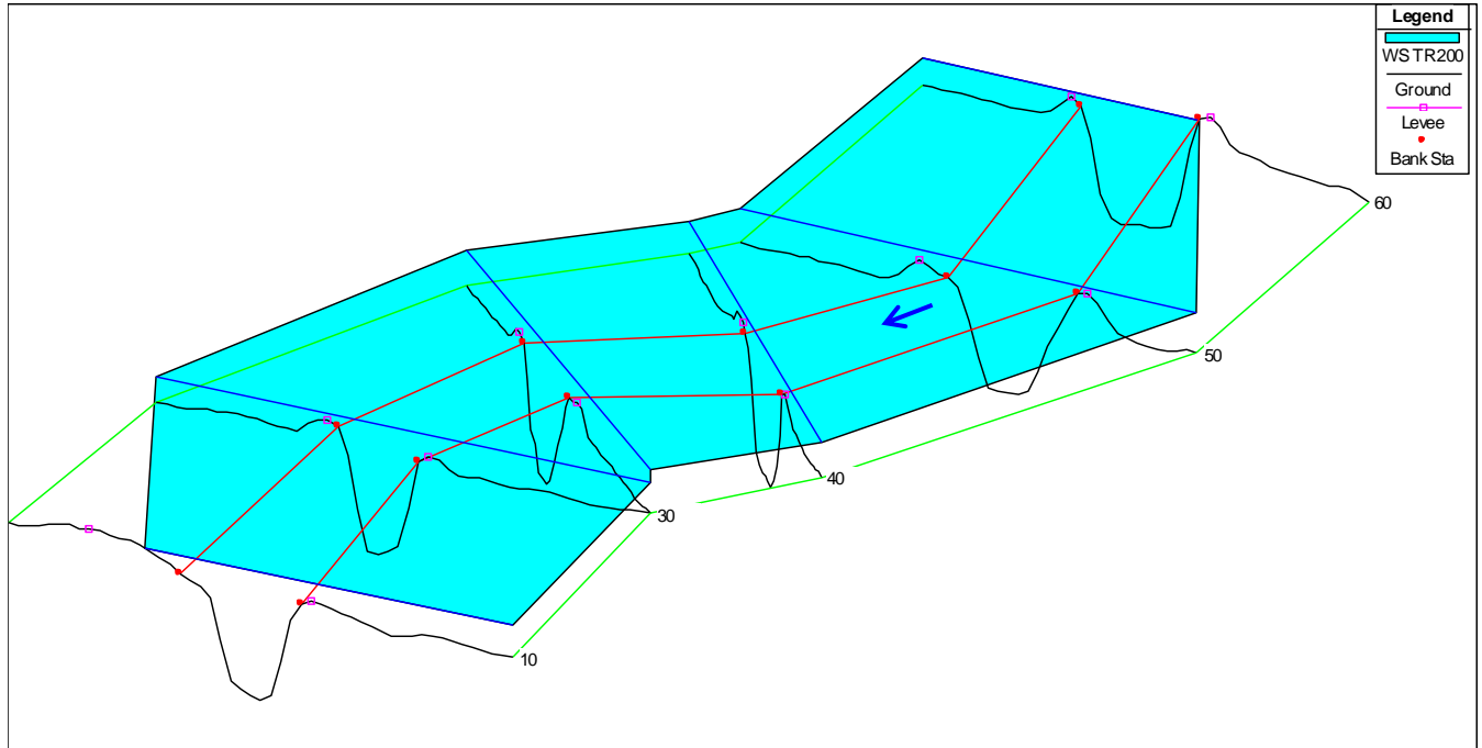
Fig.5.3/A: Schermata di Output del programma – visione prospettica (RS60: monte /RS10: valle)
