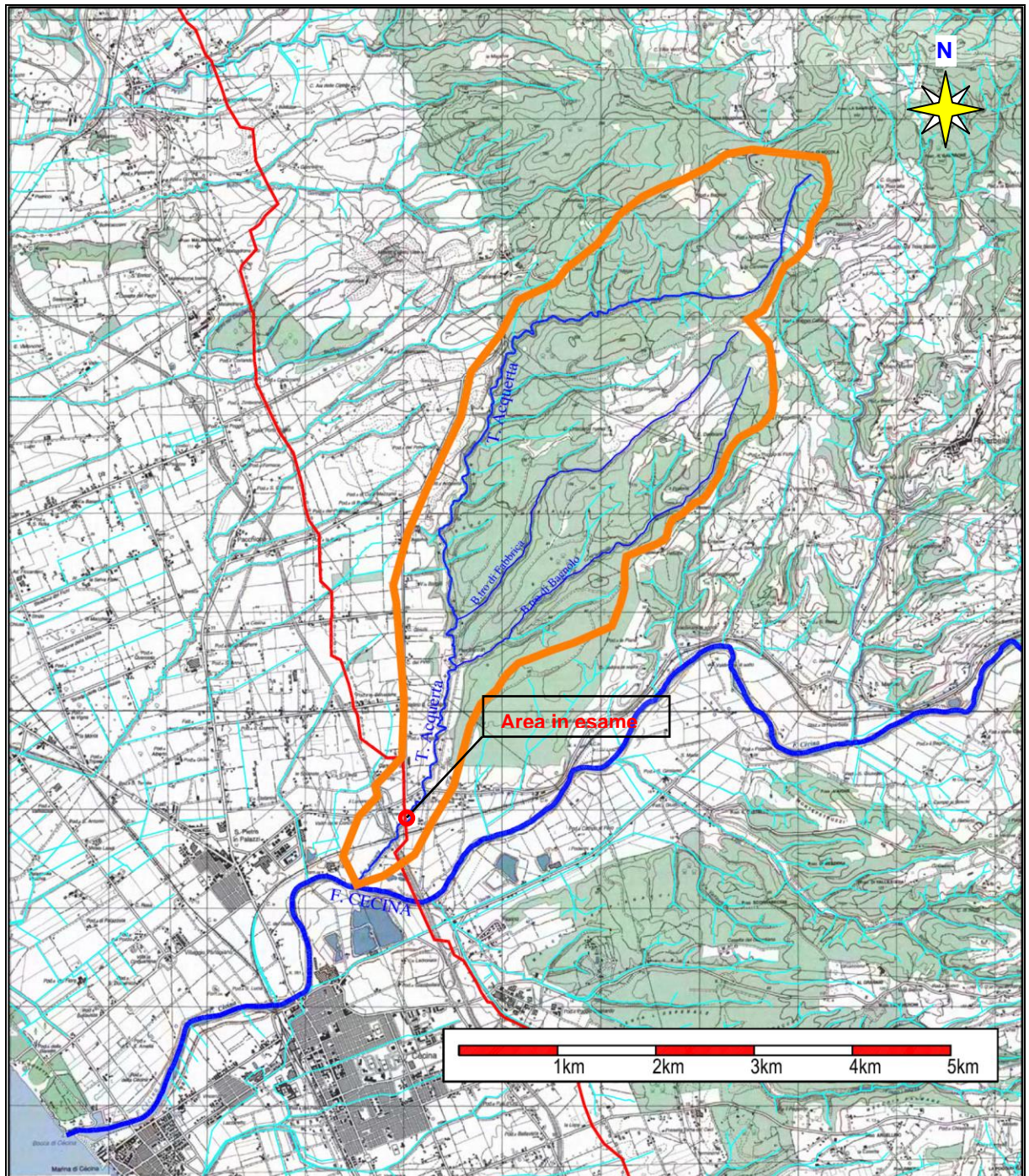
Fig.3.1/A: Bacino complessivo del corso d'acqua ed indicazione ambito di attraversamento
