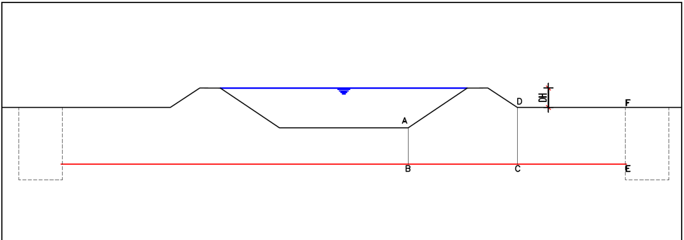
Fig. 8.3/A: Sezione schematica per le verifiche al sifonamento
