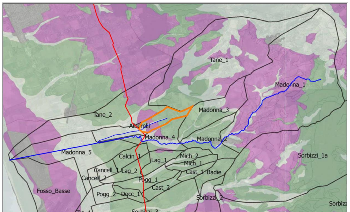
Fig.4.5/A: Sottobacini individuati per il corso d'acqua
