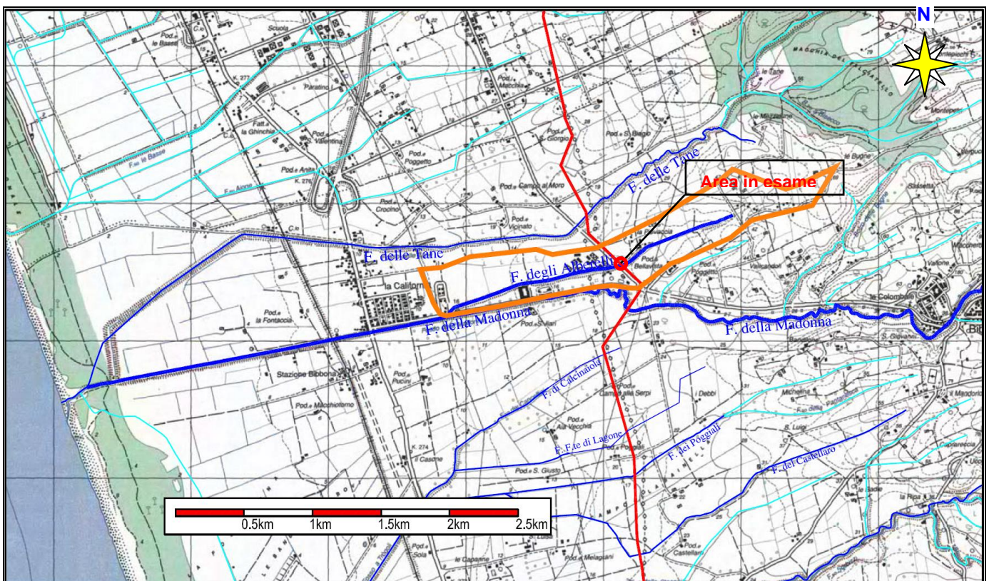
Fig.3.1/A: Bacino complessivo del corso d'acqua ed indicazione dell'ambito di studio
