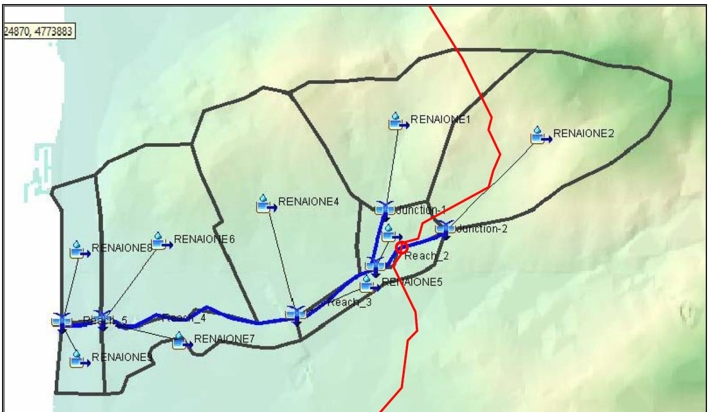
Fig.4.5/A: Planimetria con sottobacini ed elementi idrologici considerati
