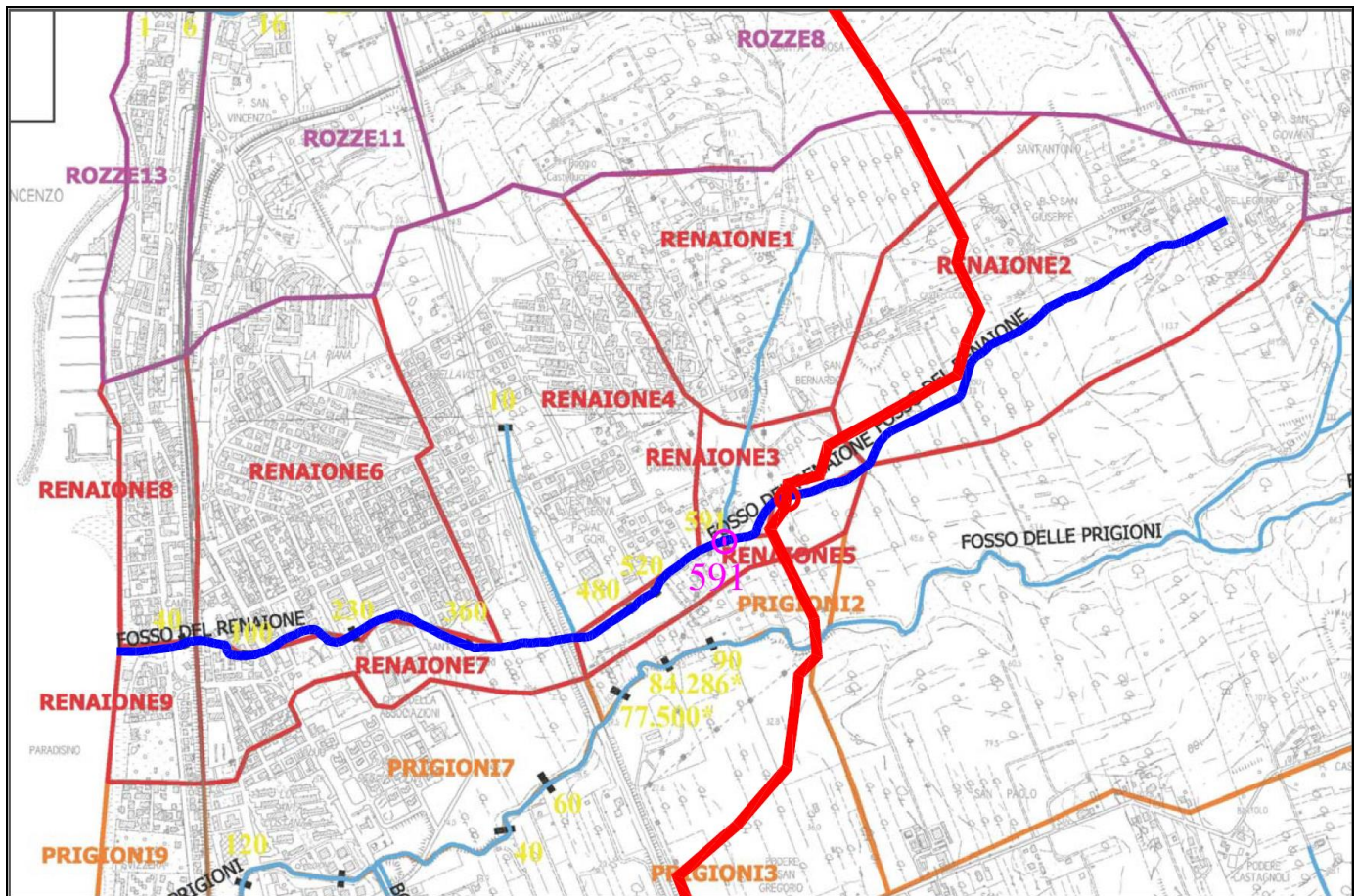
Fig.4.6/A: Inquadramento reticolo e sottobacini
