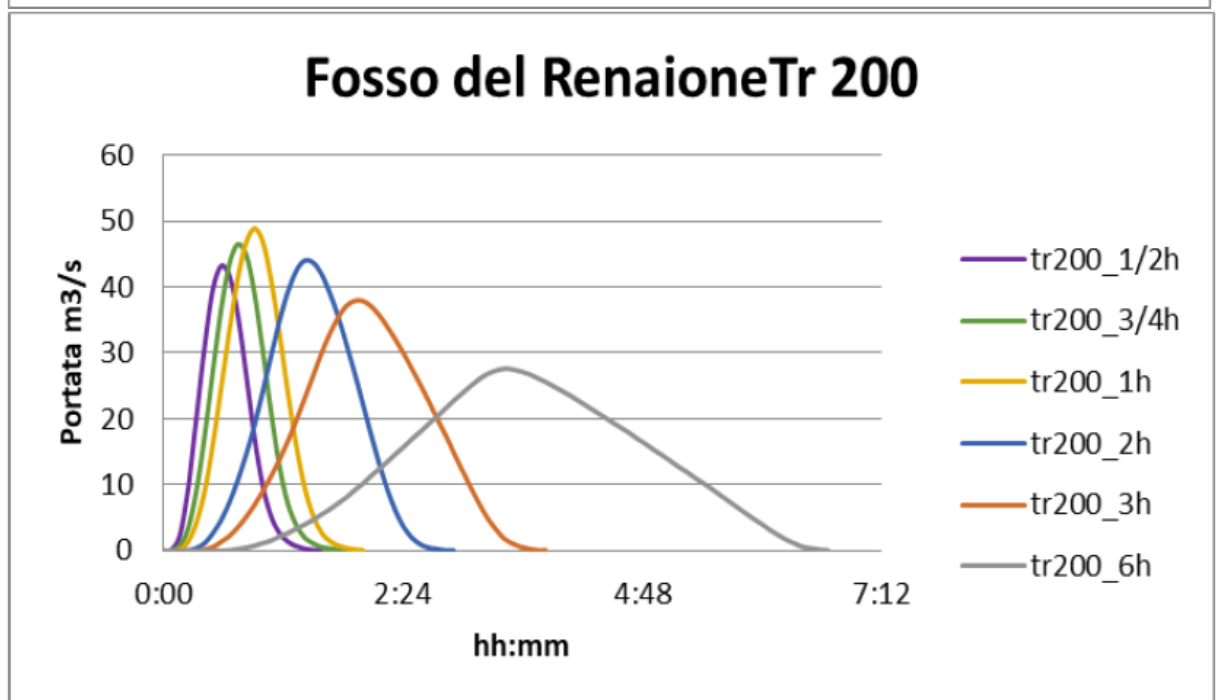
Fig.4.5/B: Idrogrammi di piena
