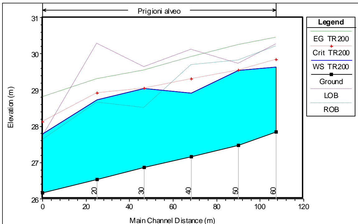
Fig.5.3/B: Schermata di Output del programma – Profilo longitudinale
