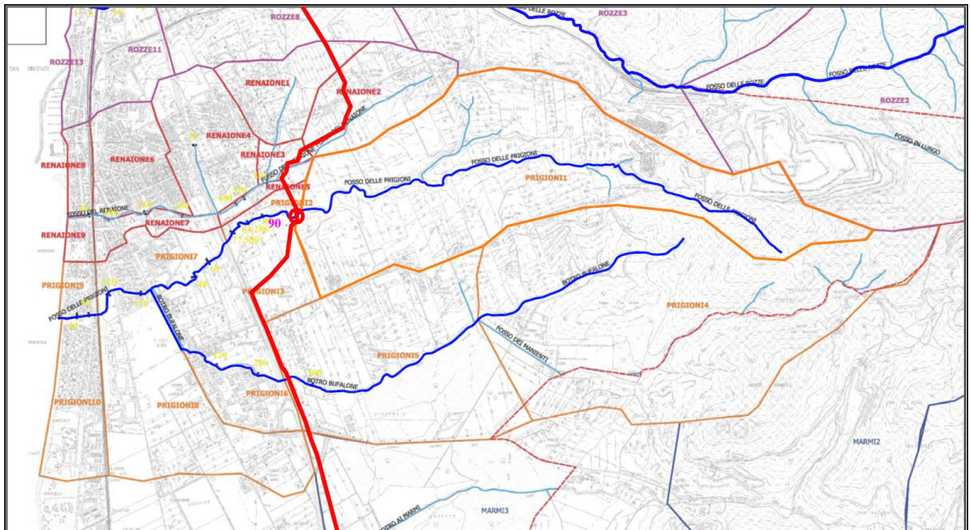
Fig.4.6/A: Inquadramento reticolo e sottobacini
