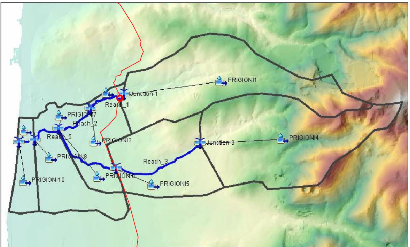
Fig.4.5/A: Planimetria con sottobacini ed elementi idrologici considerati
