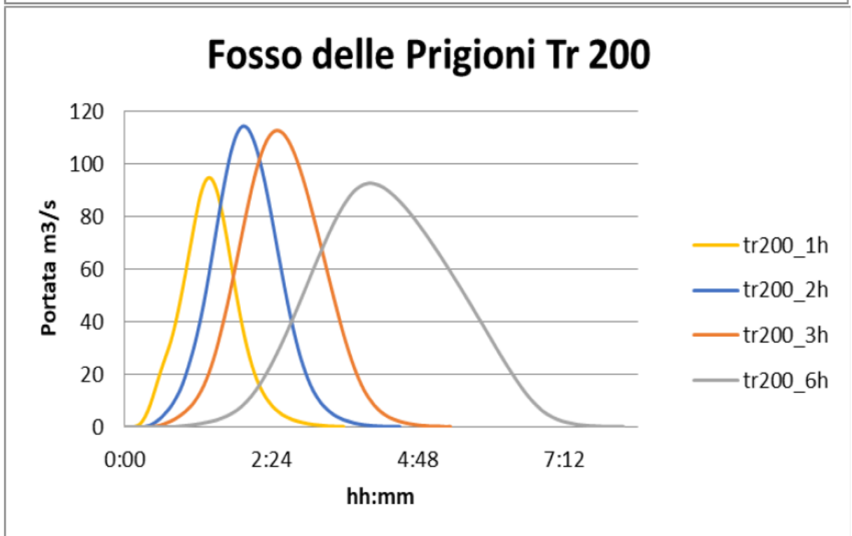
Fig.4.5/B: Idrogrammi di piena
