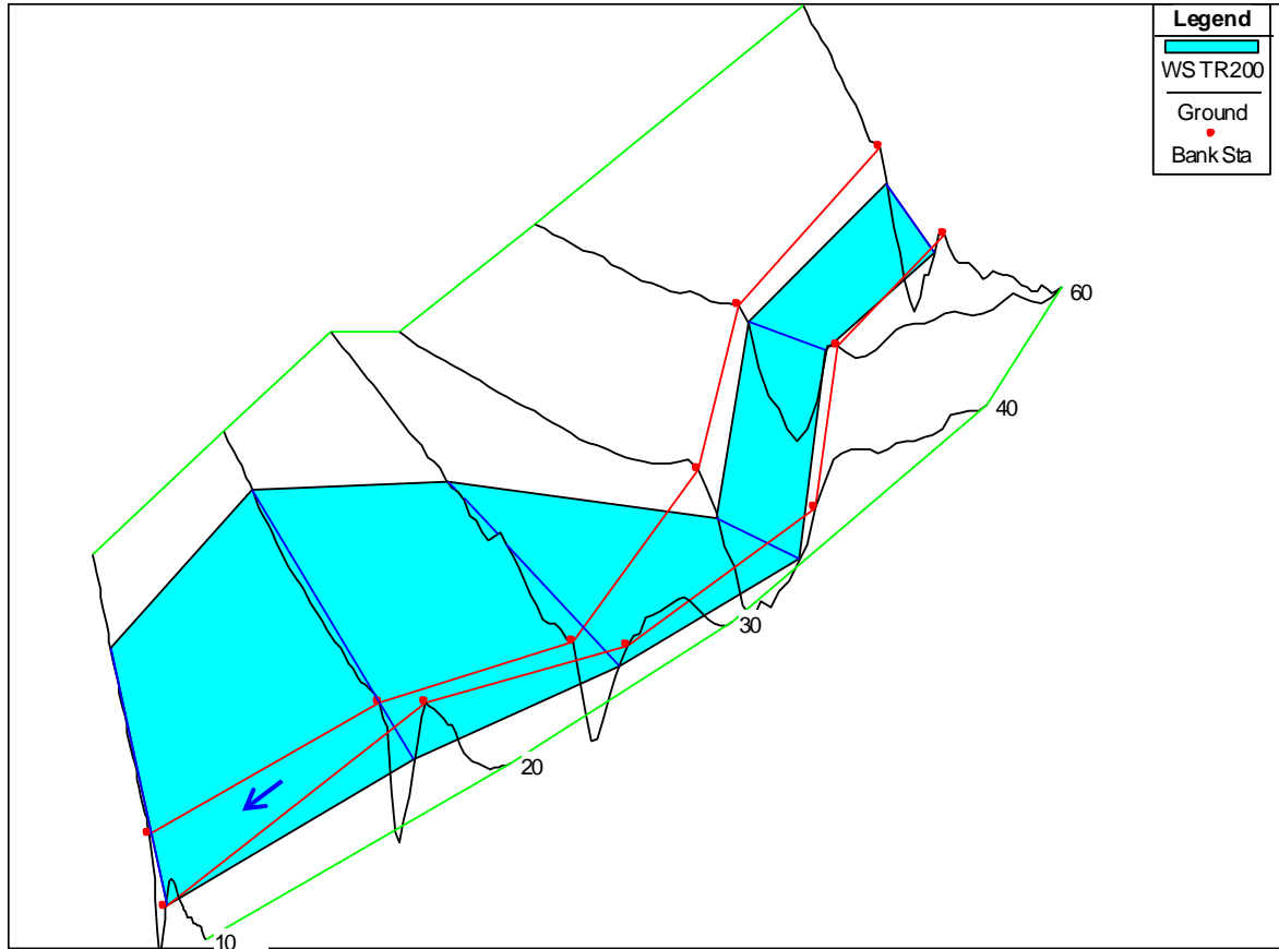
Fig.5.3/A: Schermata di Output del programma – visione prospettica (RS60: monte /RS10: valle)
