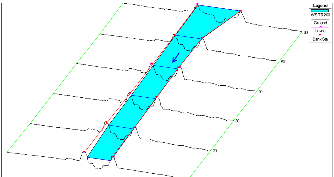
Fig.5.3/A: Schermata di Output del programma – visione prospettica (RS60: monte /RS10: valle)
