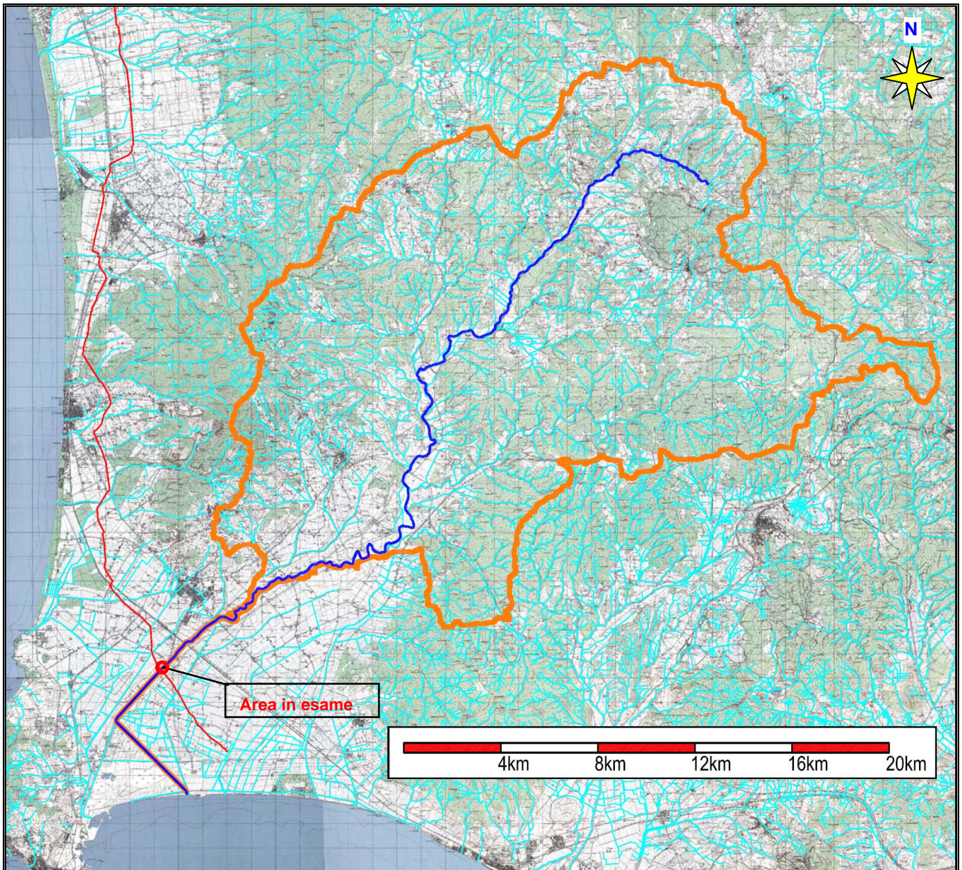
Fig.3.1/A: Bacino complessivo del corso d'acqua ed indicazione dell'ambito di studio
