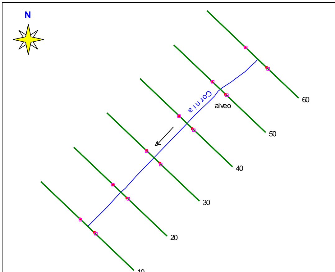
Fig.5.2/B: Modellazione geometrica in Hec Ras (RS60 a monte e RS10 a valle)
