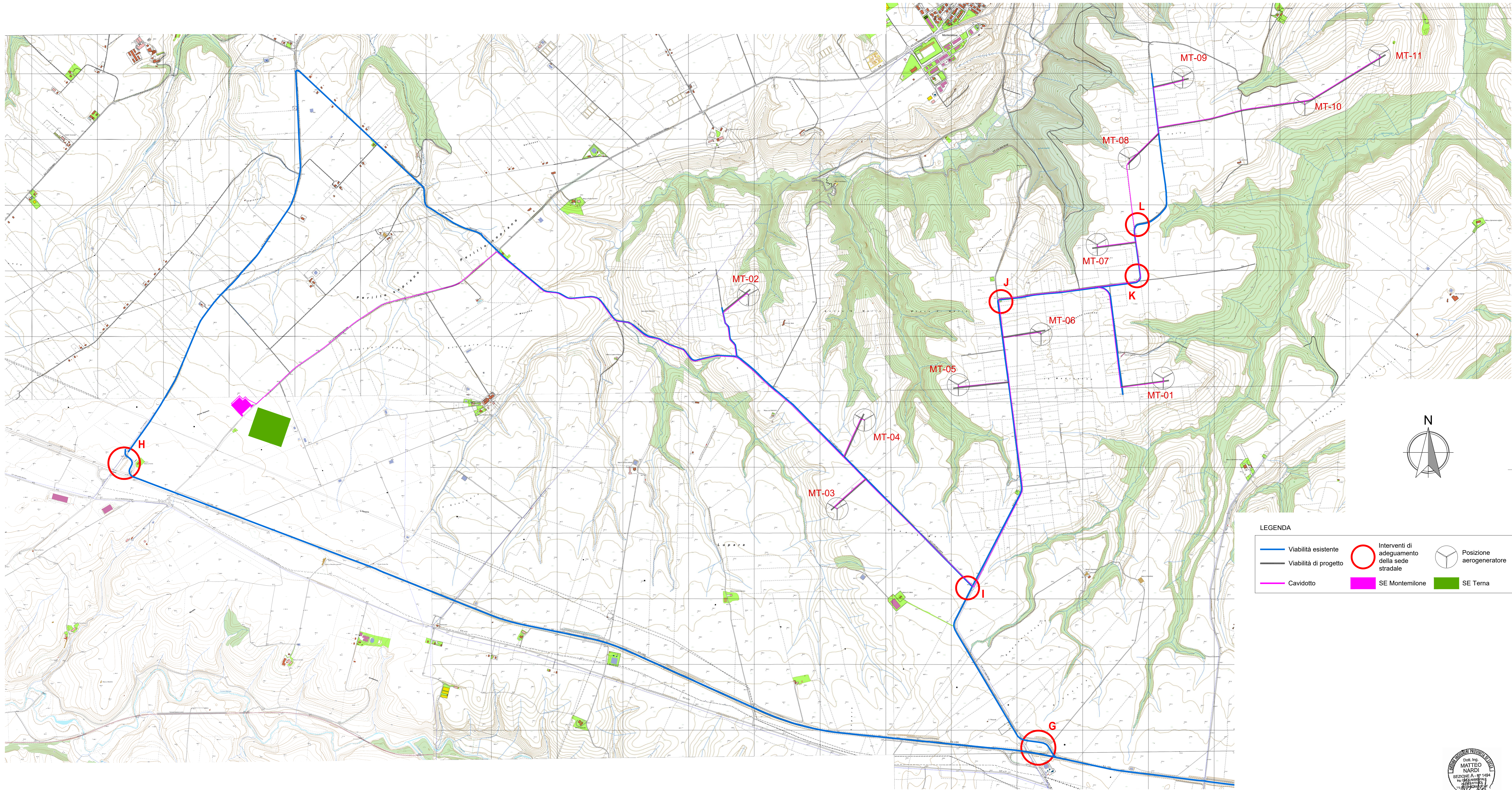
INTERVENTI ADEGUAMENTO VIABILITÀ ESISTENTE AREA DI IMPIANTO scala 1:10.000
