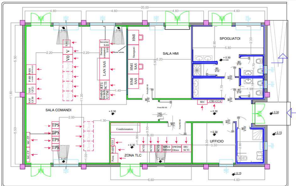
Figura 13 – planimetria edificio comandi
