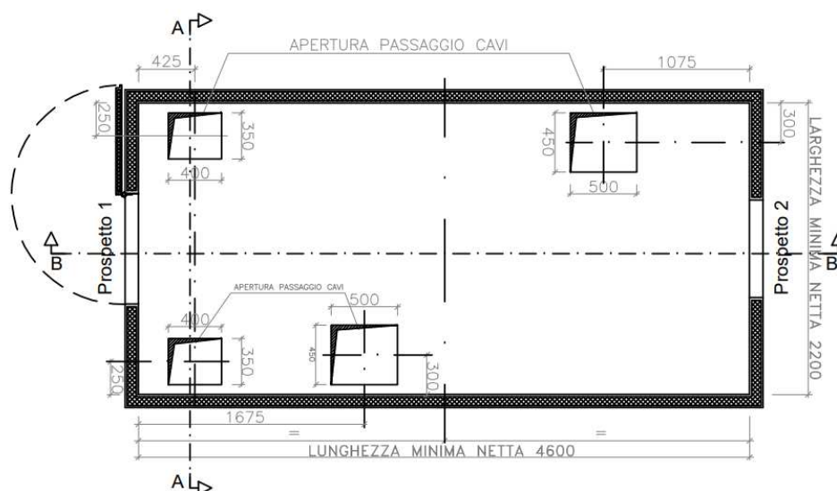
Figura 17 – planimetria chioschi
