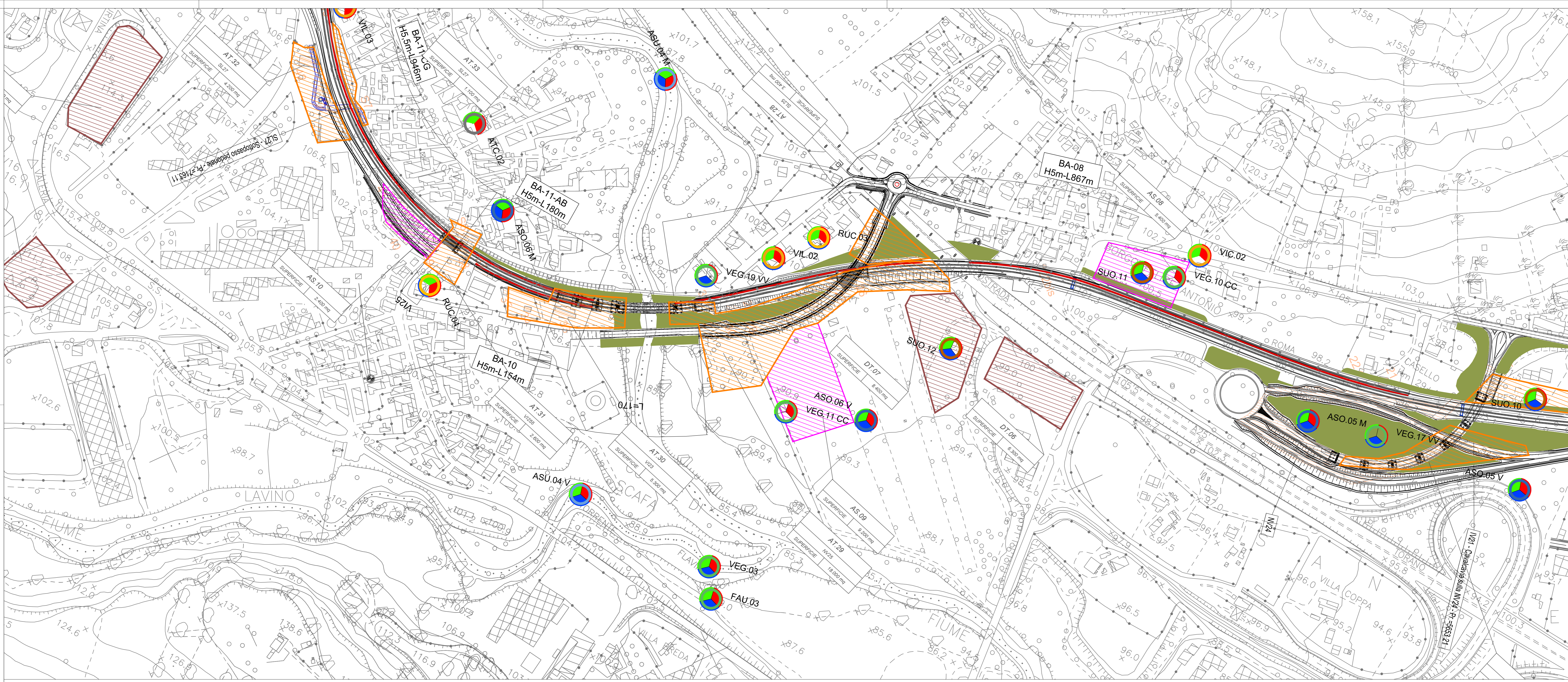
TRATTO E - PLANIMETRIA DI LOCALIZZAZIONE DEI PUNTI DI MONITORAGGIO
