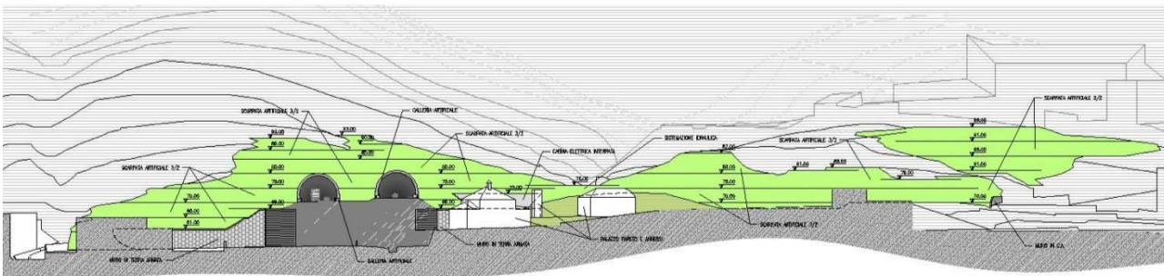
Fig. 5.1.4 – Prospetto della sistemazione finale (cfr. AUA0151-2)
