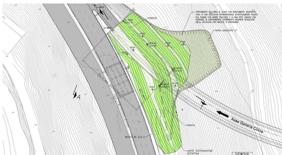
Fig. 3.5.1 – Imbocco galleria Ciocia lato Alessandria (cfr. AUA0126-1)
