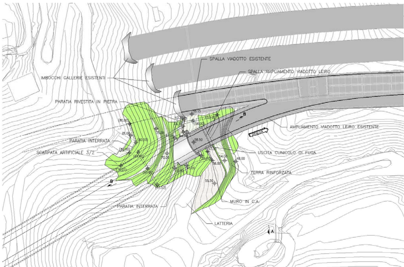
Fig. 3.6.2 – La sistemazione finale dell'area d'intervento (cfr. AUA0131-2)
