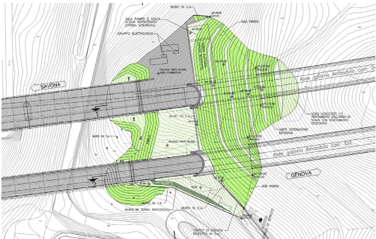
Fig. 3.7.1 – Planimetria d'imbocco galleria Amandola lato Savona (cfr. AUA0136-2)
