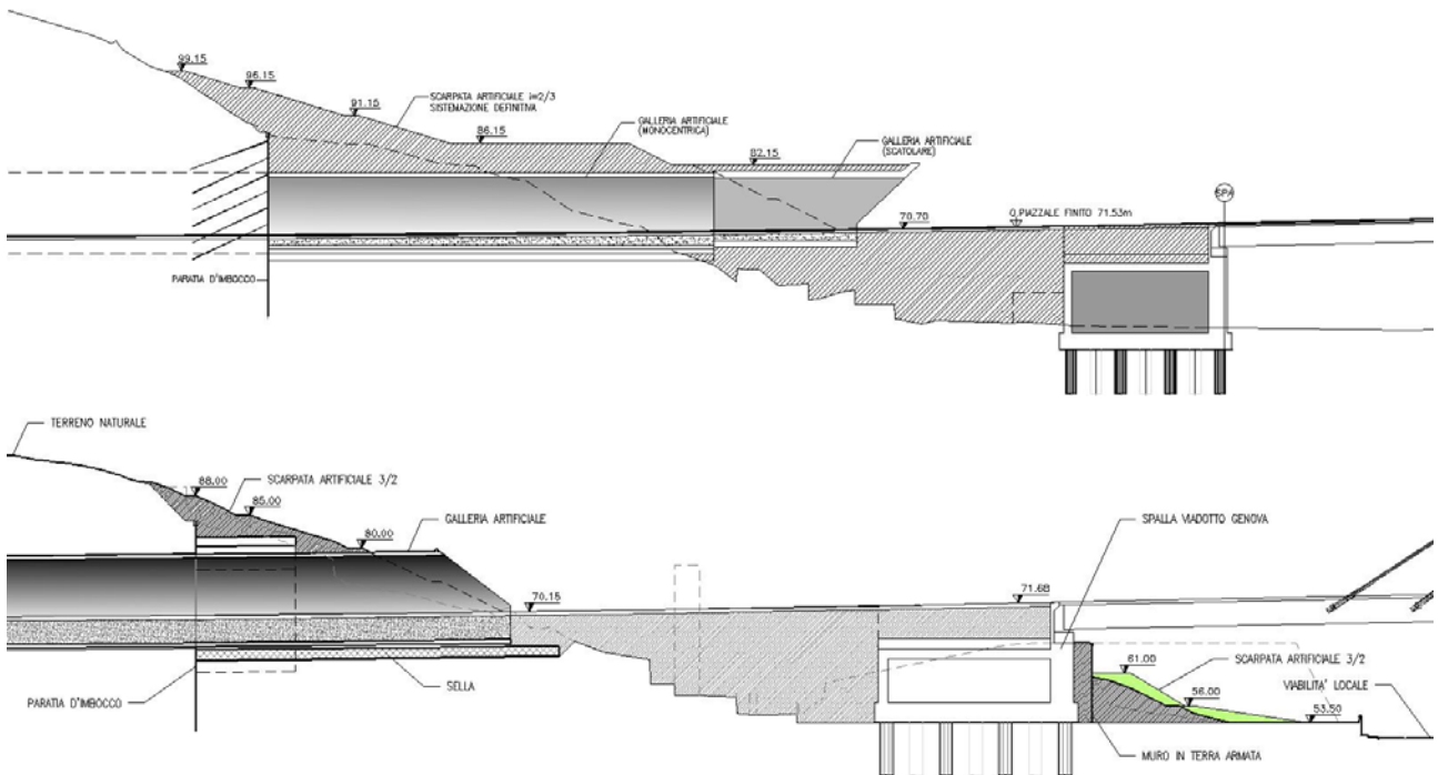
Figura 4 – Profilo longitudinale sulla carreggiata est dell’imbocco Monterosso lato Genova: in alto il progetto definitivo, in basso quello revisionato
