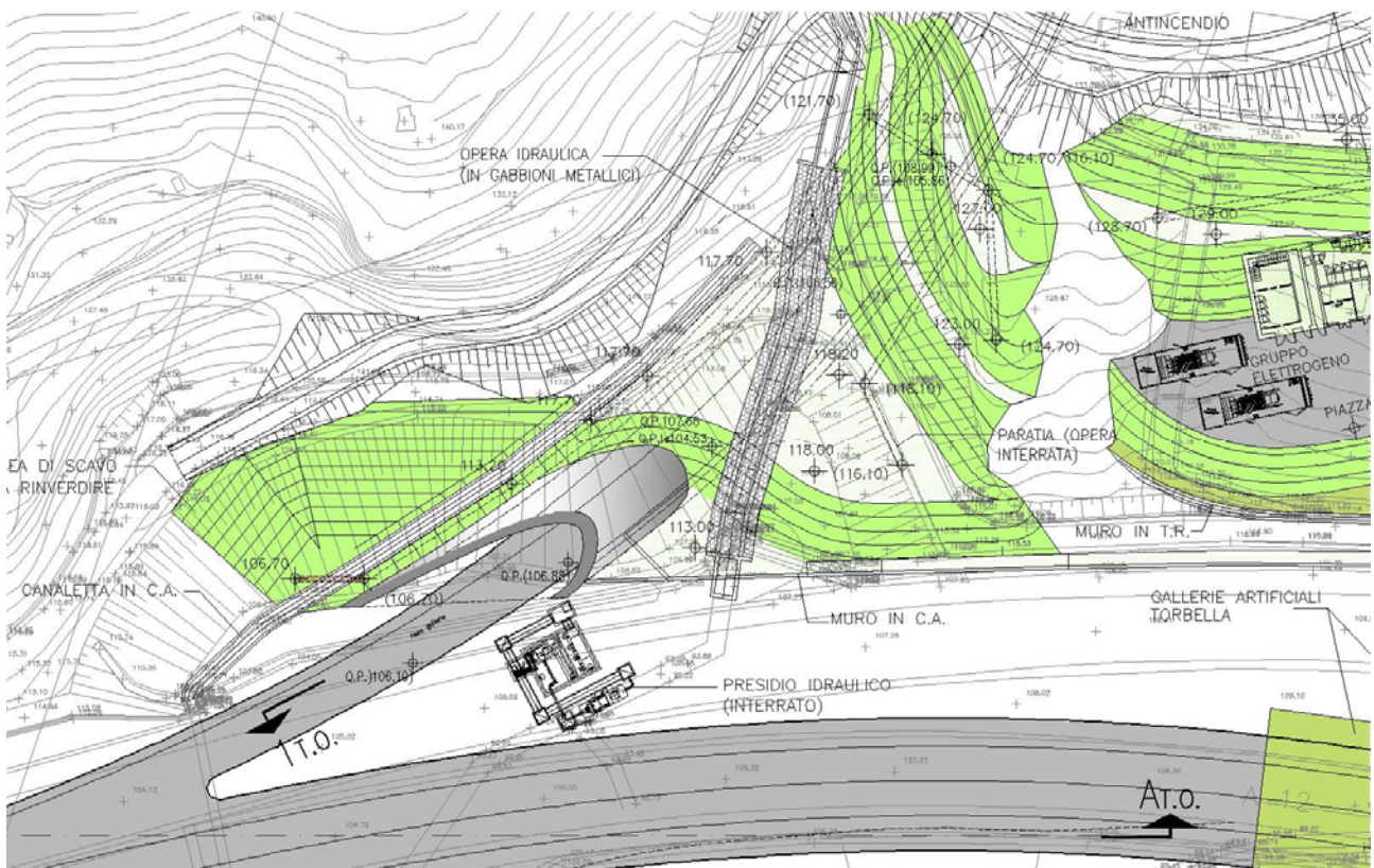
Fig. 6.2.1 – Imbocco galleria Torbella ovest (cfr. AUA0171-2)
