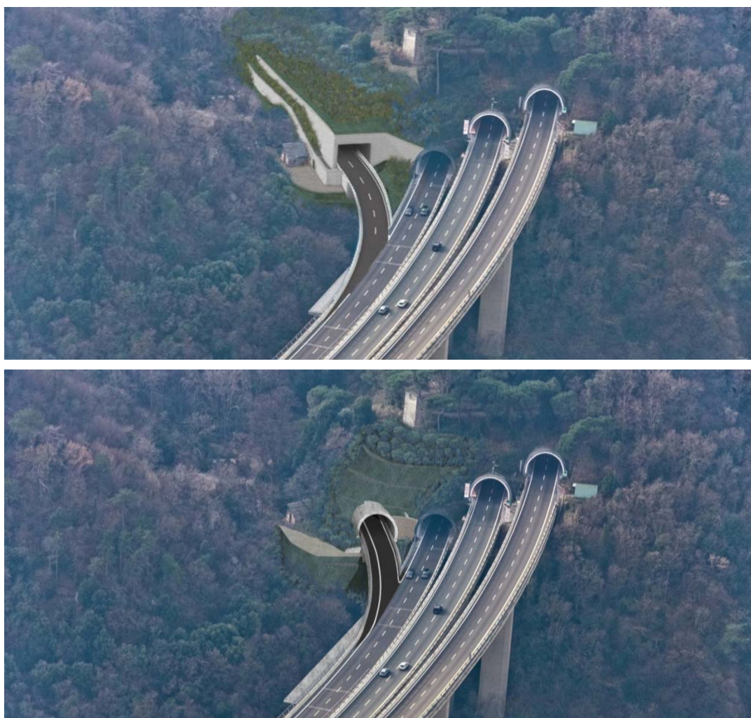
Figura 3 – Fotoinserimento dell'imbocco Delle Grazie lato sud: in alto il progetto definitivo, in basso quello revisionato
