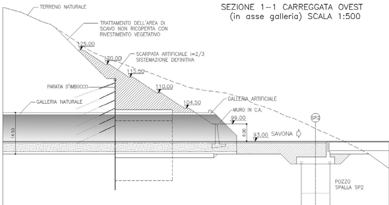
Fig. 3.7.2 – Dettaglio del concio terminale della galleria artificiale (cfr. AUA0136-2)
