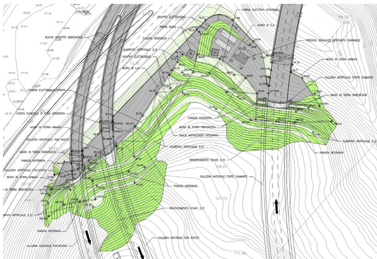
Fig. 5.2.1 – Planimetria dell'area d'imbocco (cfr. AUA0156-1)
