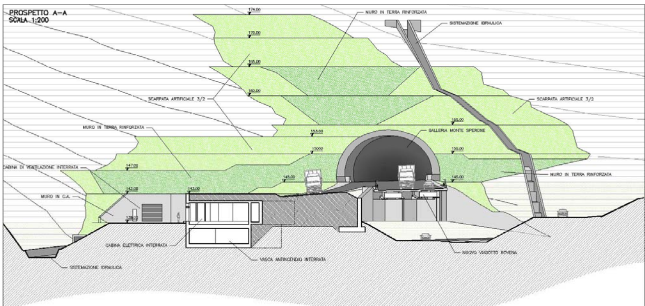
Fig. 7.1.2 – Prospetto dell'imbocco Montesperone lato Livorno con i volumi tecnici sulla sinistra (cfr. AUA0186-1)
