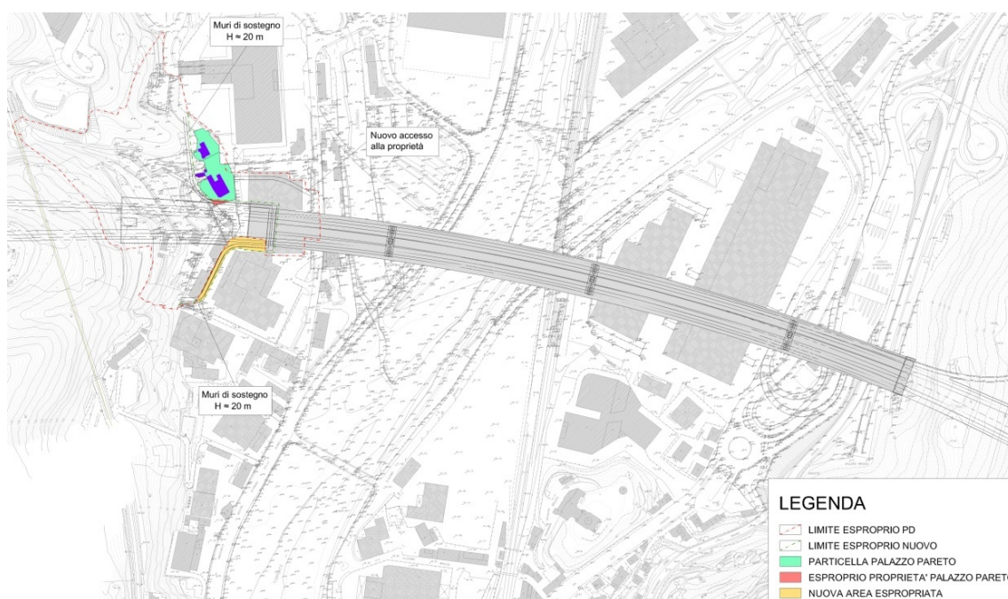
Figura 2 – Stralcio planimetrico variante di tracciato presso Palazzo Pareto
