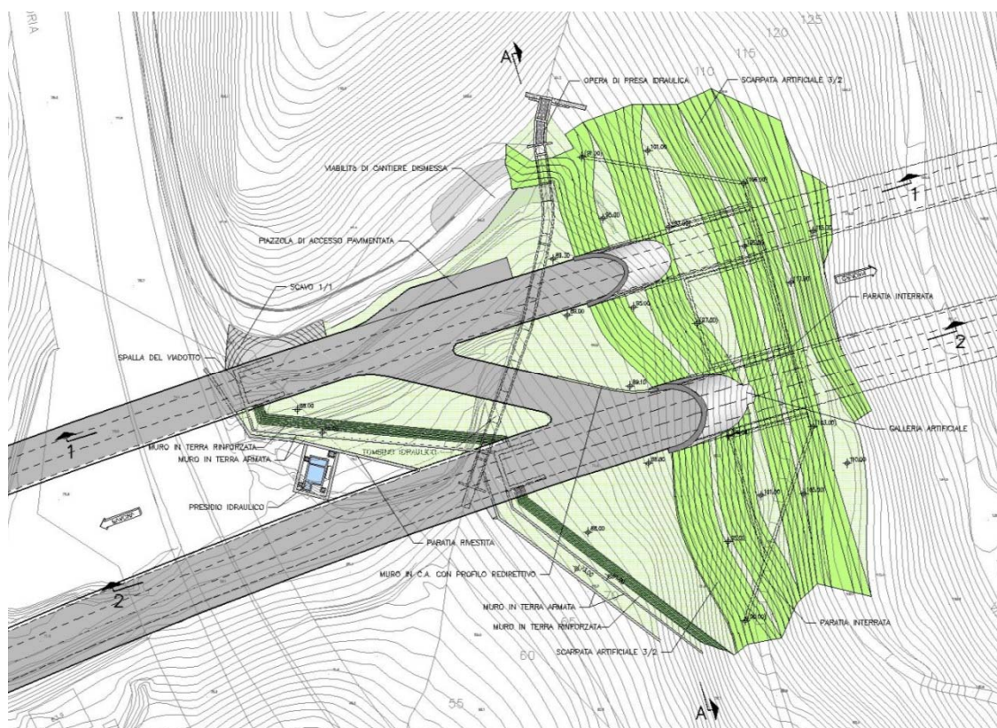
Fig. 3.3.1 – Planimetria della sistemazione finale (cfr. AUA0116-2)
