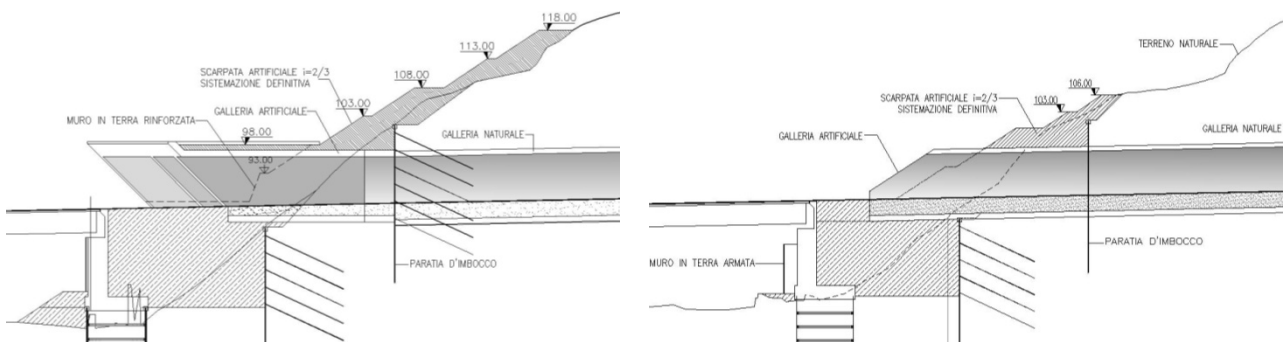
Figura 5 – Profilo longitudinale sulla carreggiata est dell’imbocco Polcevera – Baccan – Bric du vento lato Savona: a sinistra il progetto definitivo, a destra quello revisionato
