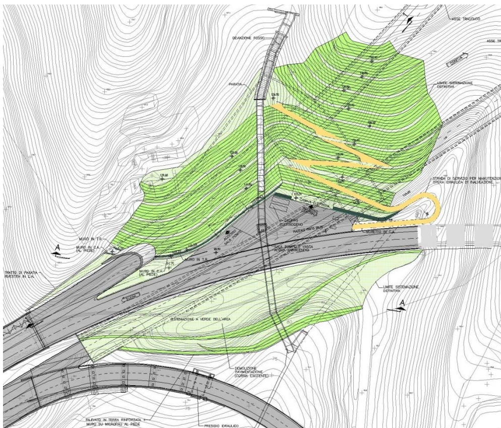
Fig. 2.1.1 – Planimetria della sistemazione definitiva (cfr. AUA0101-2)
