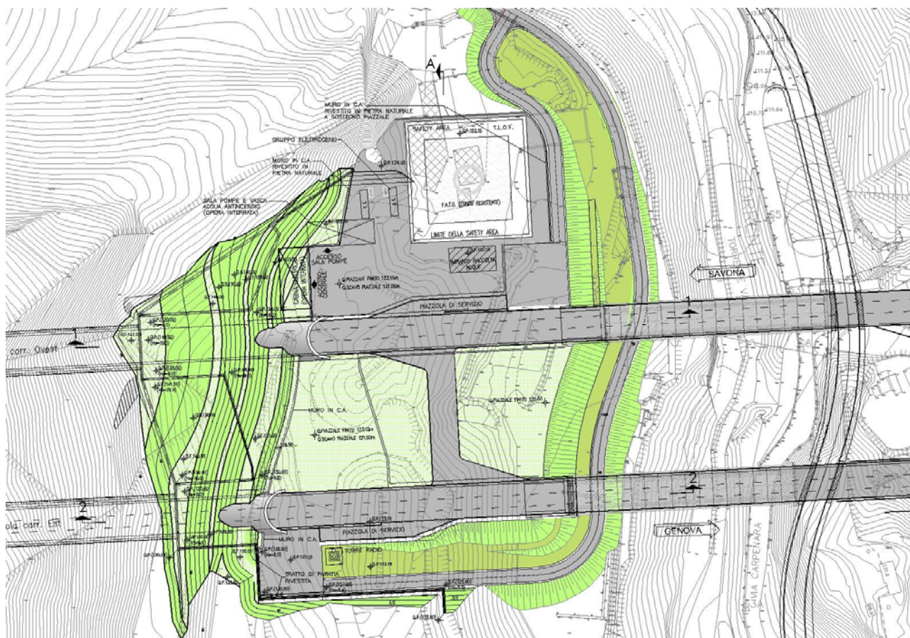
Fig. 4.1.1 – Imbocco galleria Amandola lato Genova (cfr. AUA0141-1)
