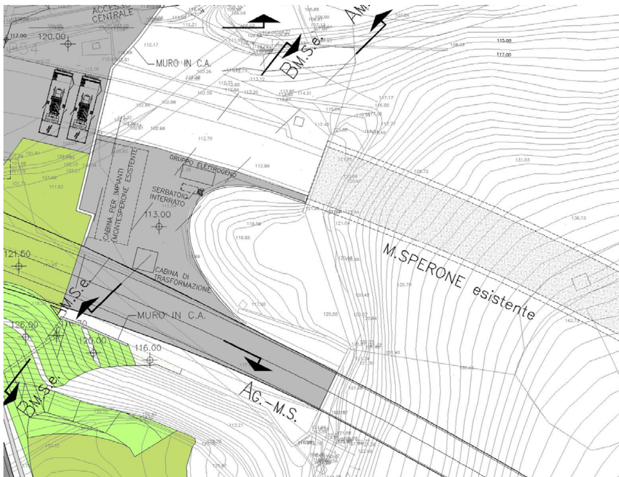
. 6.3.1 –Area imbocco Monte Sperone esistente (cfr. AUA0176-2)
