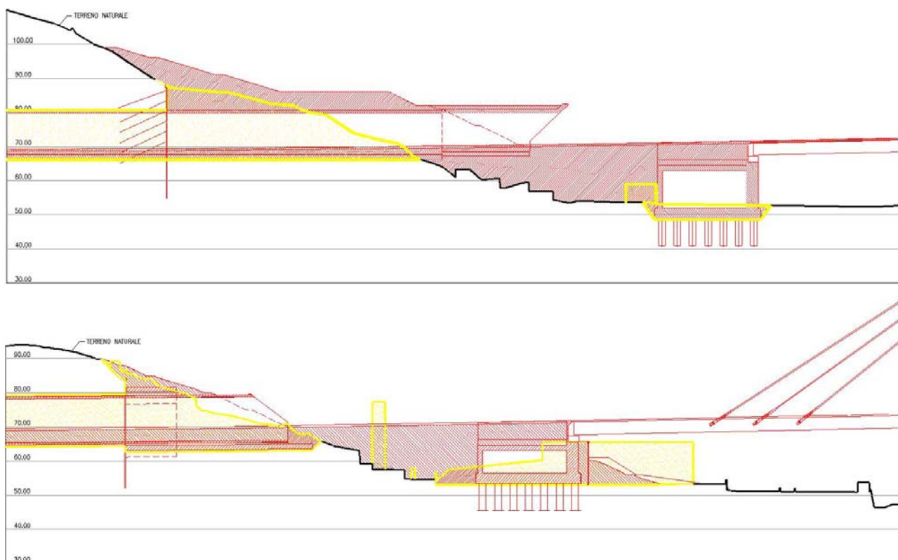
Figura 11 – Sezioni di confronto tra lo stato ante-operam e quello di progetto- Monterosso lato Genova: in alto il progetto definitivo, in basso quello revisionato
