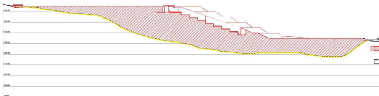
Figura 15 – Sezione di raffronto tra lo stato ante-operam e quello di progetto del deposito presso il cantiere industriale CI06 (Campursone)
