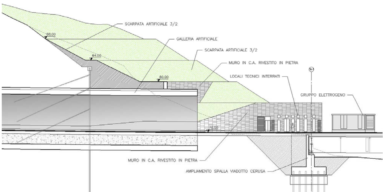
Fig. 3.2.1 – Sezione sulla galleria artificiale (cfr. AUA0111-1)
