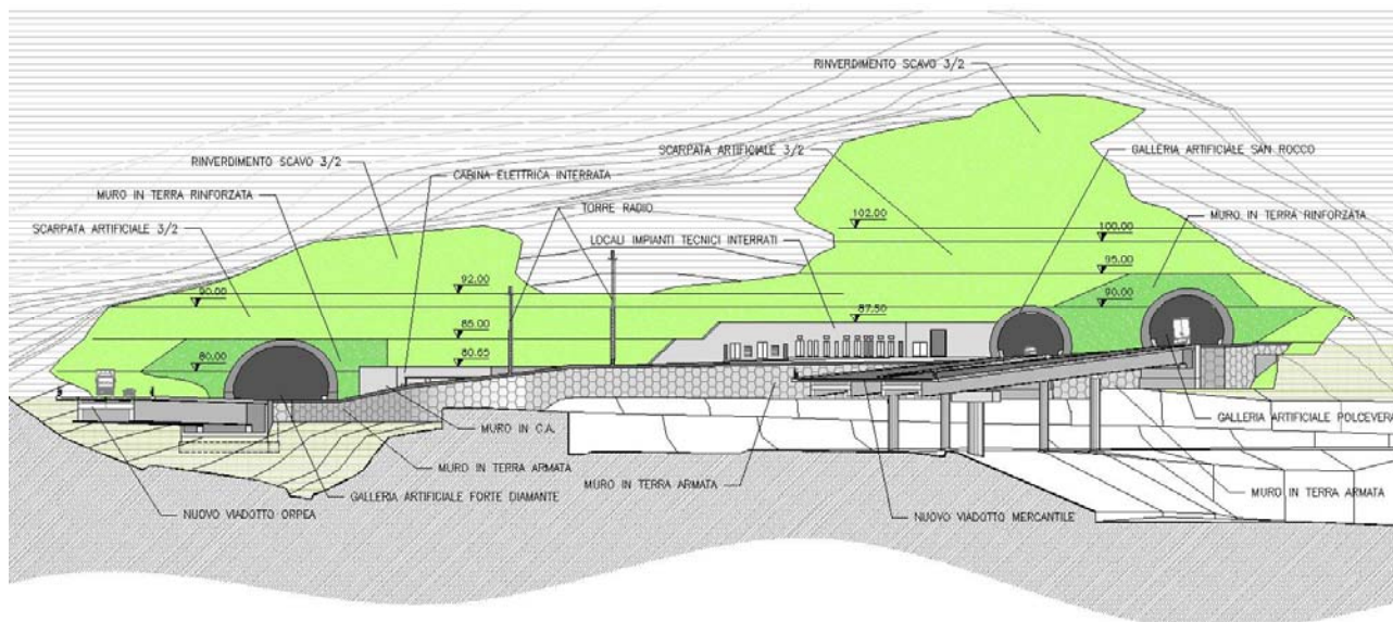
Fig. 5.2.2 – Il fronte della sistemazione definitiva con i viadotti Mercantile e Orpea (cfr. AUA0156-1)
