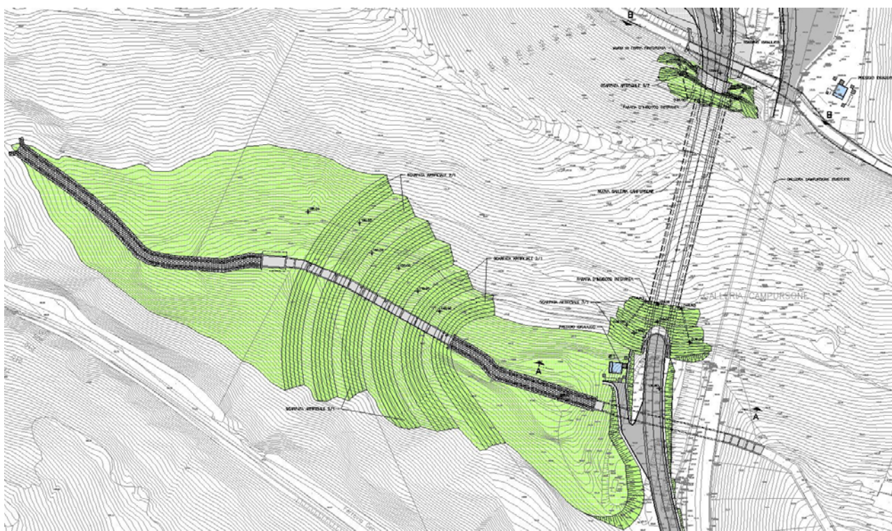
Fig. 7.4.2 – Sistemazione definitiva degli imbocchi Campursone nord e sud e del riempimento della valle del rio Briscata (cfr. AUA0201-2 e AUA0206-2)
