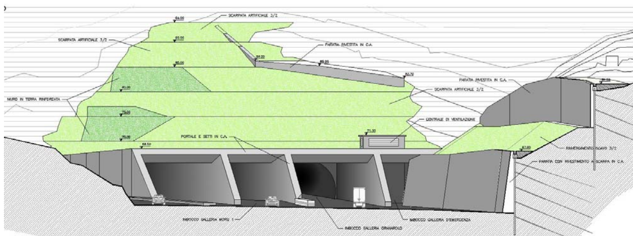
Fig. 7.2.1 – Il sistema strutturale contenente i nuovi imbocchi a nord della barriera (cfr. AUA0191-1)
