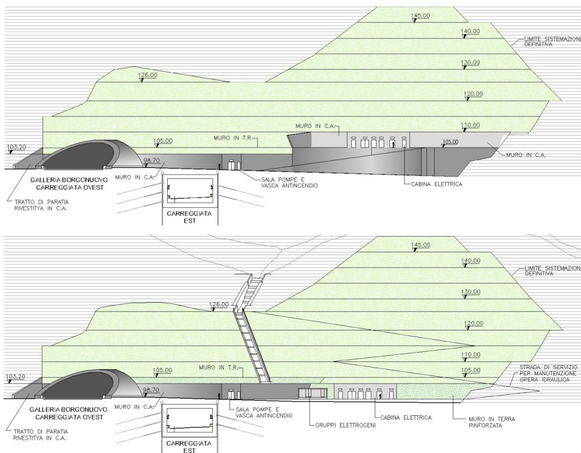
Figura 10 – Prospetto dell’area di imbocco della galleria Borgonuovo lato Savona: in alto il progetto definitivo, in basso quello revisionato
