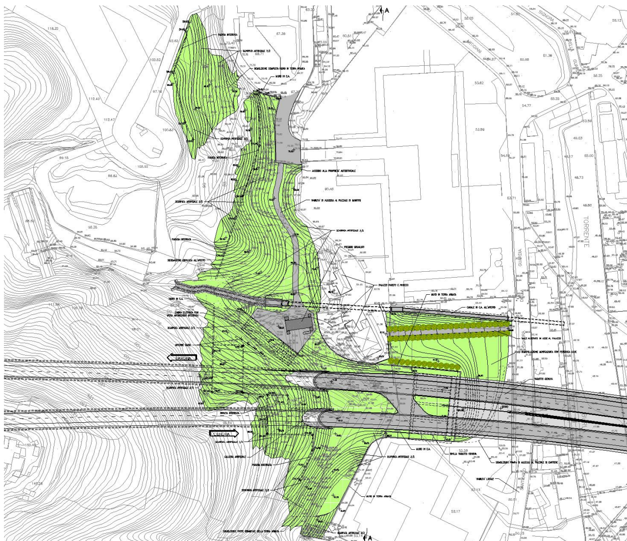
Fig. 5.1.2 – Planimetria dell'area di imbocco (cfr. AUA0151-2)
