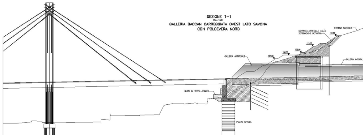
Fig. 5.3.1 – Il profilo inclinato della galleria artificiale (cfr. AUA0166-2)
