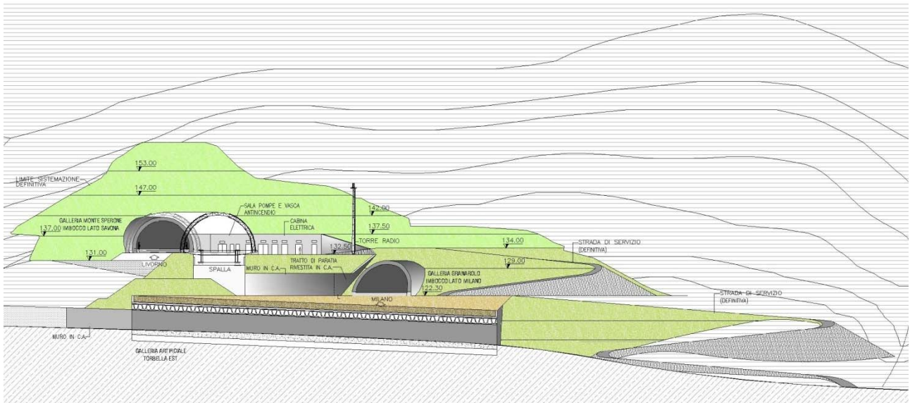
Fig. 6.4.2 – Prospetto degli imbocchi nell'area Torbella sud (cfr. AUA0181-2)
