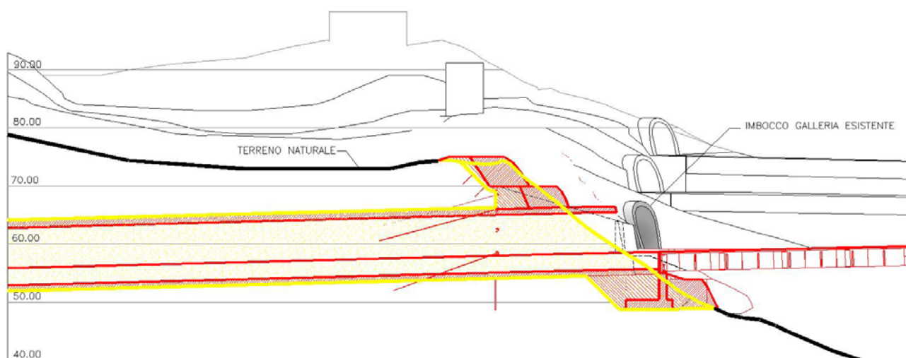
Figura 14 – Sezione di raffronto tra lo stato ante-operam e quello di progetto dell'imbocco Delle Grazie lato sud
