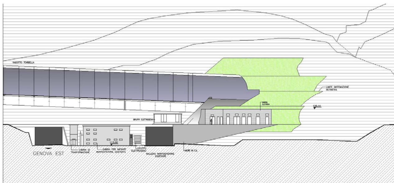
Fig. 6.3.2 – Imbocco galleria Monte Sperone esistente a sinistra (cfr. AUA0176-2), a destra, su livello superiore, gli imbocchi delle gallerie Forte Diamante (cfr. AUA0161-2) e Bric Du Vent (cfr. AUA0161-2)
