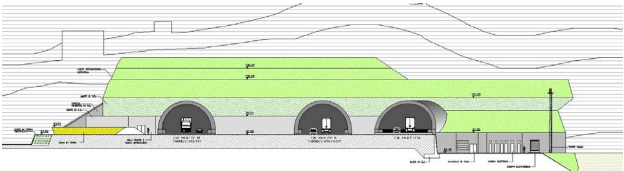
Fig. 3.4.2 – Prospetto dei tre imbocchi e del piazzale a quota inferiore (cfr. AUA0121-2)
