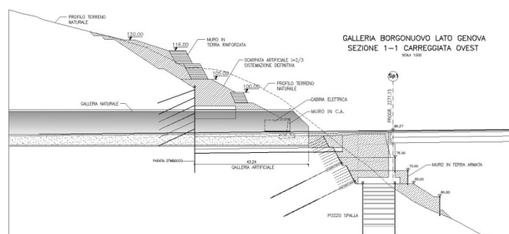
Fig. 3.1.2 – Profilo lungo la carreggiata ovest (cfr. AUA0106-2)
