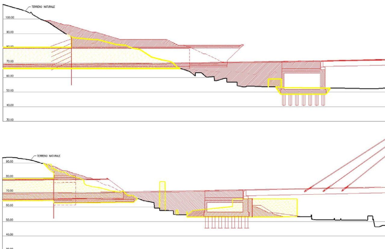
Fig. 1.1.4 – Sezioni di confronto tra lo stato ante-operam e quello di progetto lungo l'asse della carreggiata est: in alto il progetto definitivo, in basso quello revisionato
