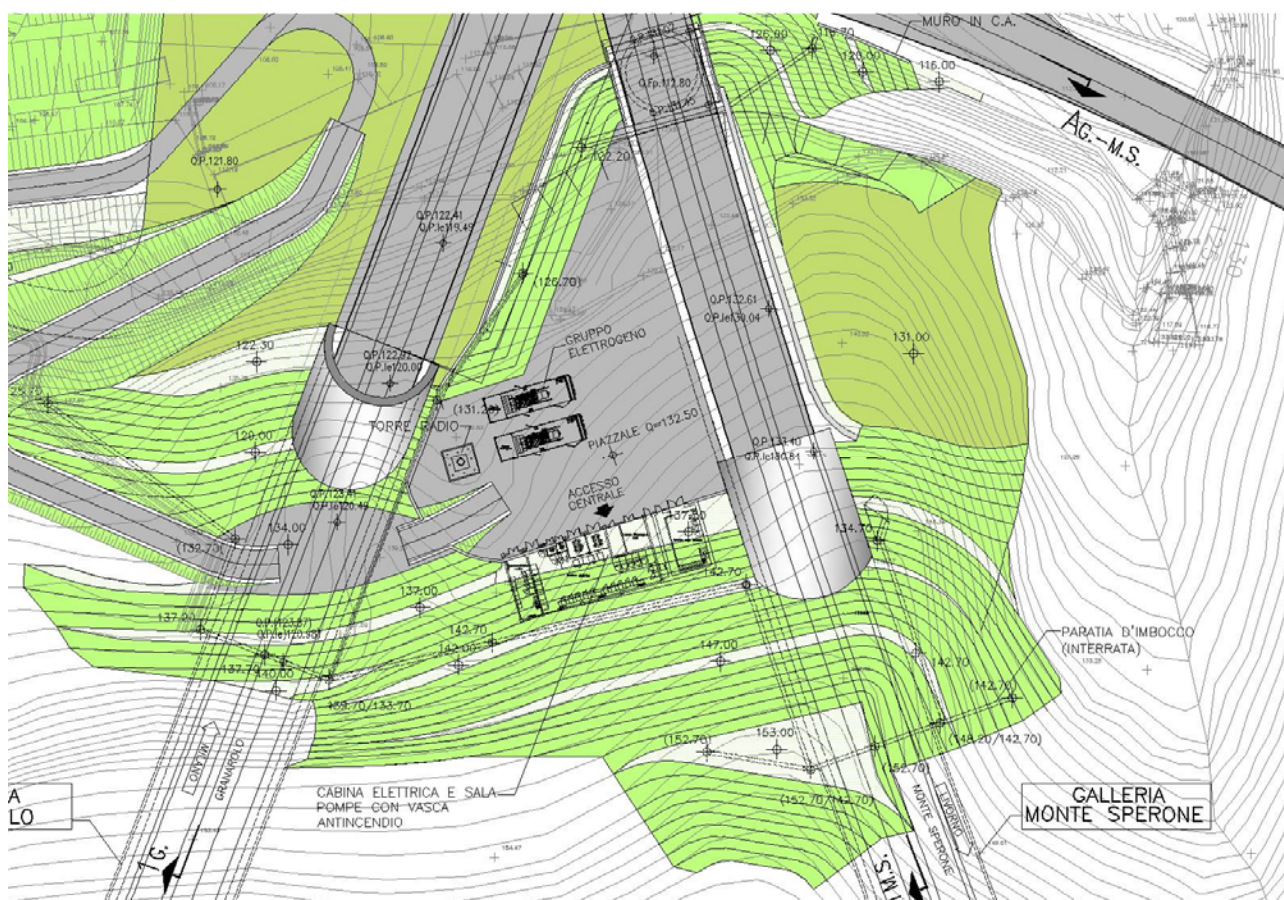
Fig. 6.4.1 – Imbocco galleria Monte Sperone (cfr. AUA0181-2)
