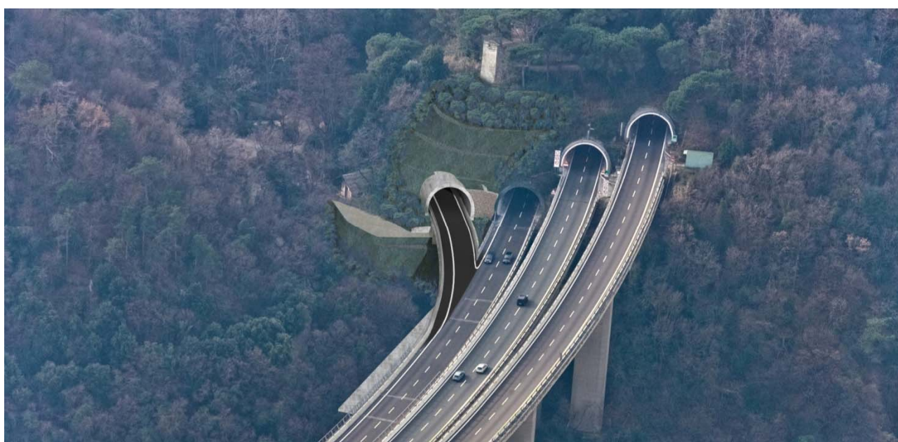
Fig. 1.1.2 – Fotoinserimento dell'imbocco Delle Grazie lato sud: in alto il progetto definitivo, in basso quello revisionato
