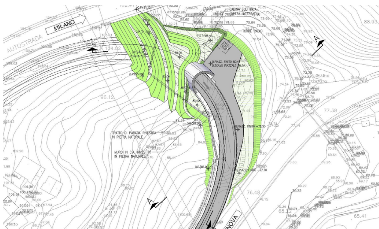
Fig. 5.4.1 – Imbocco galleria Morego lato est (cfr. AUA0211-1)
