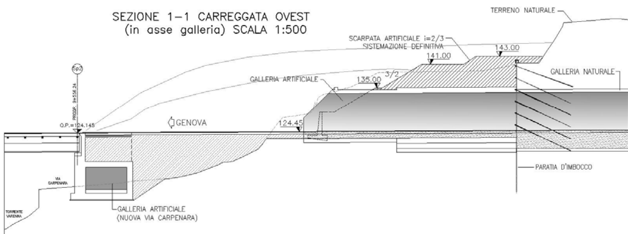
Fig. 4.2.1 – Sezione longitudinale in asse galleria (cfr. AUA0146-1)
