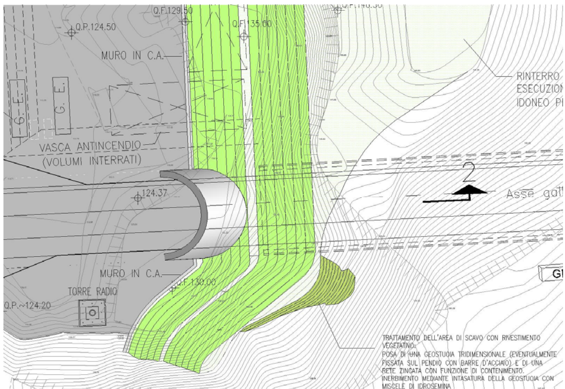
Fig. 4.2.2 – Dettaglio planimetrico imbocco carreggiata est (cfr. AUA0146-1)
