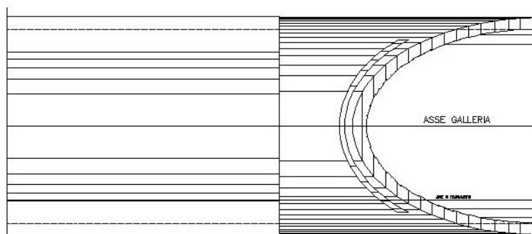
Fig. 1.3 – Concio terminale galleria artificiale a "becco di flauto"
