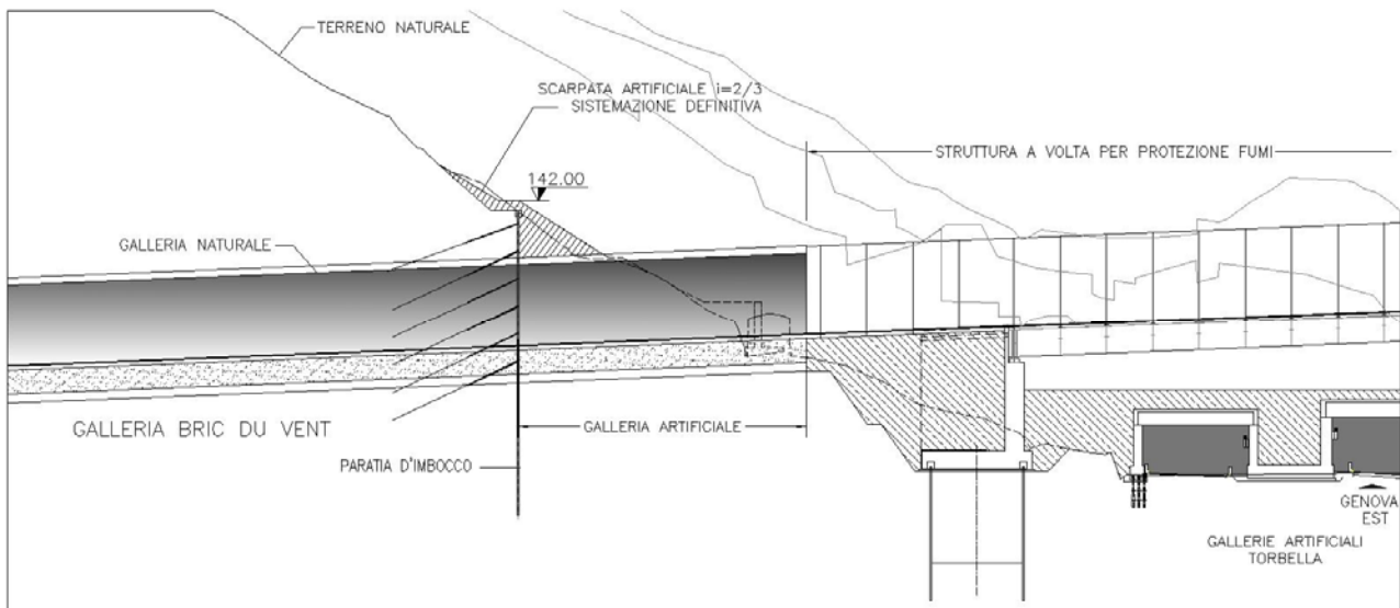
Fig. 6.1.2 – Profilo longitudinale della galleria Bric du Vento lato Livorno (cfr. AUA0161-2)
