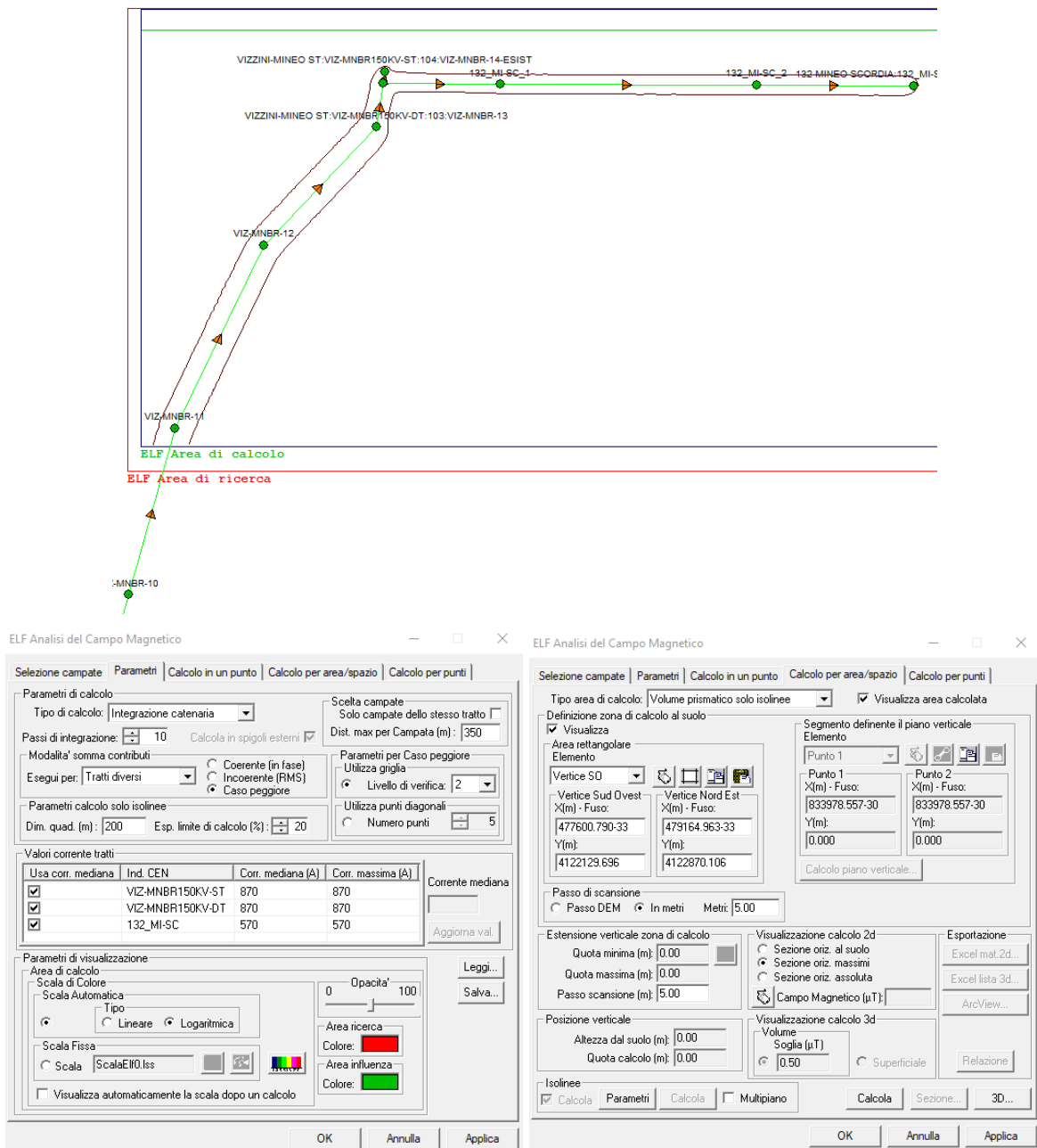
Figura 2 – Schema del modello impostato per le valutazioni CEM sul sistema WinEDT
