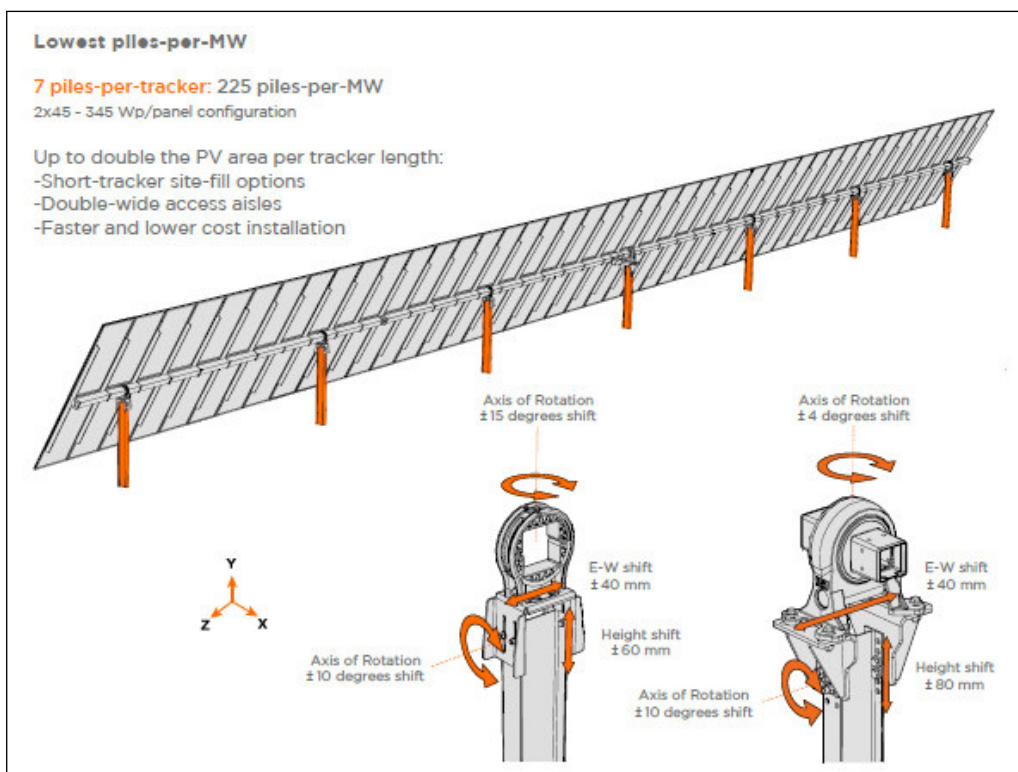
Figura 5 – schema tipo funzionamento inseguitore monoassiale
