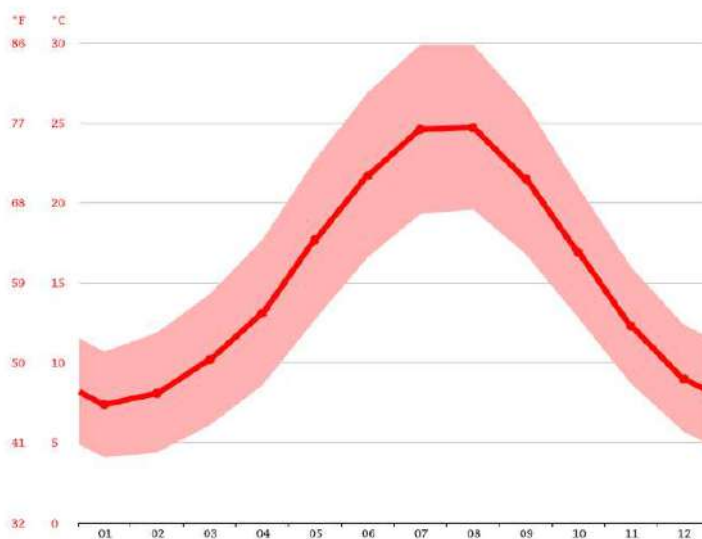
Illustrazione 3.9: Grafico temperatura di San Severo.
