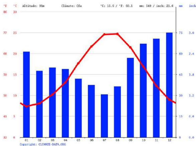
Illustrazione 3.8: Grafico del clima di San Severo (
