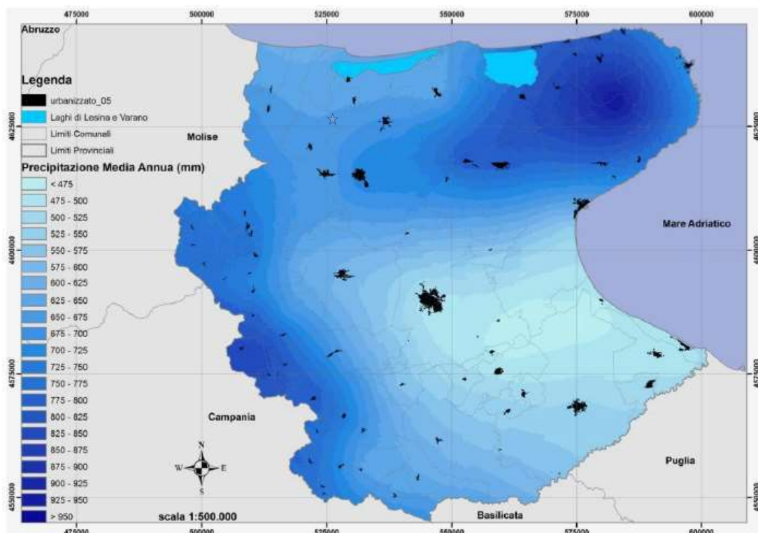
Illustrazione 3.3: Isoiete annue
