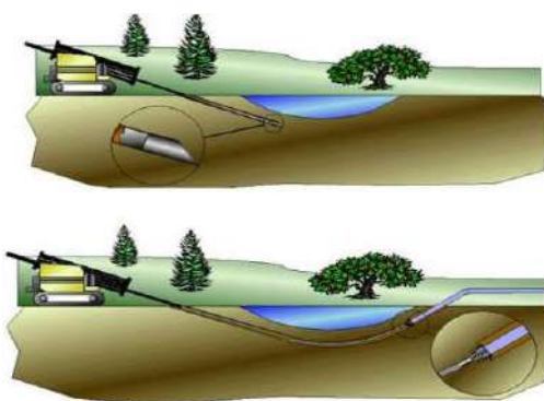
Illustrazione 2.1: Tecnica del "no dig" o "perforazione teleguidata" che sarà utilizzata per l'attraversamento dei corsi d'acqua.
