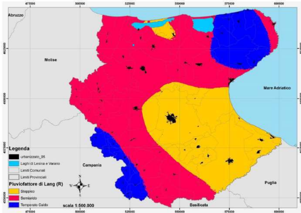
Illustrazione 3.4: Pluviofatto di Lang
