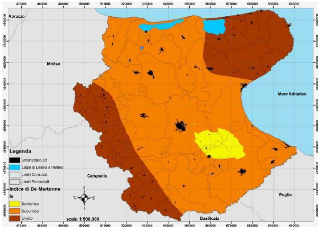
Illustrazione 3.6: Indice di Martonne
