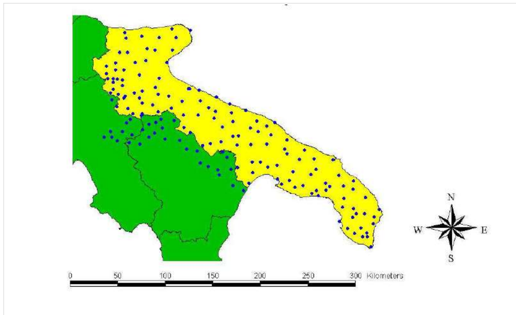
Illustrazione 3.1: Le stazioni termopluviometriche della Puglia.
