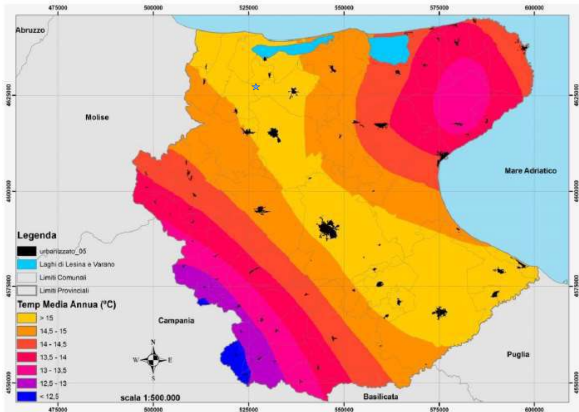
Illustrazione 3.2: Isotherme medie annue
