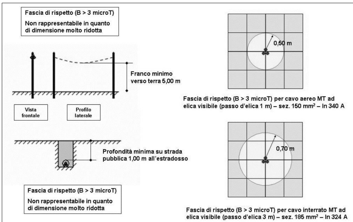
Figura 8: DPA linee MT ad elica visibile
