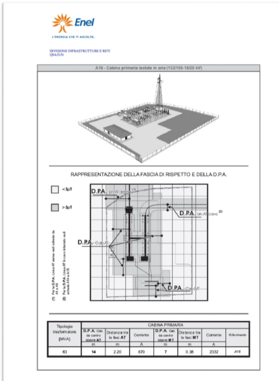
Figura 12: DPA Cabina Primaria AT/MT Enel equipaggiata con n° 2 trasformatori AT/MT da 63 MVA- Linea Guida per l'applicazione del § 5.1.3 dell'Allegato al D.M. 29.05.08 – Distanza di prima approssimazione da linee e cabine elettriche
