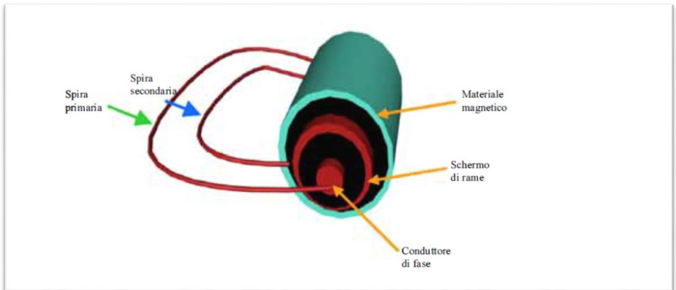
Figura 26: schema tridimensionale del cavo a debole emissione di campo magnetico- tecnica "Solid-bonding"
