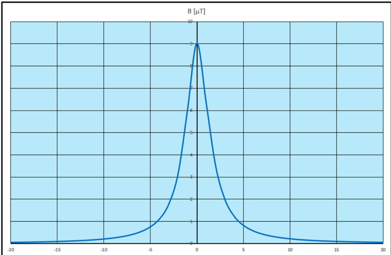
Figura 9: Induzione magnetica generata durante l'esercizio dalle dorsali MT valutata ai sensi della Norma CEI 211-4 – Guida ai metodi di calcolo dei campi elettrici e magnetici generati da linee elettriche
