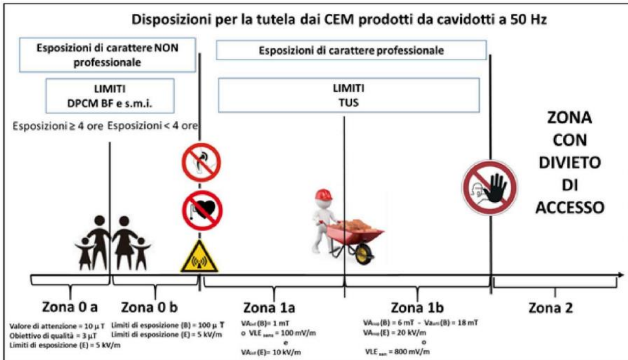
Figura 11: Misure di prevenzione e protezione per la tutela dai CEM prodotti da cavidotti a 50 Hz
