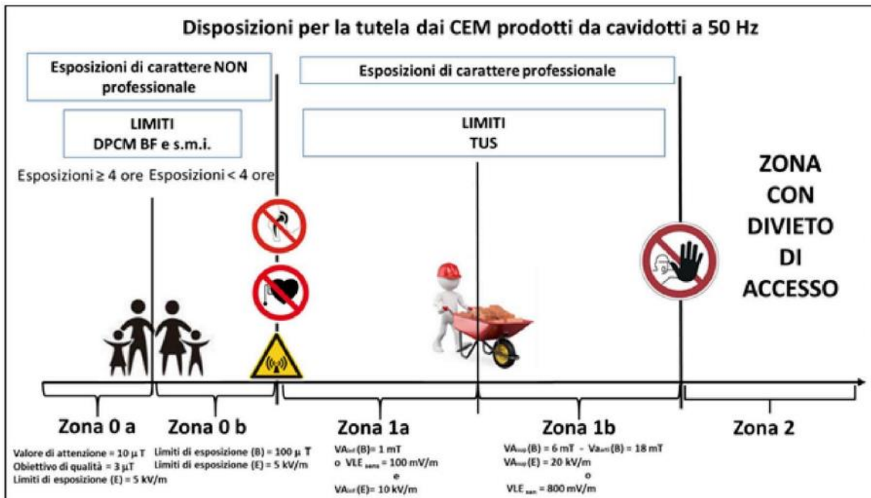
Figura 18: Misure di prevenzione e protezione per la tutela dai CEM prodotti da cavidotti a 50 Hz
