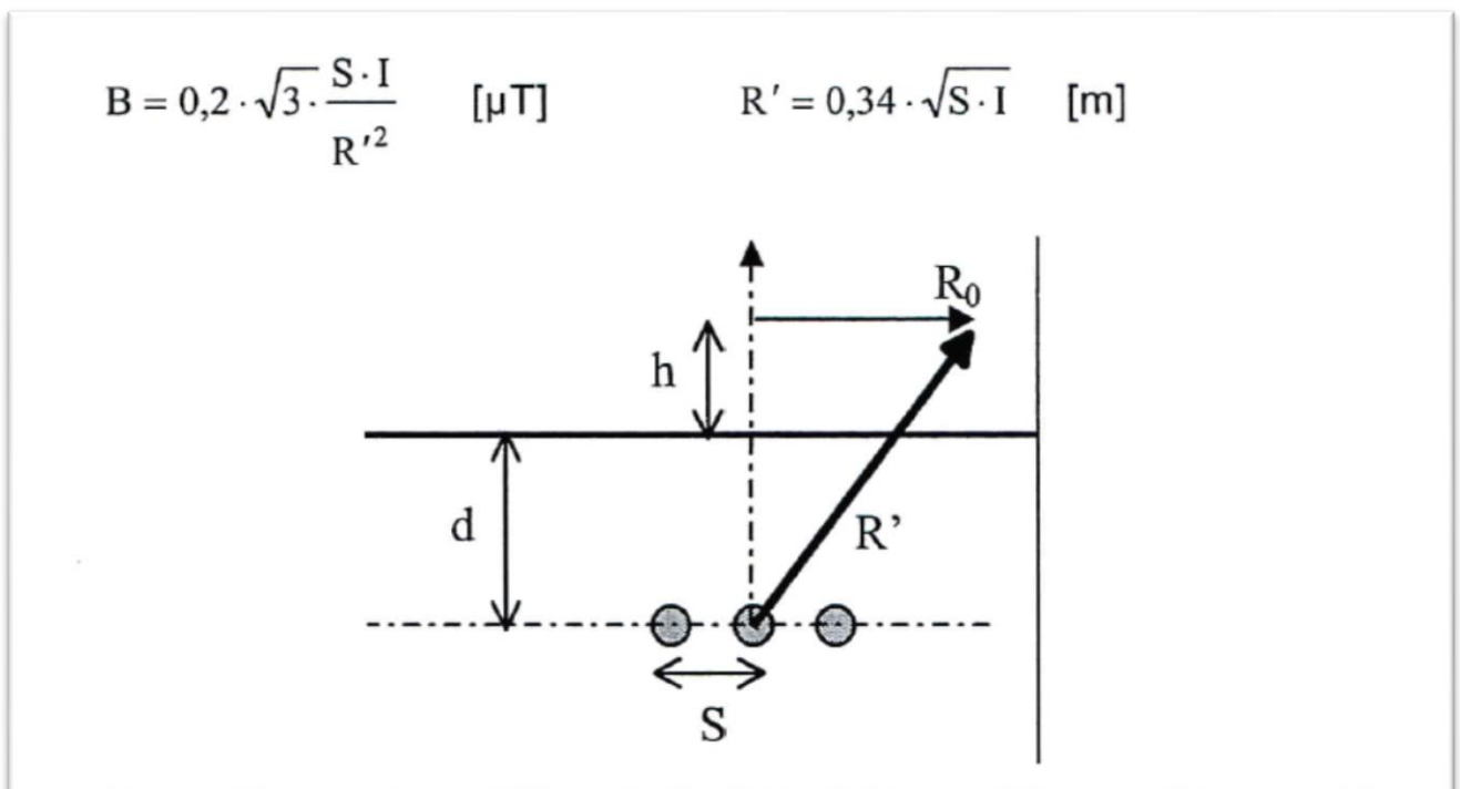
Figura 13: Schema di principio per il calcolo delle distanze da terne di cavi interrati con posa in piano/sbarre AT isolate in aria oltre le quali l'induzione magnetica è inferiore all'obiettivo di qualità – Norma CEI 106-11 – Guida per la determinazione delle fasce di rispetto per gli elettrodotti secondo le disposizioni del DPCM 8 luglio 2003
