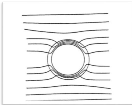
Figura 22: andamento qualitativo della deformazione delle linee di forza di un campo magnetico uniforme per effetto di un nucleo in materiale ferromagnetico
