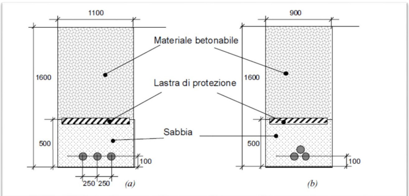
Figura 23: schermatura cavi elettrici interrati
