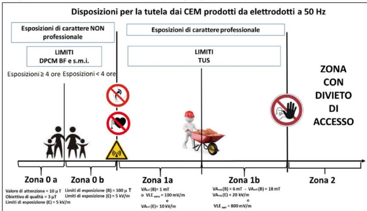
Figura 15: Misure di prevenzione e protezione per la tutela dai CEM prodotti da Elettrodotti a 50 Hz
