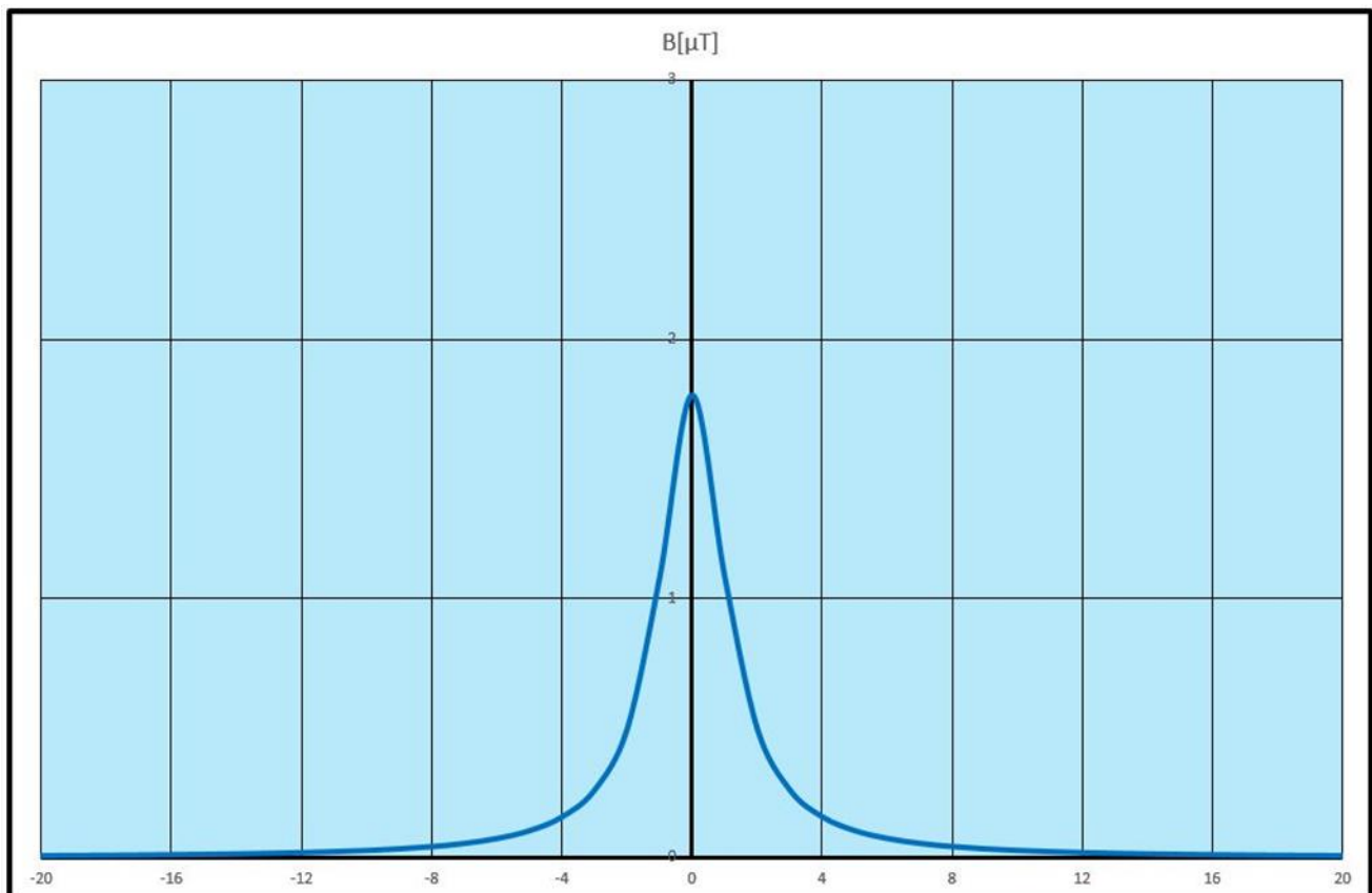
Figura 10: Induzione magnetica generata durante l'esercizio dalle linee MT di campo valutata ai sensi della Norma CEI 211-4 – Guida ai metodi di calcolo dei campi elettrici e magnetici generati da linee elettriche
