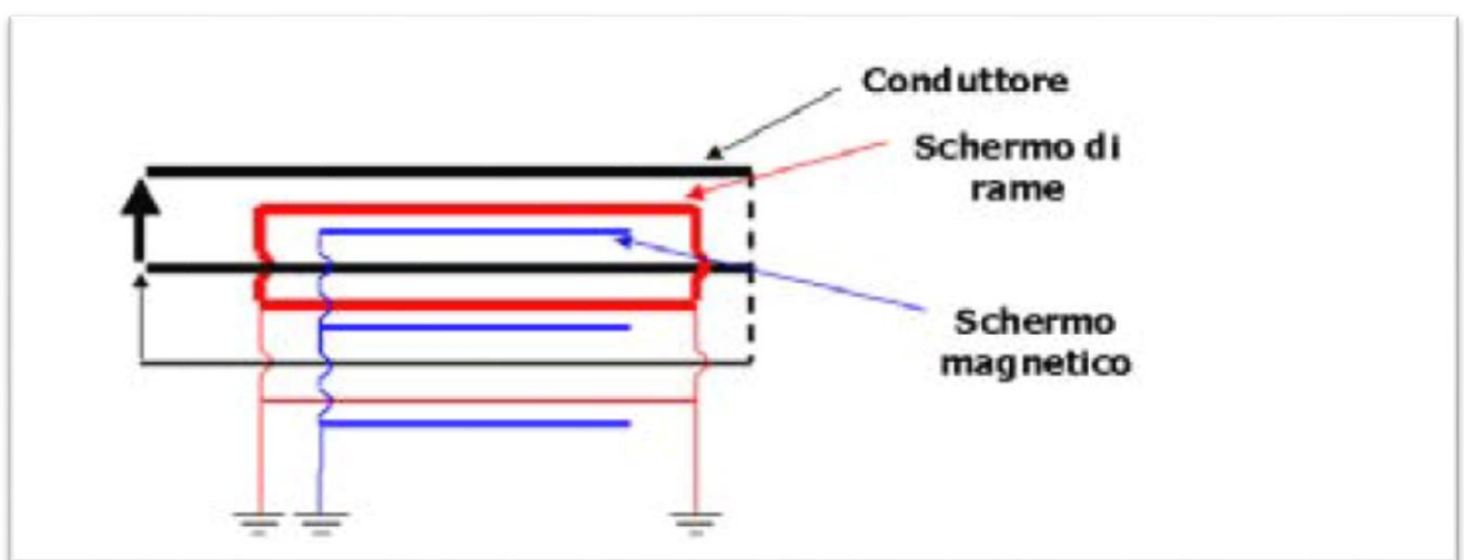
Figura 25: schema bidimensionale del cavo unipolare e della messa a terra degli schermi- tecnica "solid bonding"
