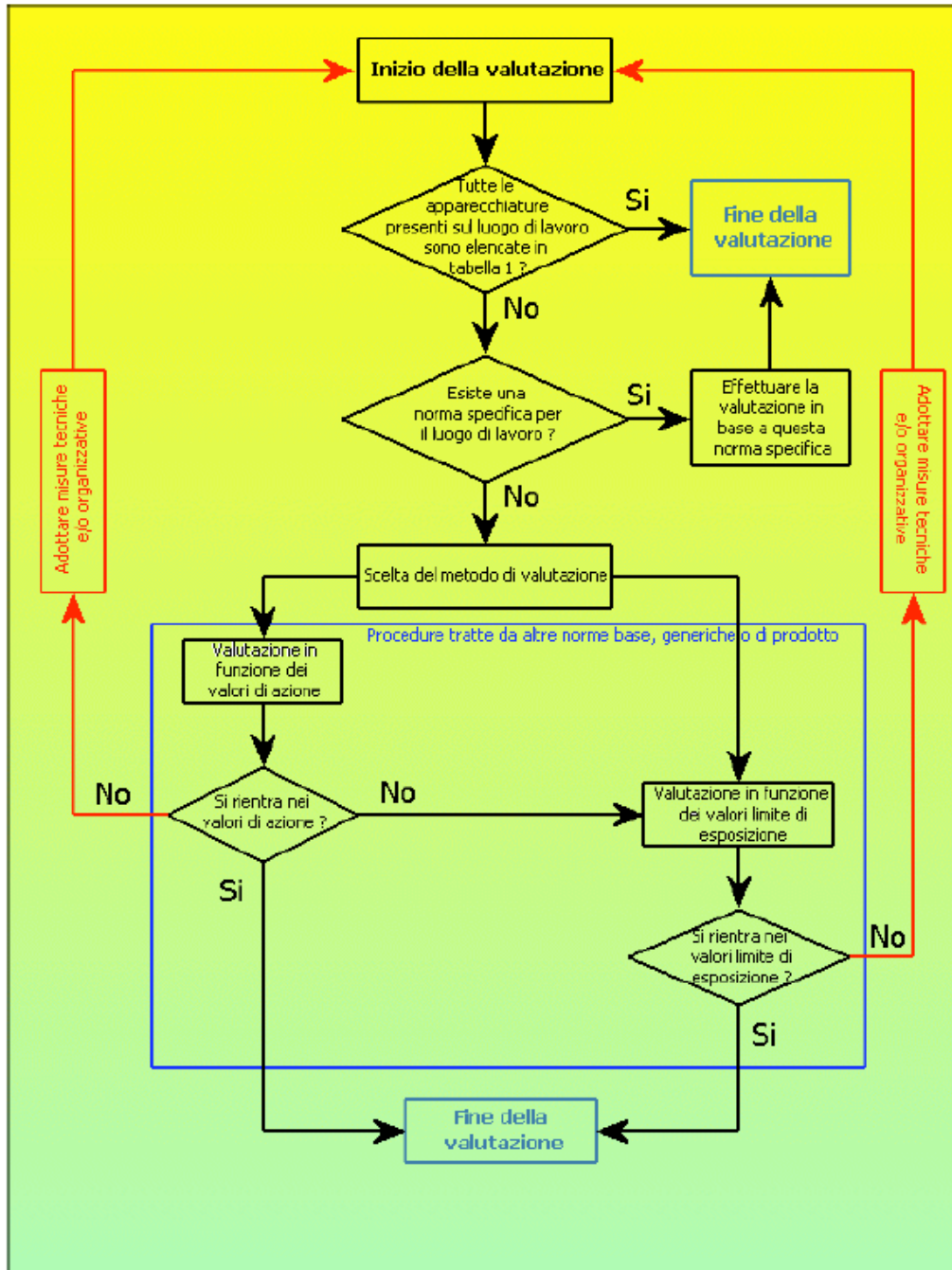
Figura 19: Diagramma di flusso del processo di valutazione del rischio elettromagnetico (CEI EN 50499)
