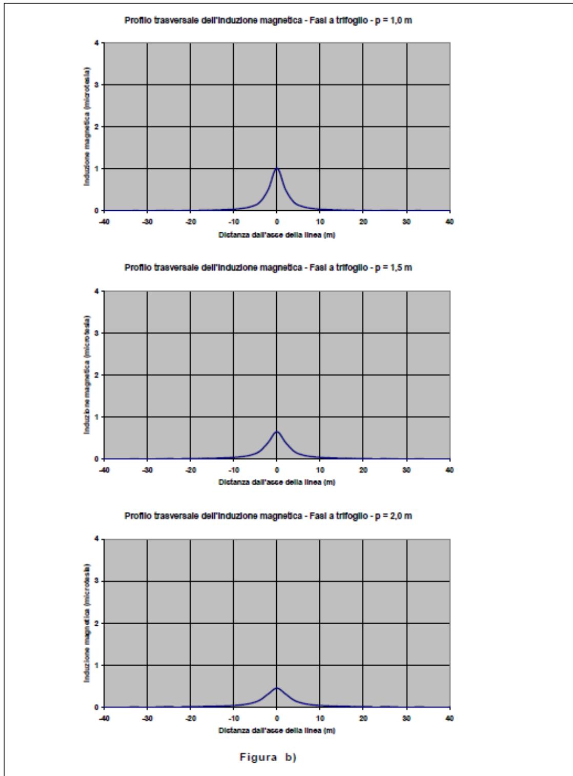
Figura 6: figura b) tratta dalla Norma CEI 11-17
