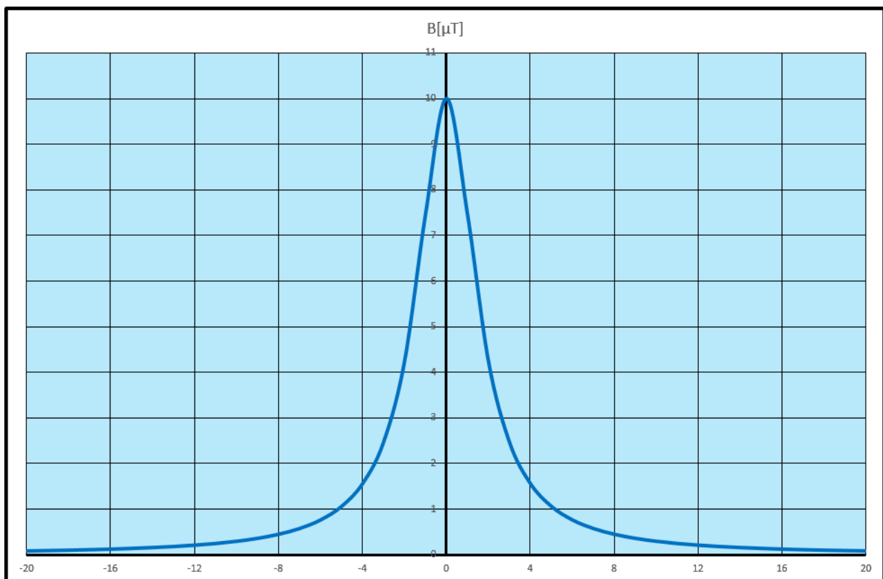
Figura 17: induzione magnetica generata durante l'esercizio dalla linea valutata applicando la procedura delle Norma CEI 211-4 – Guida ai metodi di calcolo dei campi elettrici e magnetici generati da linee elettriche
