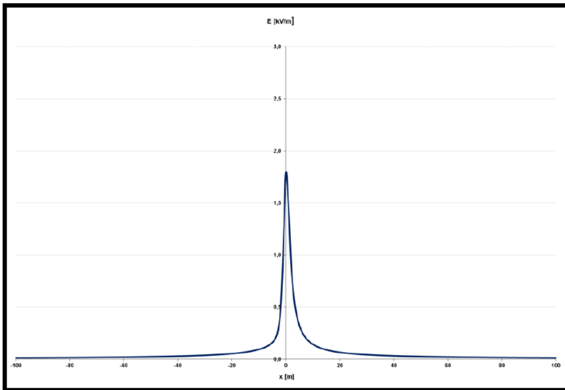
Figura 16: Campo elettrico generato dalla Linea durante l'esercizio valutato applicando la procedura della Norma CEI 211-4 - Guida ai metodi di calcolo dei campi elettrici e magnetici generati da linee elettriche
