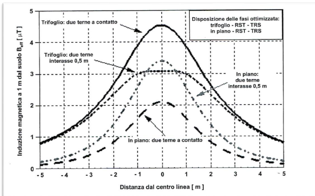
Figura 7: Confronto tra i profili laterali dell'induzione magnetica a 1 m da terra di due terne poste rispettivamente a trifoglio e in piano a contatto, I=1000 ; profondità di posa= 1,2 m; diametro cavi 100 mm
