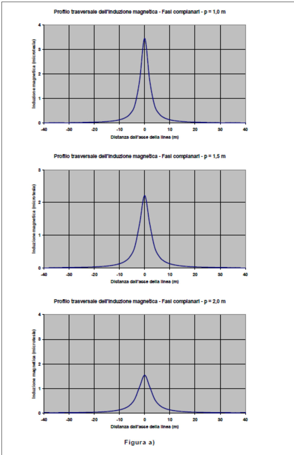
Figura 5: figura a) tratta dalla Norma CEI 11-17
