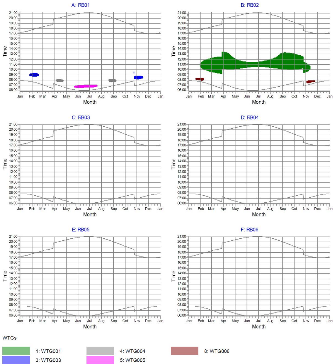
Figura 2 Calendario grafico ombreggiatura dei recettori ottenuto con la simulazione al caso peggiore (non realistica, si veda REL010). Il recettore RB02 subisce ombreggiatura principalmente da WTG001.
