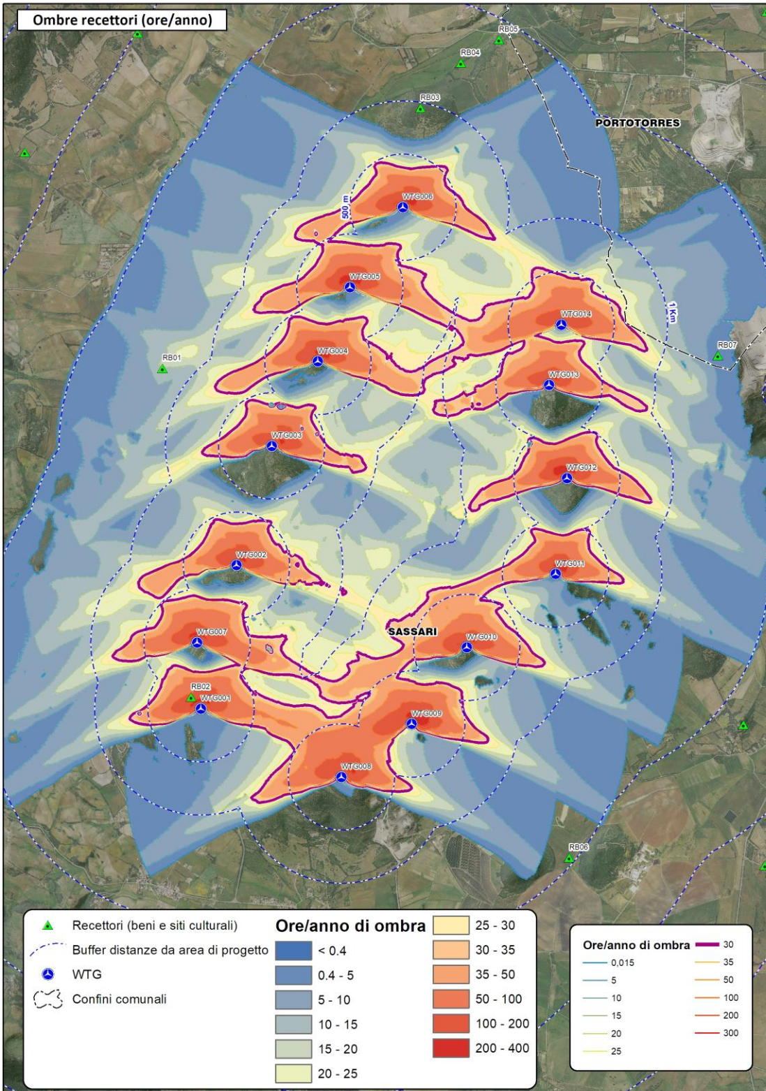
Figura 1 Ombreggiatura (ore di ombra all'anno) subita dai recettori. Solamente il recettore RB02 subisce un ombreggiatura maggiore di 30 ore/anno.
