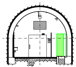
SEZIONE B-B 1:100 COUPE B-B 1:100
