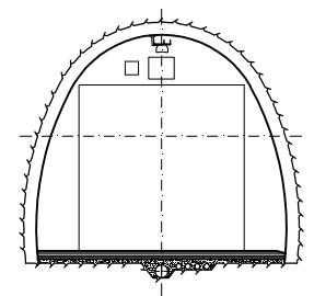
SEZIONE A-A 1:100 COUPE A-A 1:100
