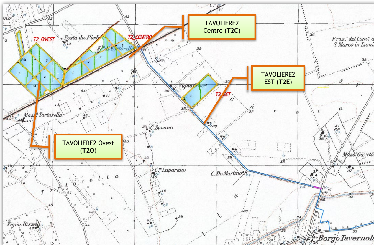
Fig. 3. Layout impianto con identificazione dei Tre Sotto Impianti Ovest, Centro ed EST, e tratto iniziale dell'elettrodoto dorsale (in azzurro) su I.G.M.
