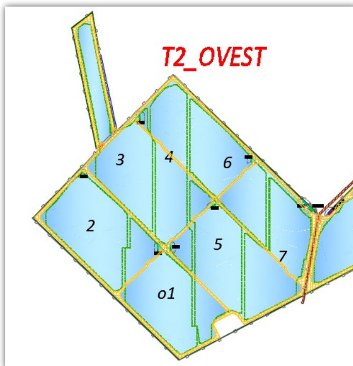
Fig. 4. Layout del Sottoimpianto "TAVOLIERE2 OVEST" con identificazione dei vari subcampi (da 1 a 7).
