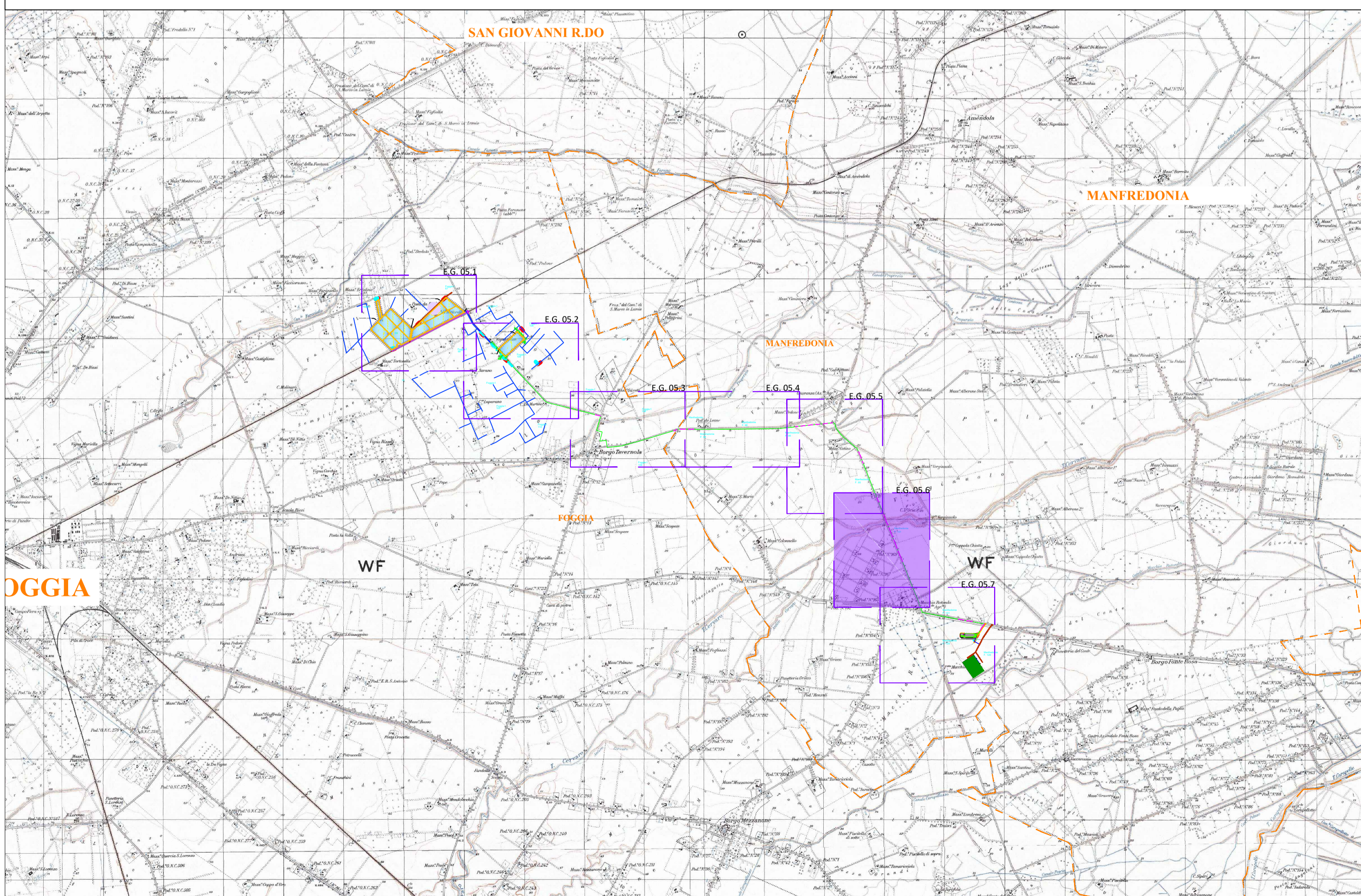
Planimetria chiave su IGM - scala 1:50.000
