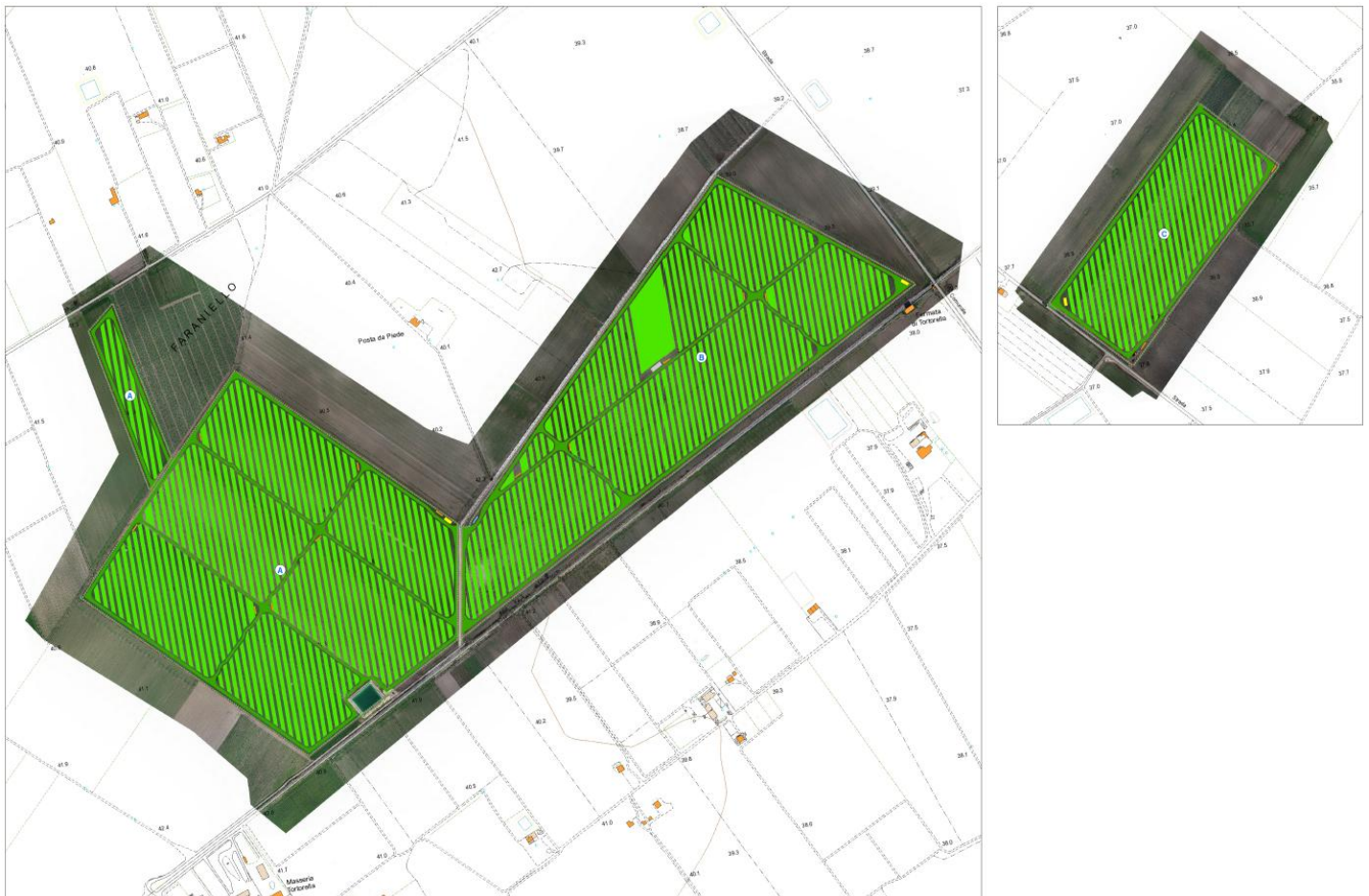
Fig. 4. Schema di irrigazione a zone con sistema di micro-irrigatori.
