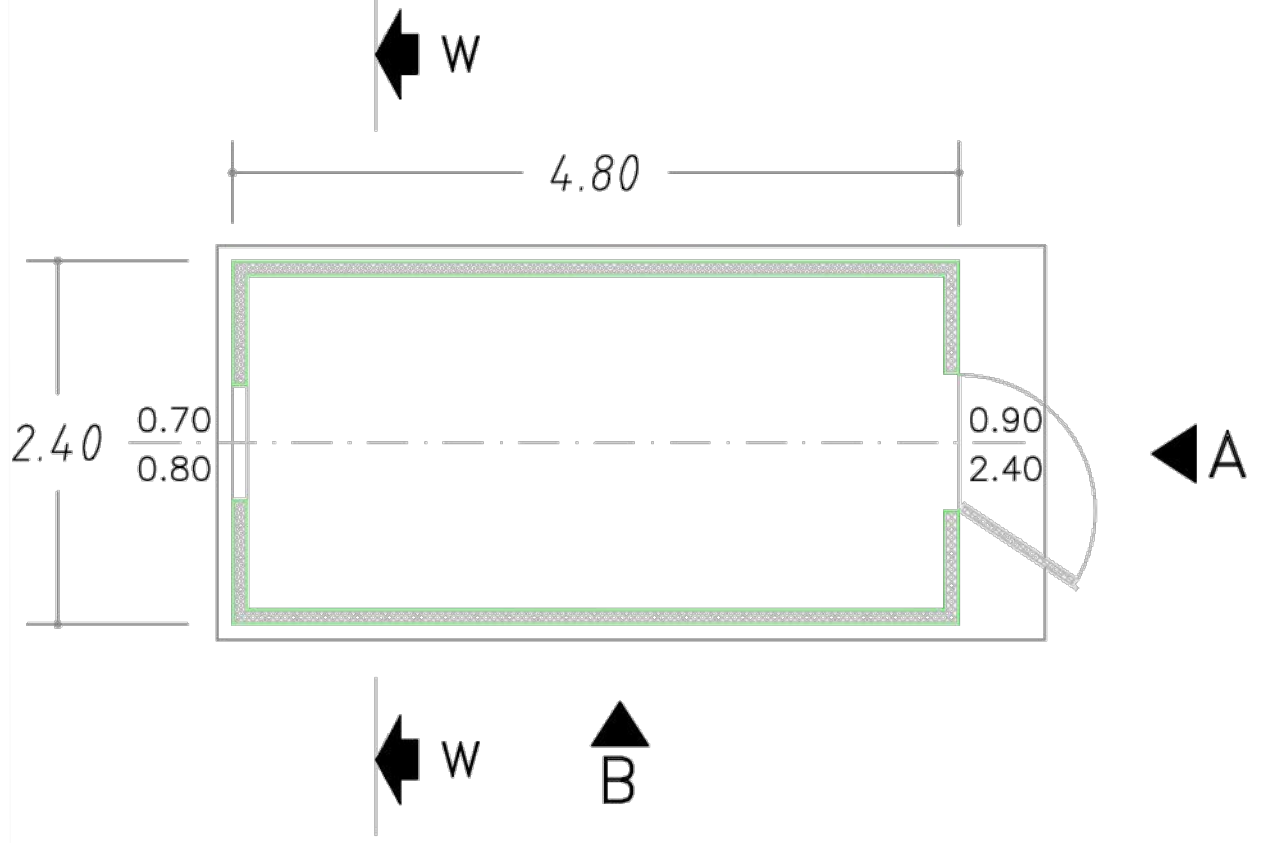
PIANTA
