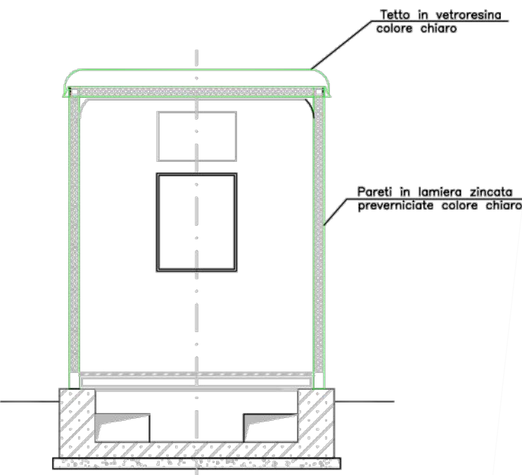
SEZIONE W-W
