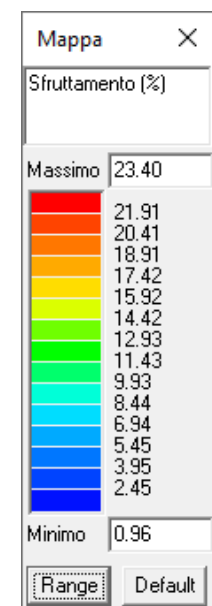
Sfruttamenti condizione D
