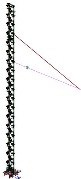
Carichi dovuti al vento longitudinale (Y)
