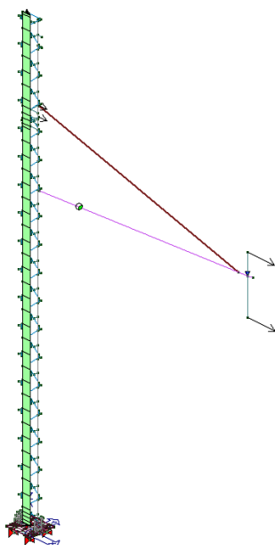
Carichi dovuti al vento trasversale (X)
