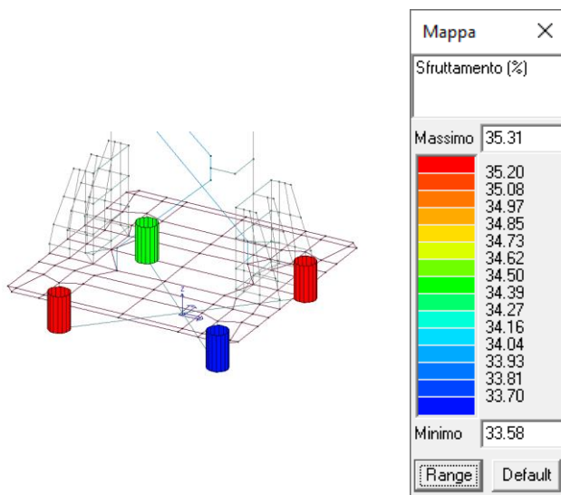
Sfruttamenti condizione B
