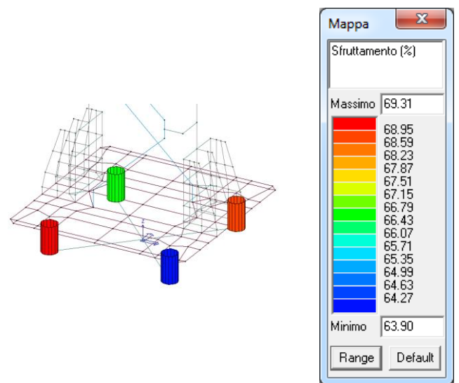
Sfruttamenti condizione D
