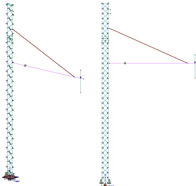
Modellazione del palo picc. 108 agli elementi finiti
