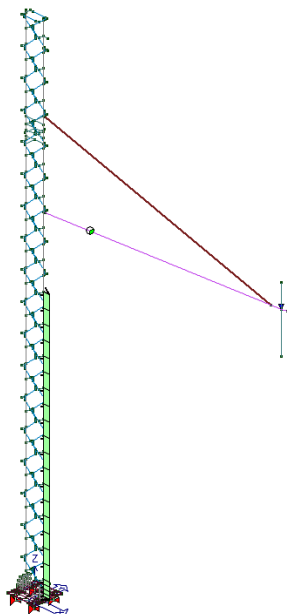
Carichi dovuti al vento trasversale aerodinamico (X)
