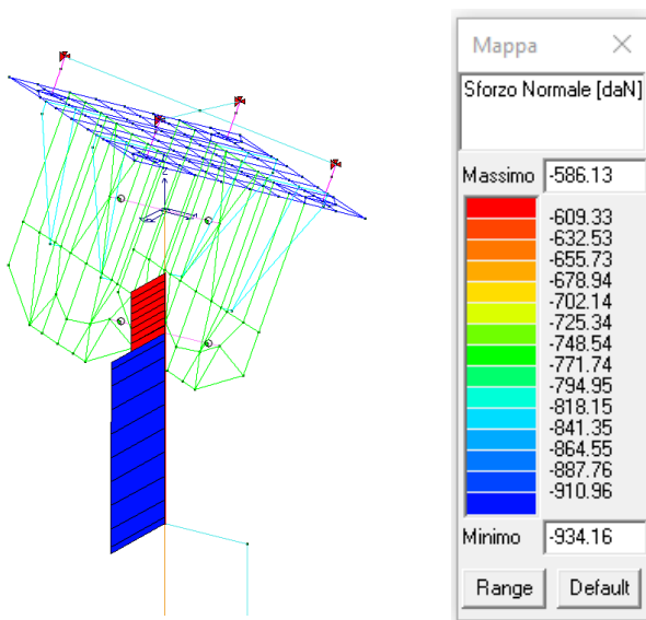
Combinazioni statiche
