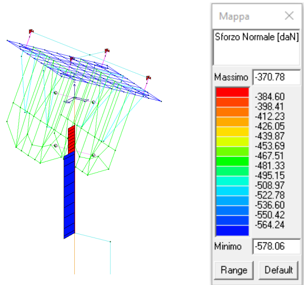
Combinazioni sismiche
