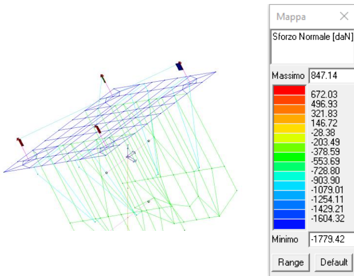
Combinazioni statiche
