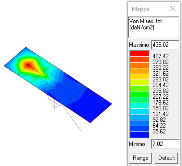
Combinazioni sismiche
