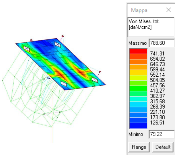
Combinazioni statiche
