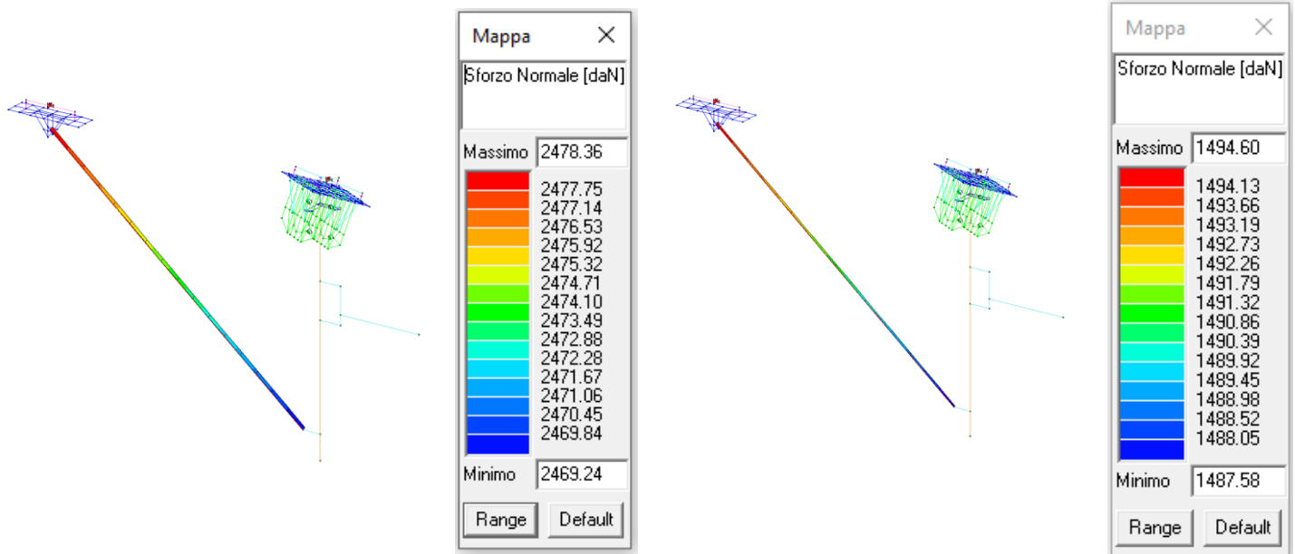
Combinazioni statiche
