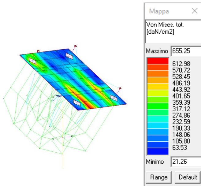
Combinazioni sismiche
