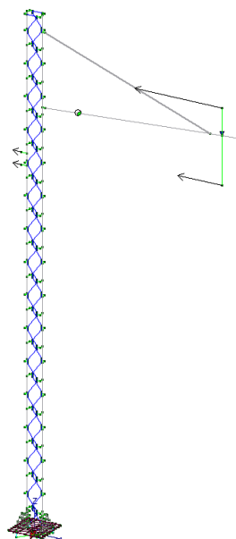
Carichi dovuti al tiro dei conduttori
