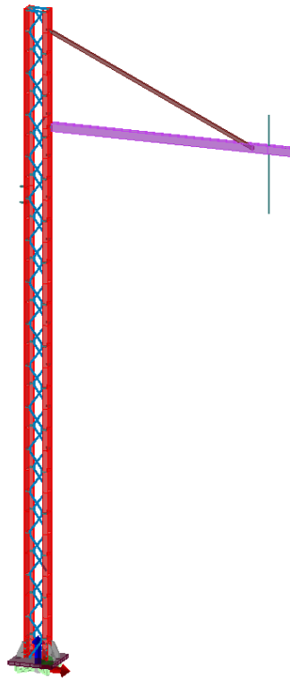
Modellazione del palo picc. 232 agli elementi finiti
