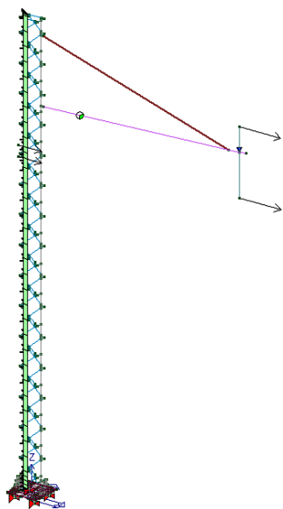
Carichi dovuti al vento trasversale (X)
