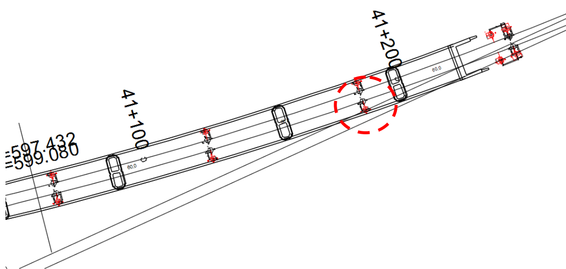
Figura 1 Stralcio planimetrico
