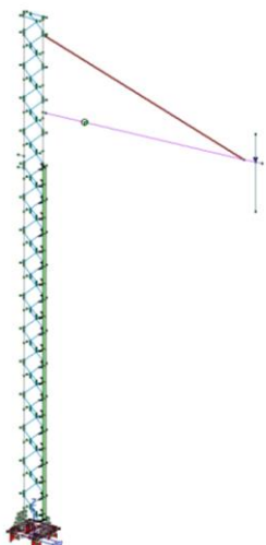
Carichi dovuti al vento trasversale aerodinamico (X)
