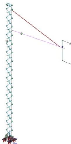
Carichi dovuti al tiro dei conduttori
