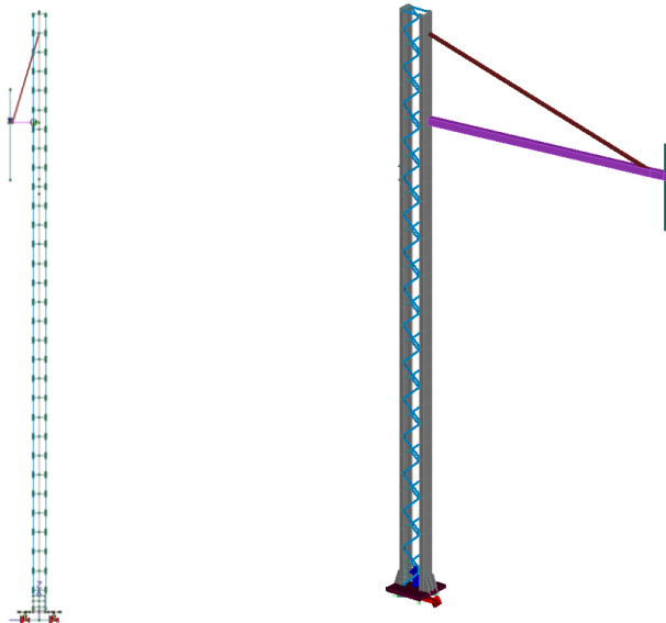
Modellazione del palo picc. 84 agli elementi finiti
