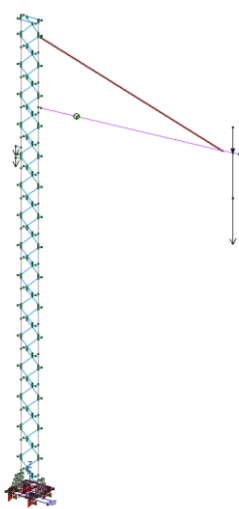
Carichi dovuti al peso dei conduttori
