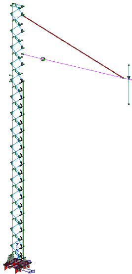
Carichi dovuti al vento trasversale aerodinamico (X)
